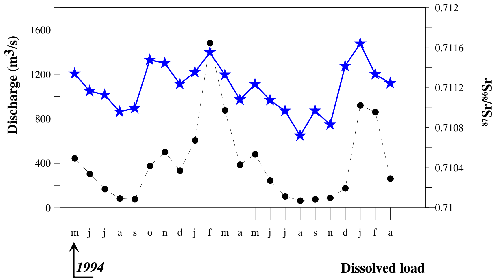
Figure 3. Fluctuations des rapports ^{87}\text{Sr}/^{86}\text{Sr} dans la fraction dissoute (★) en fonction du débit de la Loire (☞) selon les mois depuis le début de la période de prélèvements en Mai 1994, figure extraite de Grosbois et al. (2000, Chemical Geology 170, 179-201).
