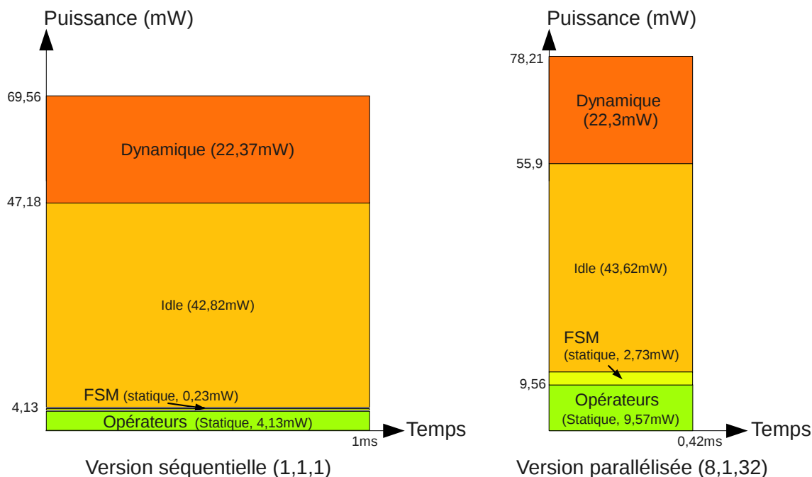
FIGURE 2.9: Représentation de la puissance consommée par deux versions accélératrices matérielles de la multiplication matricielle. Les échelles sont respectées entre les deux schémas.
