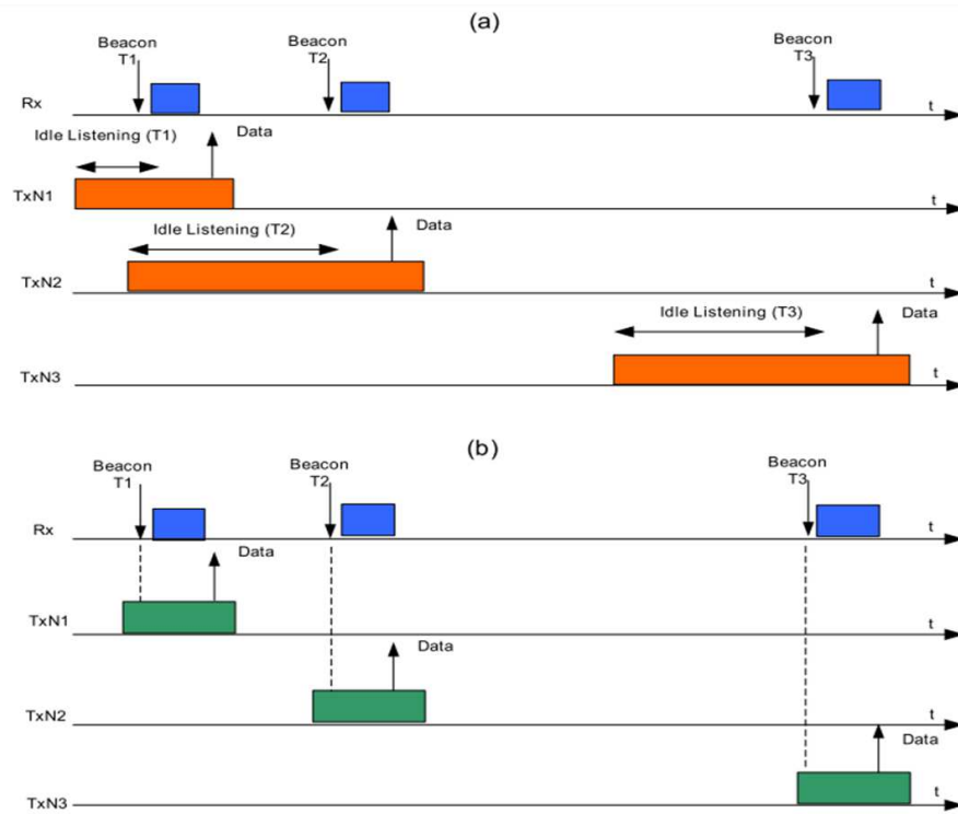
FIGURE 11: Adaptation de l'intervalle de réveil aux messages des différents capteurs
