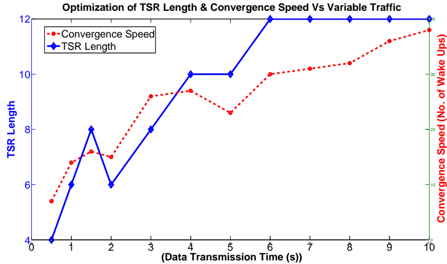
FIGURE 14: Optimisation de la longueur du TSR et vitesse de convergence associée en fonction du trafic (de 2 paquets par seconde à 1 paquet toutes les 10 secondes).
