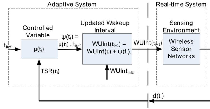
FIGURE 13: Vue d'ensemble du système adaptatif.
