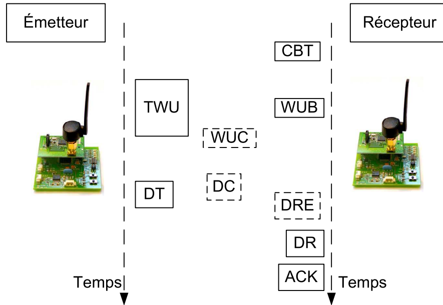
FIGURE 8: Phases de communication entre émetteurs et récepteurs. Le modèle d'énergie est basé sur les traces d'exécution des différents scénarios possibles durant la communication.
