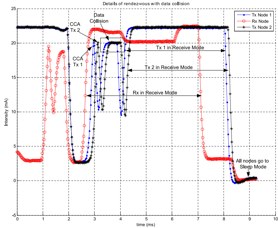
FIGURE 7: Communication ratée pour cause de collision de données entre les deux émetteurs.
