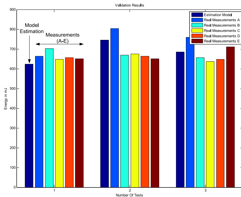
FIGURE 10: Comparaison de notre modèle d'énergie avec différentes sessions de mesures pour 3 tests de 300s avec des valeurs différentes pour TWU et WUInt .
