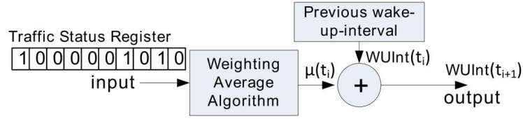
FIGURE 12: Algorithme de mise à jour de l'intervalle de réveil. TSR désigne le registre de statut du trafic, dans lequel '1' veut dire que le nœud a reçu un paquet qui lui était destiné, tandis que '0' révèle un réveil inutile.
