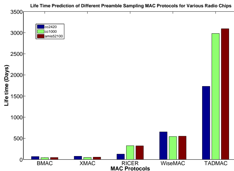
FIGURE 15: Durée de vie d'un nœud (batterie alcaline AA) pour différents protocoles MAC et transceivers radio. Les transceivers amis52100 et cc1000 sont préférables pour de faibles trafics tandis que le cc2420 convient à des trafics plus élevés. Le protocole TAD-MAC apporte dans tous les cas un gain important.
