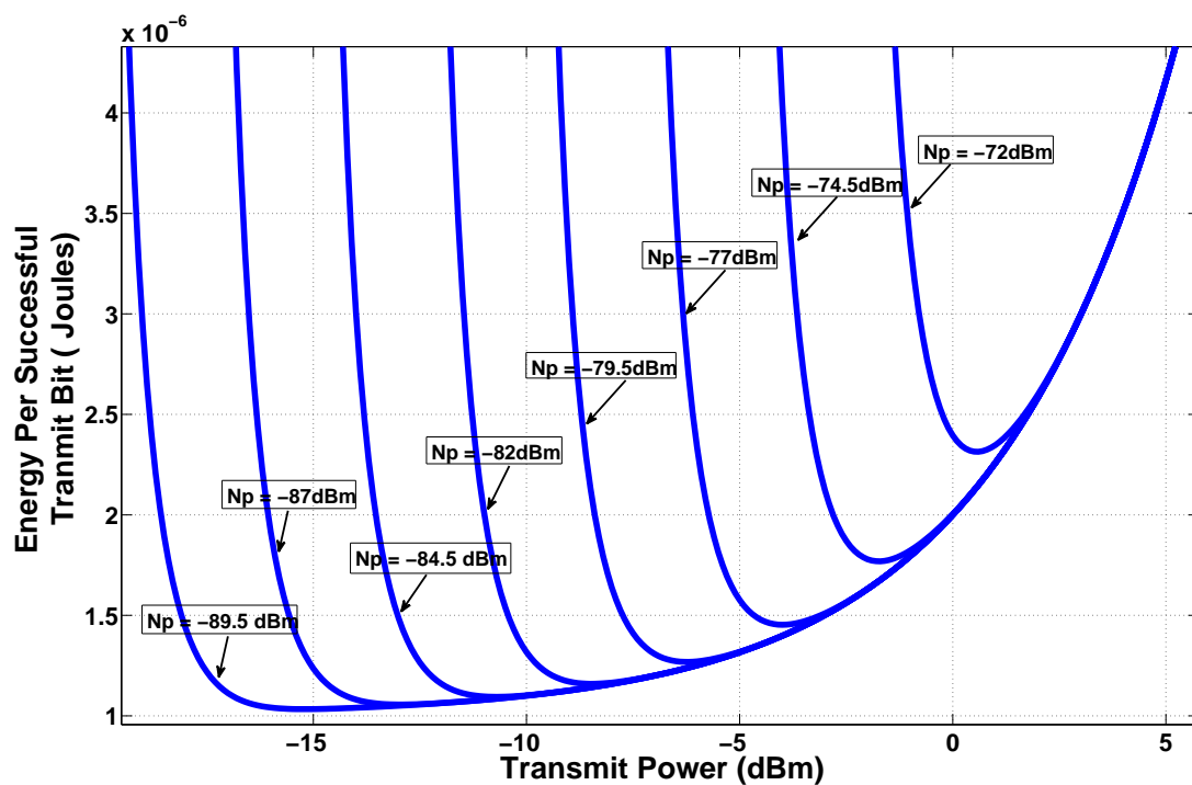
FIGURE 16: Energie consommée par bit transmis avec succès pour différents niveaux de bruit N_p .
