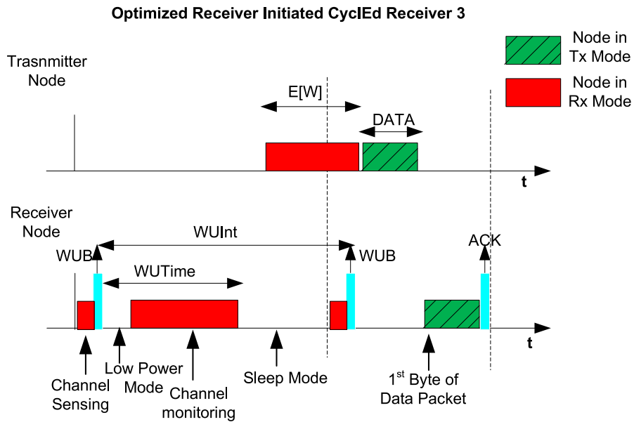
FIGURE 6: Protocole RICER optimisé ajustable à l'application et diminution de l'écoute inutile.
