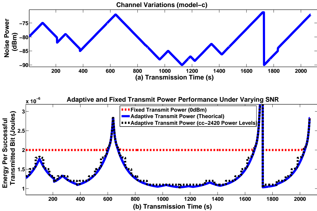
FIGURE 17: (a): Variations temporelles du canal (b): energie dépensée correspondante.
