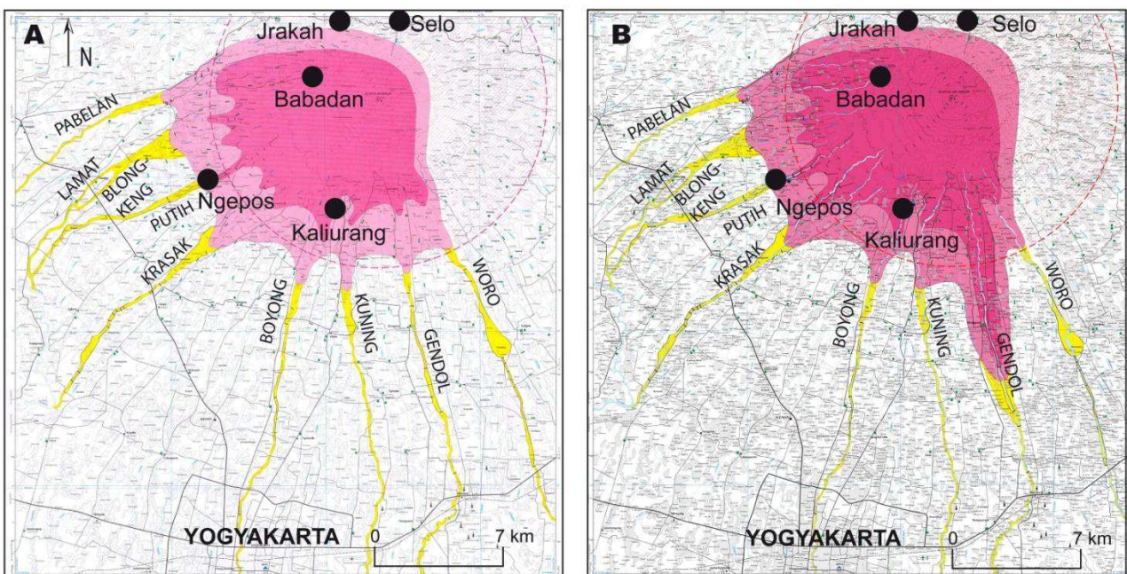
Figure 12 – Exemples de l’évolution de la « cartes des risques » publiées par le PVMBG (A : 2002 ; B : 2011). Rose vif : zone d’exposition maximale aux aléas éruptifs (flux pyroclastiques notamment, émissions gazeuses, projections), évacuations prioritaires. Rose pâle : zone susceptible d’être touchée par les aléas éruptifs en cas d’éruption centennale, évacuations en fonction de l’intensité de l’éruption. Jaune : rivières dans lesquelles peuvent se produire des lahars. Cercle en pointillés rouges : extension possible des projections de téphras de diamètre > 2 mm. En points noirs : les observatoires du volcan. Remarquer le prolongement des zones d’exposition aux aléas éruptifs le long de la Gendol, suite à l’éruption de 2010.
