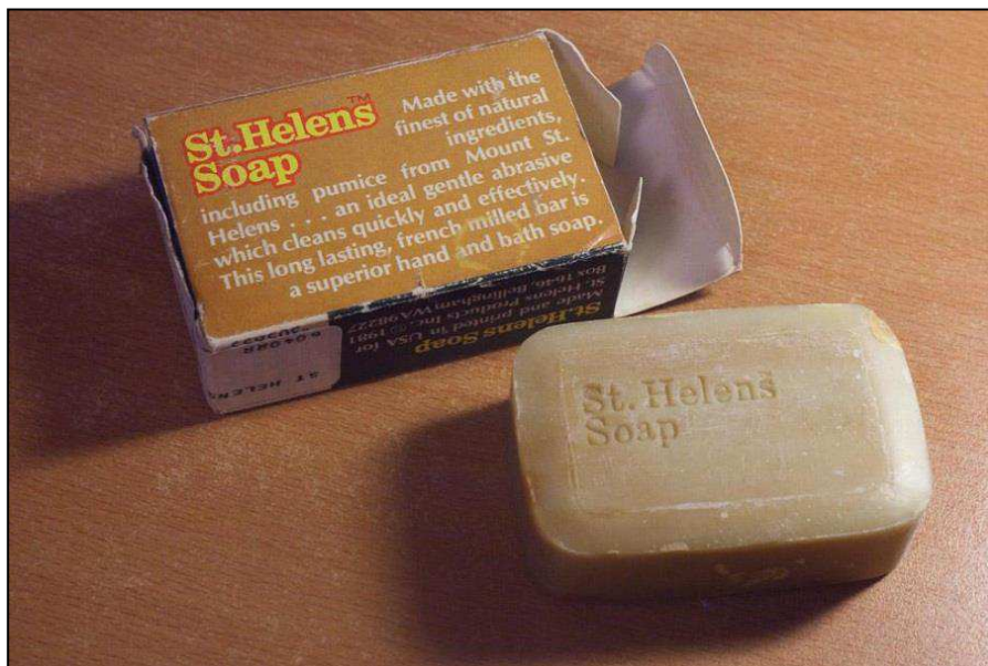
Figure 16 – Savon auquel des cendres ponceuses du St Helens ont été incorporées ( http://greg-willis.com/2010.05.18/mount-st-helens-soap )
