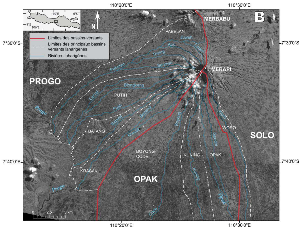
Figure 3 – Bassins-versants du Merapi. A : modèle numérique de terrain ASTER GDEM ; B : image Spot 5 (2008) ; seules les principales rivières sont figurées
