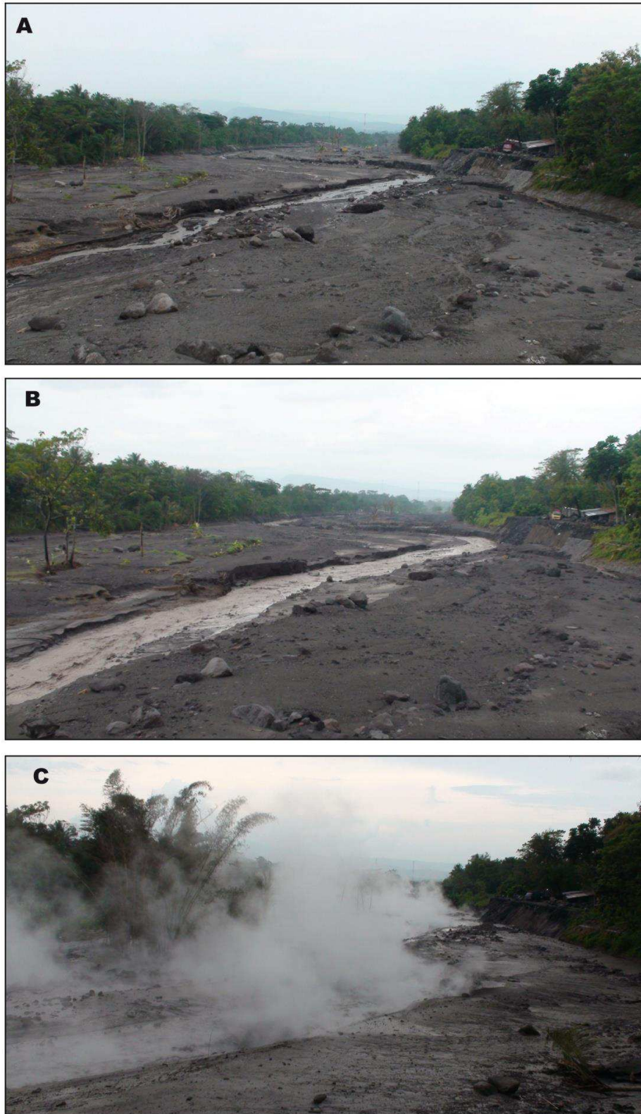
Figure 117 – La rivière Gendol, différences entre : A mode d'écoulement fluviatile et lent de faible profondeur, incision des dépôts du large corridor de lahar. B : « banjir », écoulement torrentiel plus profond et rapide, augmentation du débit mais pas de débordement sur le corridor de lahar. C : lahar, écoulement non chenalisé sur l'ensemble du corridor, transport de matériel grossier (repérer les blocs à gauche de l'image et les débordements latéraux sur la rive droite du chenal). La haute température du lahar est indiquée par le panache de vapeur qu'il dégage.
