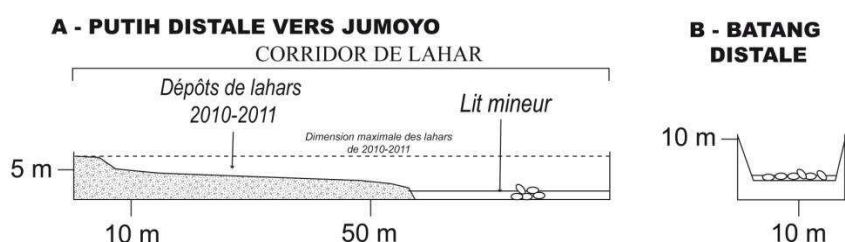
Figure 50 - Profils comparés de la Putih (A) et de la Batang (B) au niveau de Muntilan Les lahars de la Putih peuvent atteindre des largeurs maximales de près de 90 m pour des profondeurs de plus de 5 m. Avec des dimensions réduites, la Batang n'est plus calibrée pour supporter le passage d'un éventuel lahar de grande intensité. La seule occurrence de lahar survenue dans la Batang après l'éruption de 2010 n'a laissé que de maigres dépôts dans le lit de la rivière. Une défluviation d'un lahar énergique depuis la Putih vers la Batang provoquerait inmanquablement de très importants réajustements du réseau hydrographique qui menacent les habitations riveraines de cette rivière, regroupant près de 3000 personnes (recensement de 2010).
