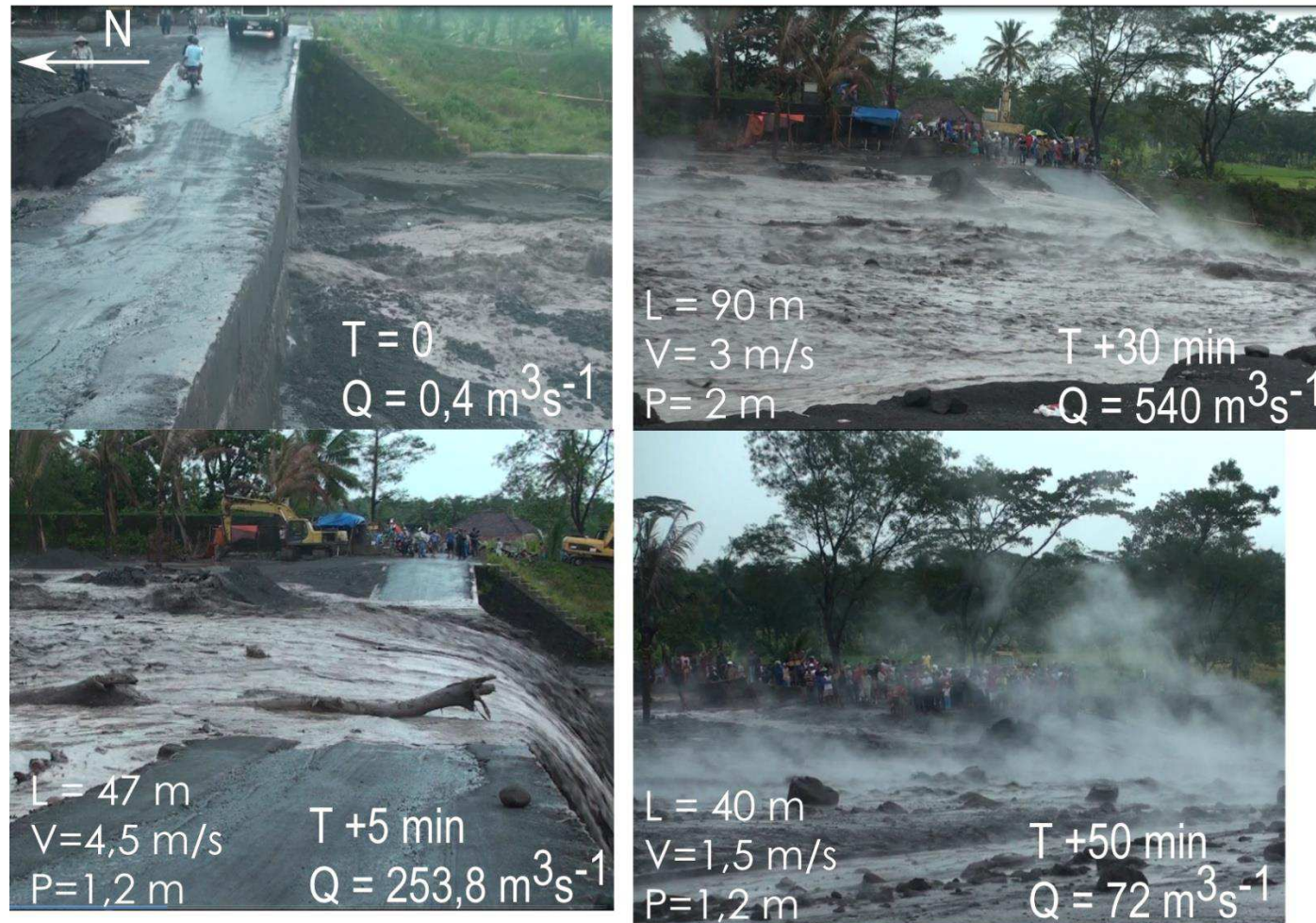
Figure 34 - Prises de vue des lahars de la Gendol filmés à Plumbon (L = Largeur ; V = Vitesse de surface ; P = Profondeur) A : Lahar du 28 février 2011 (le pont des deux premières photos est visible sur la partie droite des deux dernières photos)
