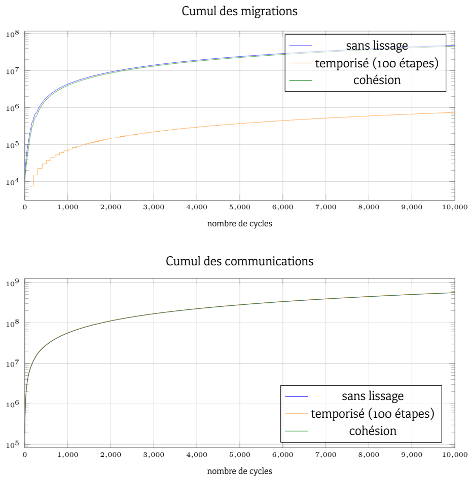
FIGURE 10.13 : Évolution du nombre total de communications effectives et de migrations pour la simulation \mathcal{S}_2 (échelle logarithmique)
