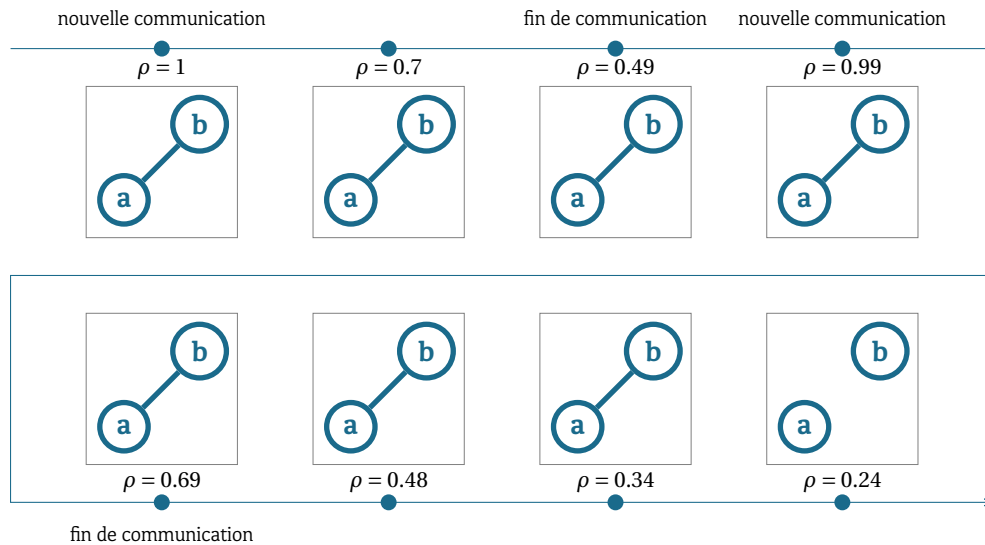
FIGURE 6.4 : Création d'interactions avancée avec \rho_{init} = 1 , \delta_\rho = 0.5 , \omega = 0.7 et \rho_{del} = 0.3 .
