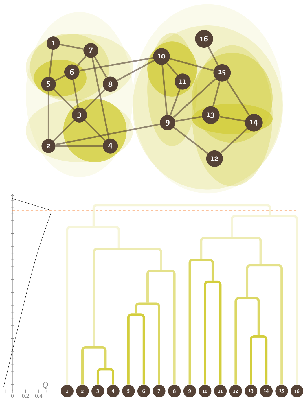
FIGURE 4.3 : Dendrogramme associé à une classification hiérarchique ascendante. La courbe de gauche représente l'évolution de la qualité Q au fur et à mesure des fusions. On observe que la qualité maximale est atteinte à l'avant dernière fusion, ce qui nous donne une bissection du graphe.
