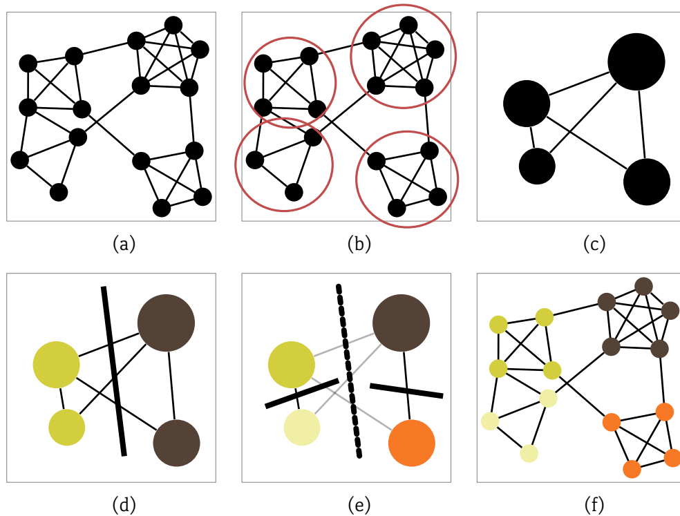
FIGURE 4.2 : Illustration de l'approche multi-niveaux appliquée au partitionnement. (a) présente le graphe initial, dans lequel on détermine un regroupement des nœuds en (b). Puis en (c) les nœuds des groupes sont fusionnés afin de créer un graphe d'un plus haut niveau. (d) et (e) montrent le calcul d'une partition par bisection. Le graphe est reconstruit en (f).
