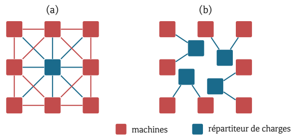
FIGURE 10.1 : Différents scénarios d'utilisation du répartiteur de charges : (a) une machine dédiée, (b) un ensemble de machines dédiées, (c) chaque machine participe à la répartition
