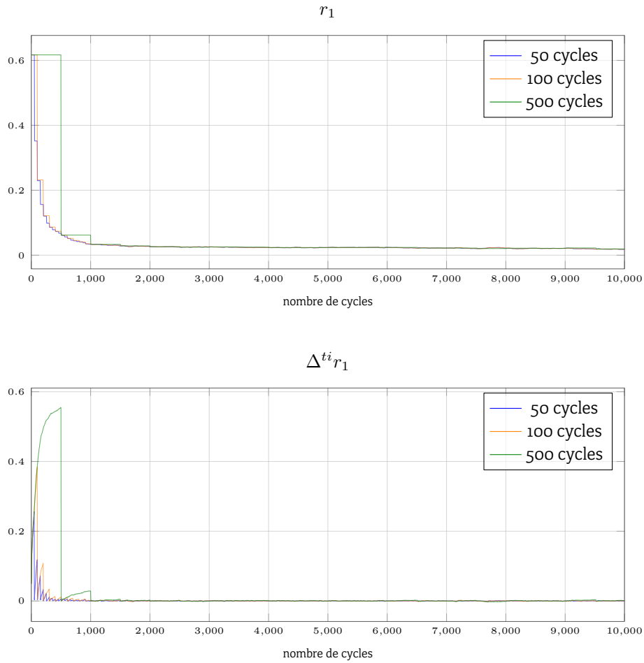
FIGURE 10.6 : Impact de la valeur du délai sur l'évolution de r_1 pour la simulation \mathcal{S}_1 .
