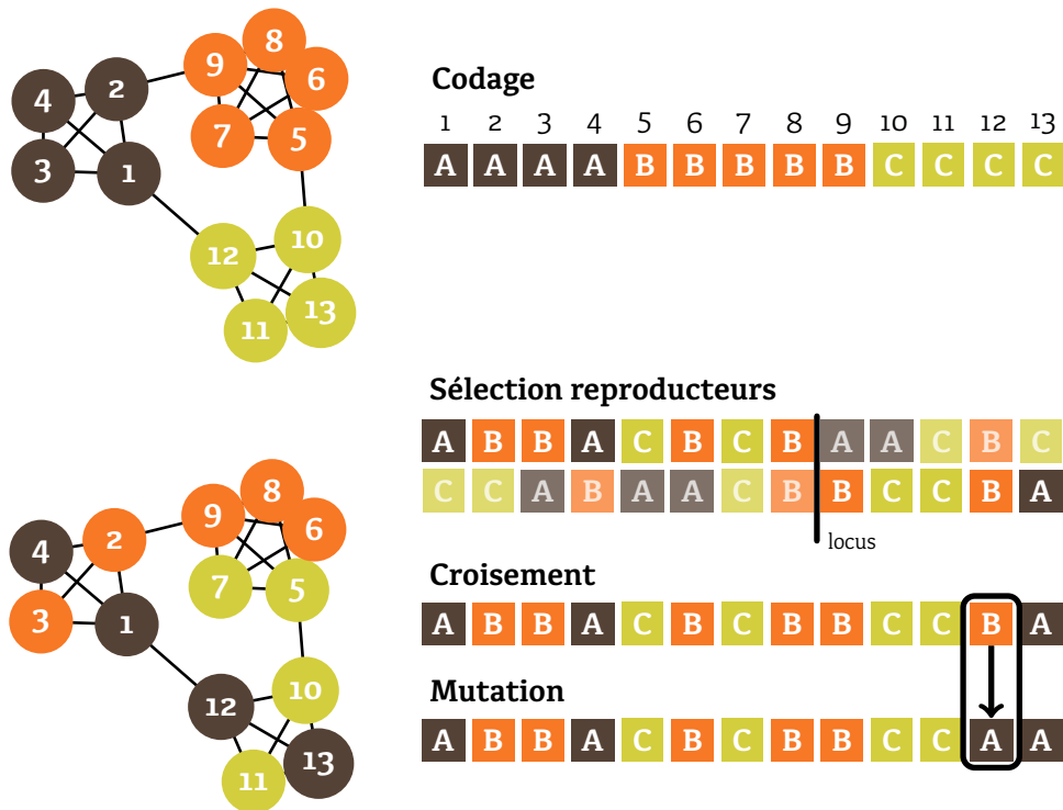
FIGURE 4.5 : Codage, croisement et mutation dans un algorithme génétique. On considère pour le codage que les nœuds peuvent être de numérotés de 1 à n , le code est alors une chaîne de caractères où le i^{\text{ème}} caractère représente la classe du nœud i . Le croisement permet de combiner les codes de deux individus, et la mutation d’ajouter de l’aléatoire.
