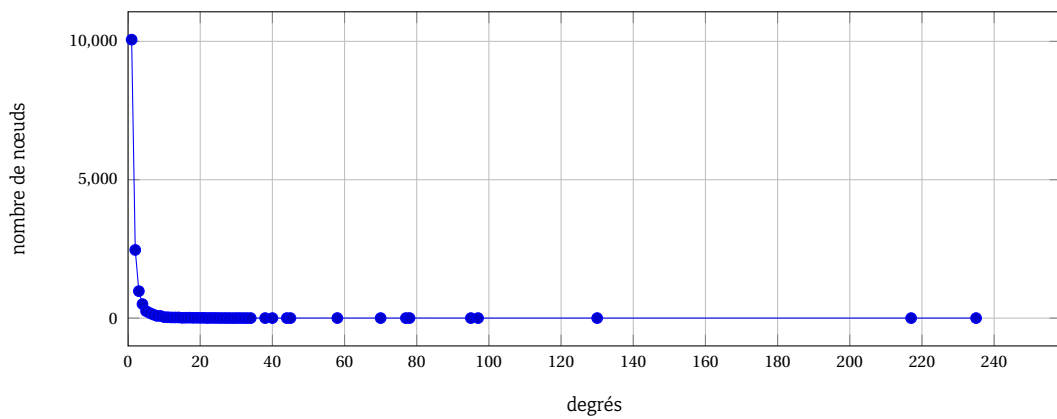
34 FIGURE 3.2 : Réseau sans-échelle généré avec GRAPHSTREAM par attachement préférentiel.
