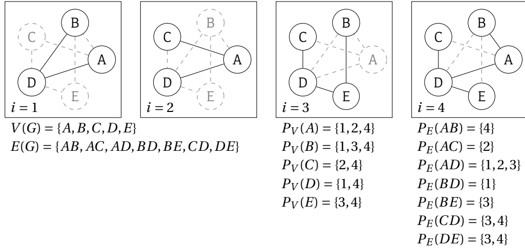
FIGURE 3.5 : Illustration du modèle de dynamique cumulative. Les éléments en pointillés ne sont pas présents dans le graphe pour le temps donné.
