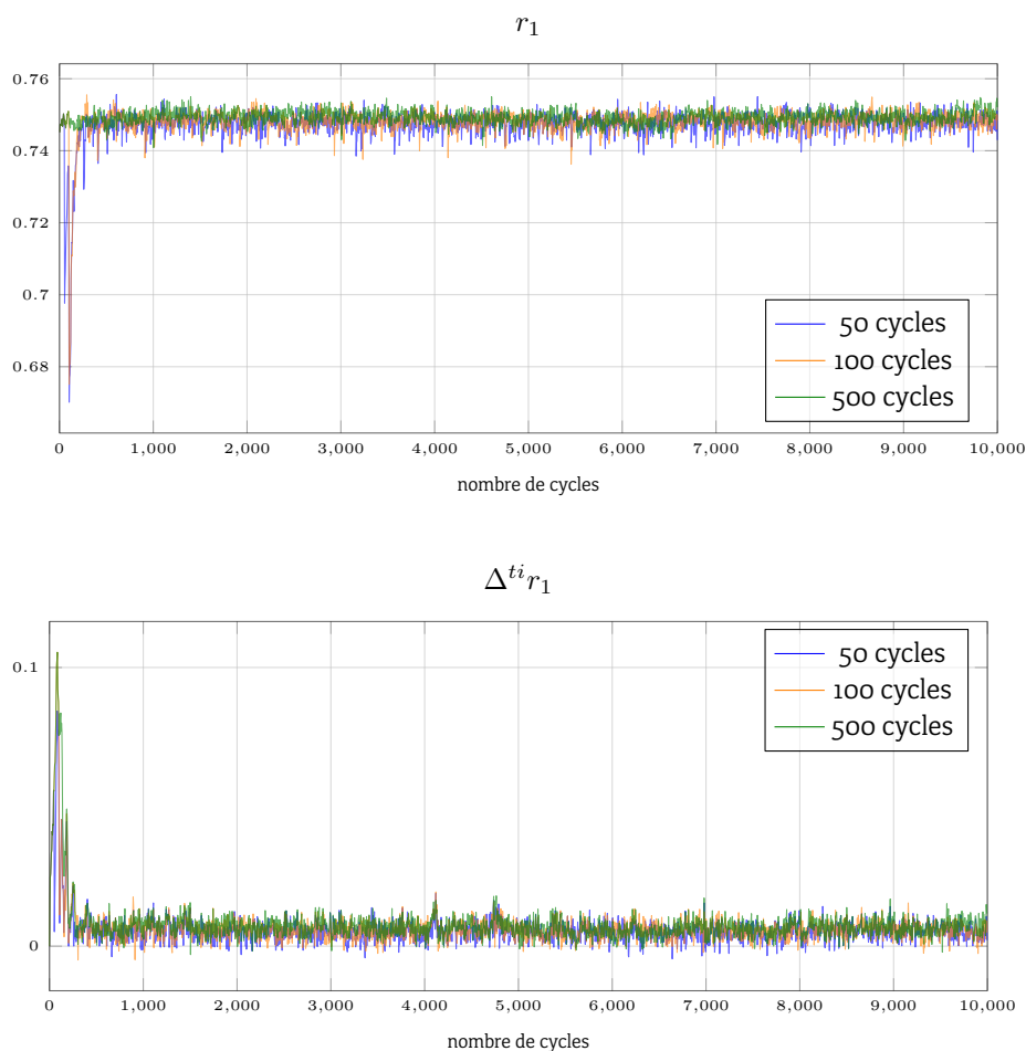
FIGURE 10.8 : Impact de la valeur du délai sur l'évolution de r_1 pour la simulation S_2 .
