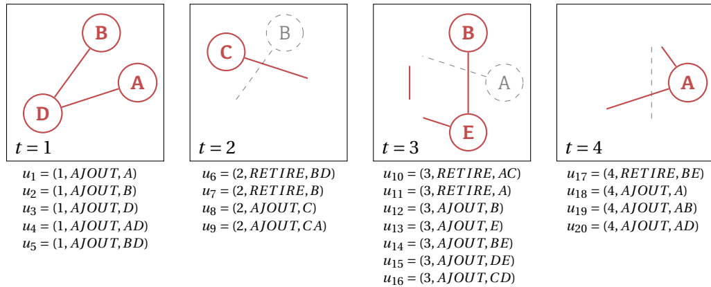
FIGURE 3.6 : Illustration du modèle de dynamique en flux. Les éléments rouges viennent d'être ajoutés dans le graphe, tandis que les éléments en pointillés ont été supprimés.
