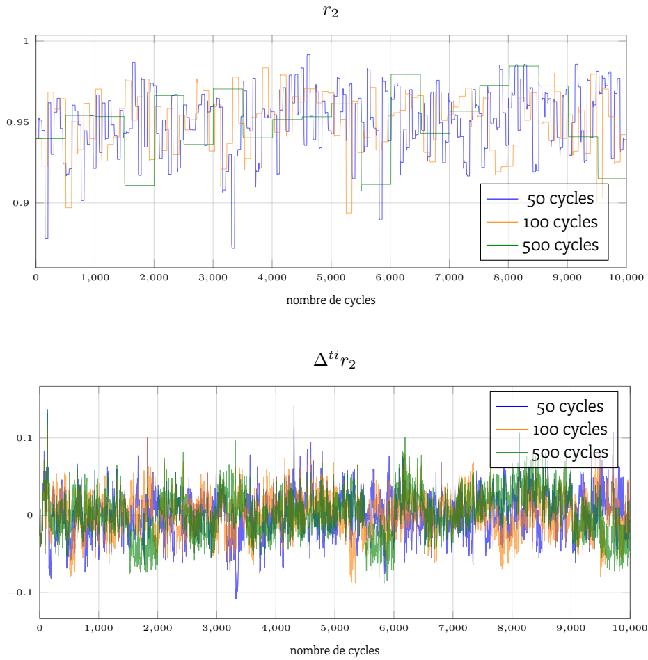
FIGURE 10.9 : Impact de la valeur du délai sur l'évolution de r_2 pour la simulation S_2 .
