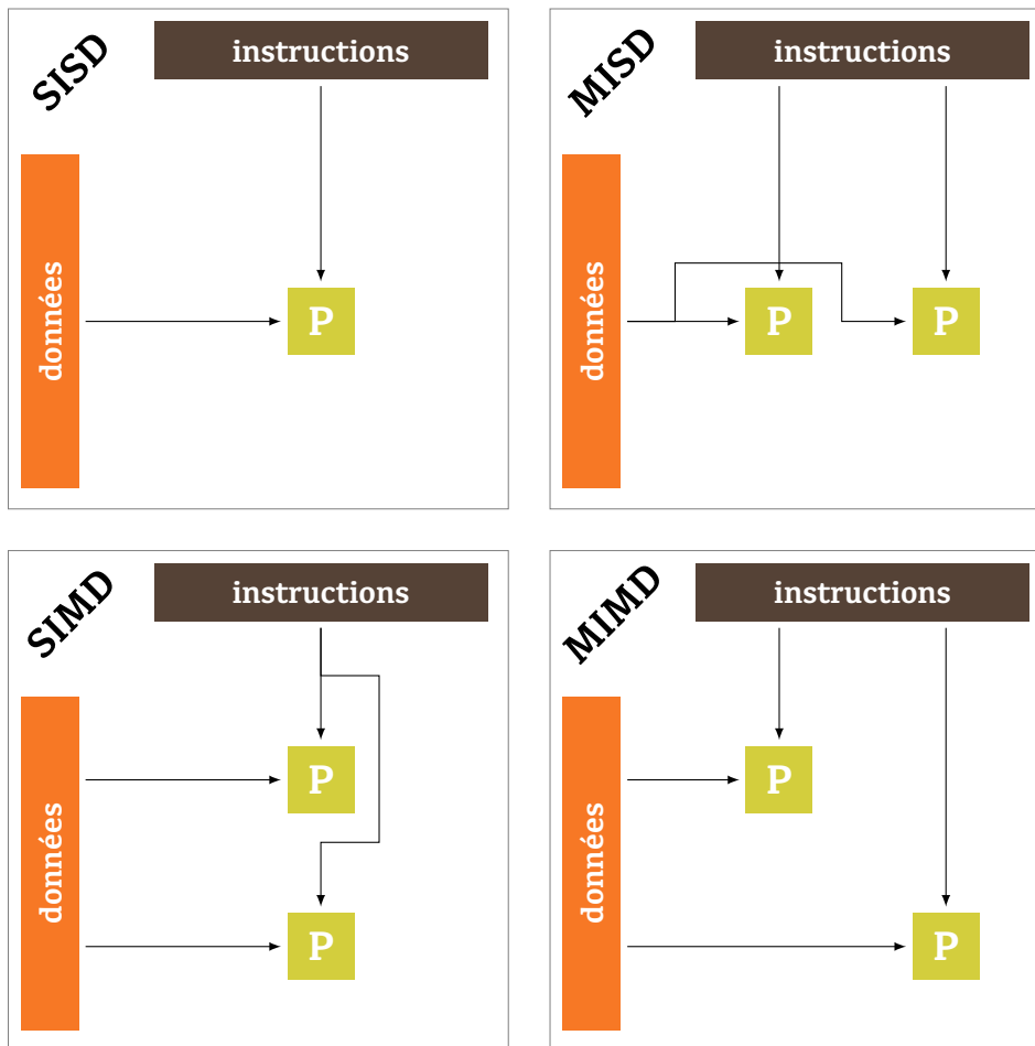
FIGURE 5.1 : Classification de l'architecture des machines proposée par Michael J. FLYNN. Les processeurs sont représentés par P .
