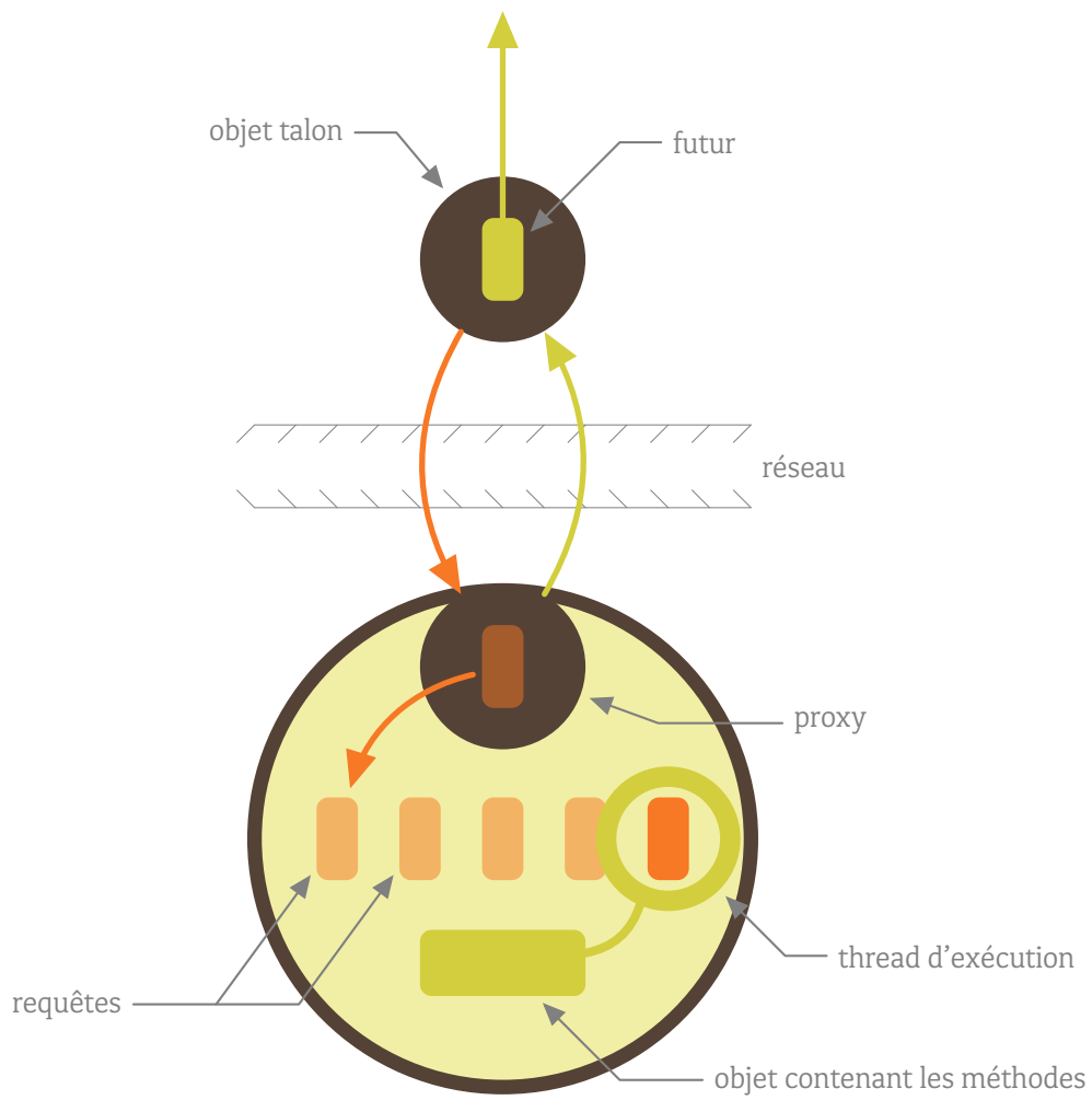
FIGURE 11.2 : Architecture d'un acteur.
