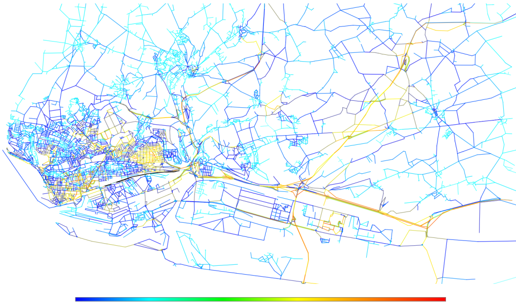
FIGURE 9.8 : Le réseau routier du Havre et de ses environs modélisé en tant que graphe par GRAPHSTREAM. On applique sur ce graphe une marche aléatoire « temporisée » c'est à dire que les entités qui l'utilisent vont à la vitesse maximale autorisée sur les arcs. Les entités possèdent, de plus, une mémoire des arcs traversés (la taille de la mémoire est fixée à 40 pour cet exemple) qui agit comme une liste d'arcs tabous qui ne peuvent être utilisés qu'en dernier recours.
