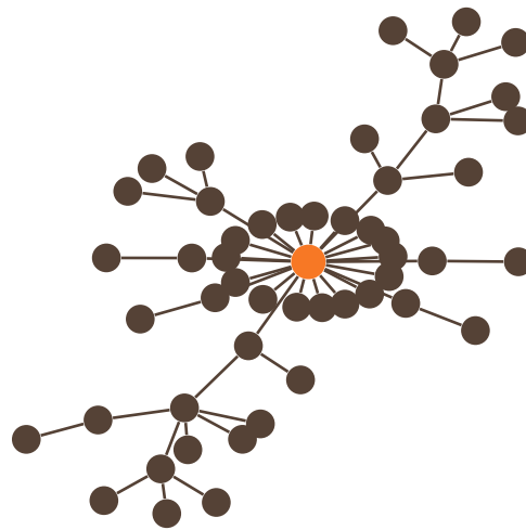
FIGURE 8.4 : Dans cet arbre de 50 nœuds, les fourmis ont détecté le centroïde optimal (représenté en orange sur la figure), c'est à dire le même centroïde que celui calculé par l'algorithme classique
