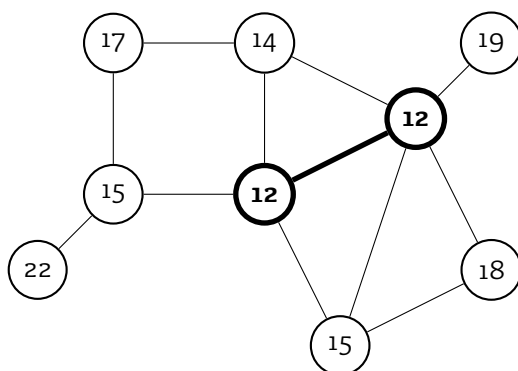
FIGURE 8.1 : Distances des nœuds. La structure en gras représente le sous-graphe induit par les nœuds dont la distance est minimale, ce qui correspond au centroïde de ce graphe.
