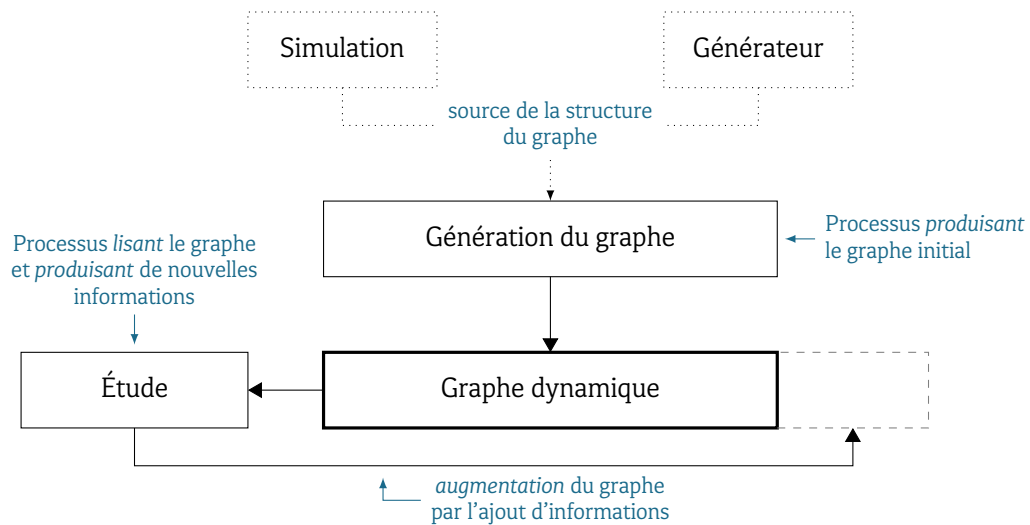
FIGURE 3.14 : Concept de processus. Un processus initial est utilisé pour générer le graphe. Un autre processus est utilisé pour analyser le graphe et l'augmenter grâce aux informations calculées.
