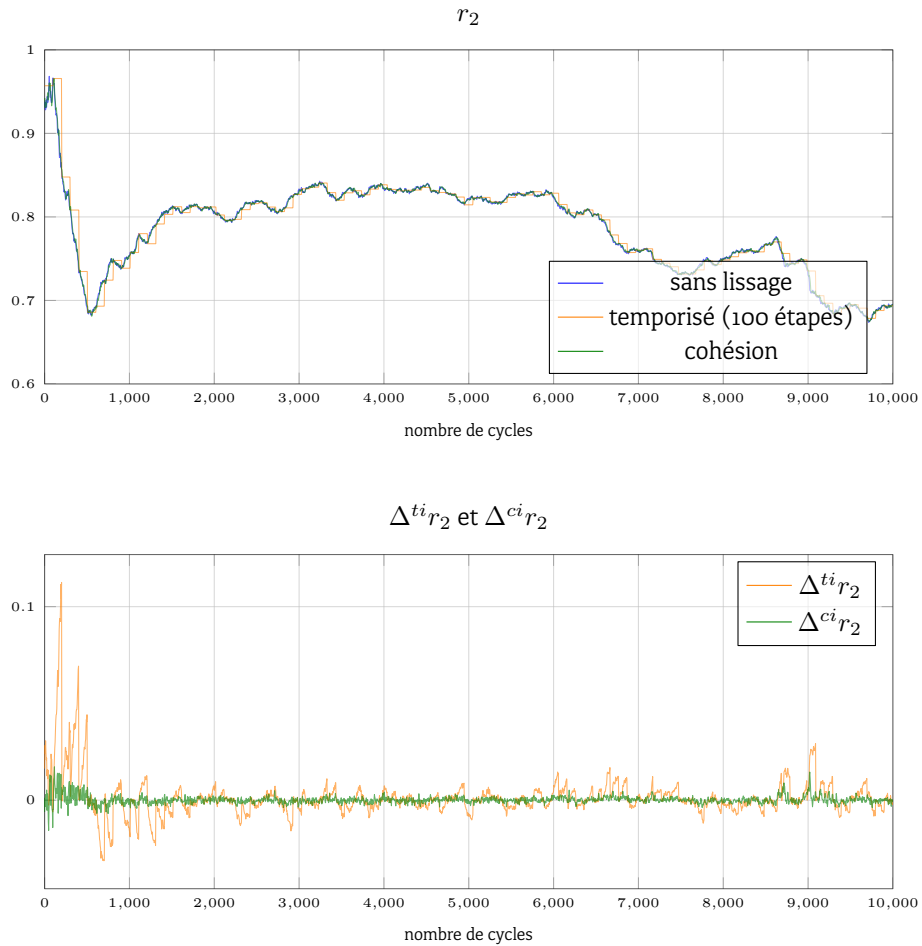
FIGURE 10.5 : Tracé de la mesure r_2 pour la simulation \mathcal{S}_1 . La différence moyenne entre la mesure de r_2 pour le lissage temporisé et celle de la méthode sans lissage est 1.20 \cdot 10^{-3} avec un écart type de 1.05 \cdot 10^{-2} . Pour le lissage par cohésion, cette différence moyenne est de 1.72 \cdot 10^{-4} avec un écart type de 2.07 \cdot 10^{-3}
