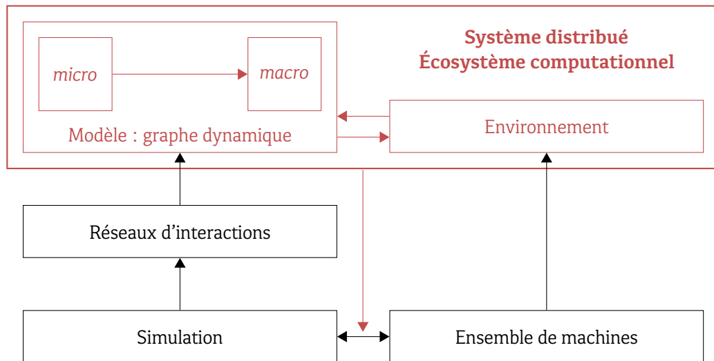
FIGURE 2.1 : Description du contexte. La partie colorée désigne ce à quoi nous nous intéressons c'est à dire d'une part le modèle d'un réseau d'interactions créé par une simulation et d'autre part un environnement de distribution modélisant les ressources disponibles.
