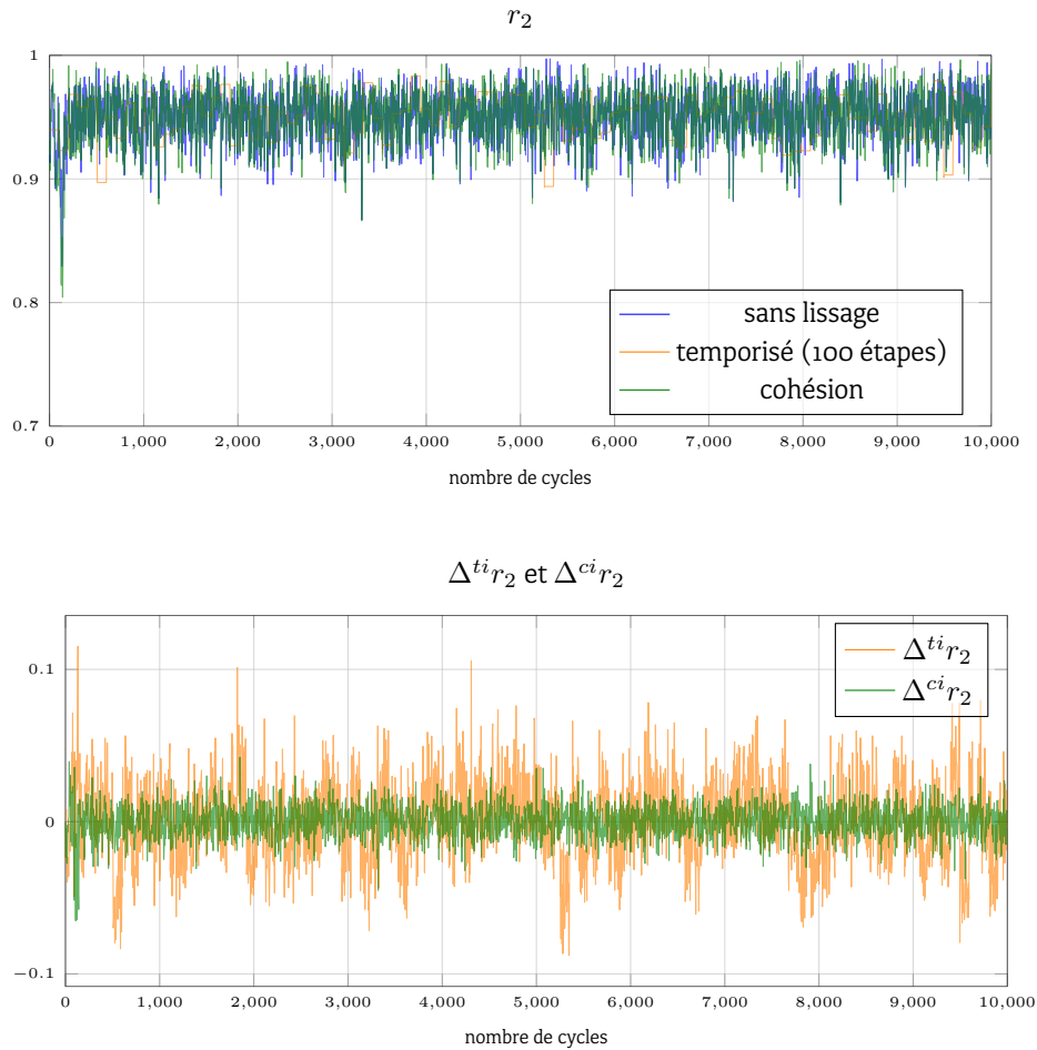
FIGURE 10.11 : Tracé de la mesure r_2 pour la simulation \mathcal{S}_2 . La différence moyenne entre la mesure de r_2 pour le lissage temporisé et celle de la méthode sans lissage est -5.21 \cdot 10^{-4} avec un écart type de 2.71 \cdot 10^{-2} . Pour le lissage par cohésion, cette différence moyenne est de -9.47 \cdot 10^{-5} avec un écart type de 1.08 \cdot 10^{-2}
