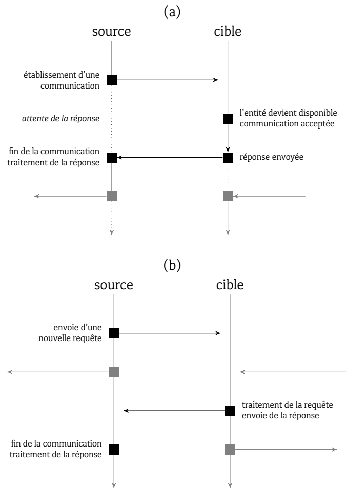
FIGURE 6.2 : Interaction (a) synchrone et (b) asynchrone entre une entité source et une entité cible.
