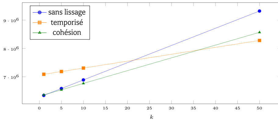
FIGURE 10.14 : Évolution de C en fonction de k pour la simulation S_1
