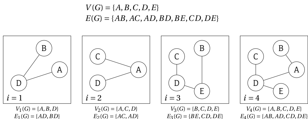
FIGURE 3.4 : Illustration du modèle de dynamique séquentielle
