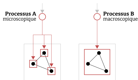
FIGURE 3.17 : Processus micro/macro.
