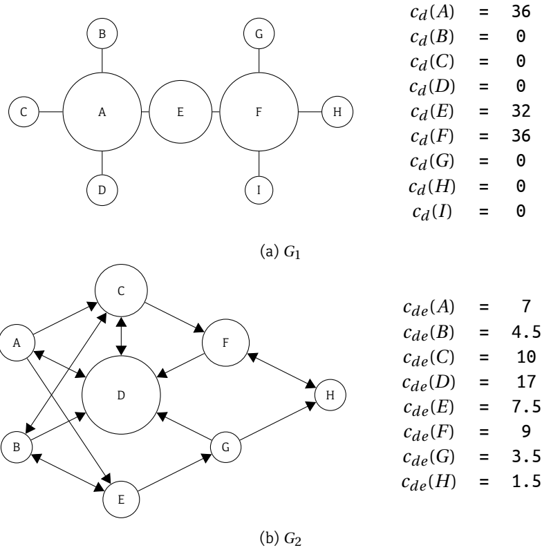
FIGURE 3.11 : Application de l'intermédierité aux graphes G_1 et G_2
