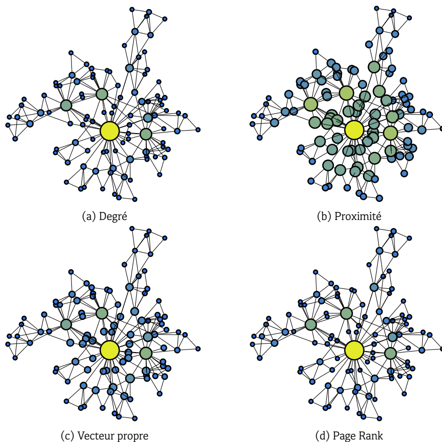
FIGURE 3.7 : Quelques exemples de mesure de la centralité. Plus la taille du nœud est importante (et plus sa couleur s’approche du jaune), plus la valeur de la centralité de ce nœud est importante.
