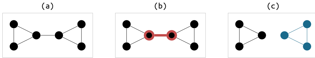
FIGURE 8.3 : (a) une organisation est fournie par un algorithme de détection d'organisations, (b) une partie faible est détectée, (c) l'organisation initiale est scindée en deux nouvelles organisations sans partie faible.
