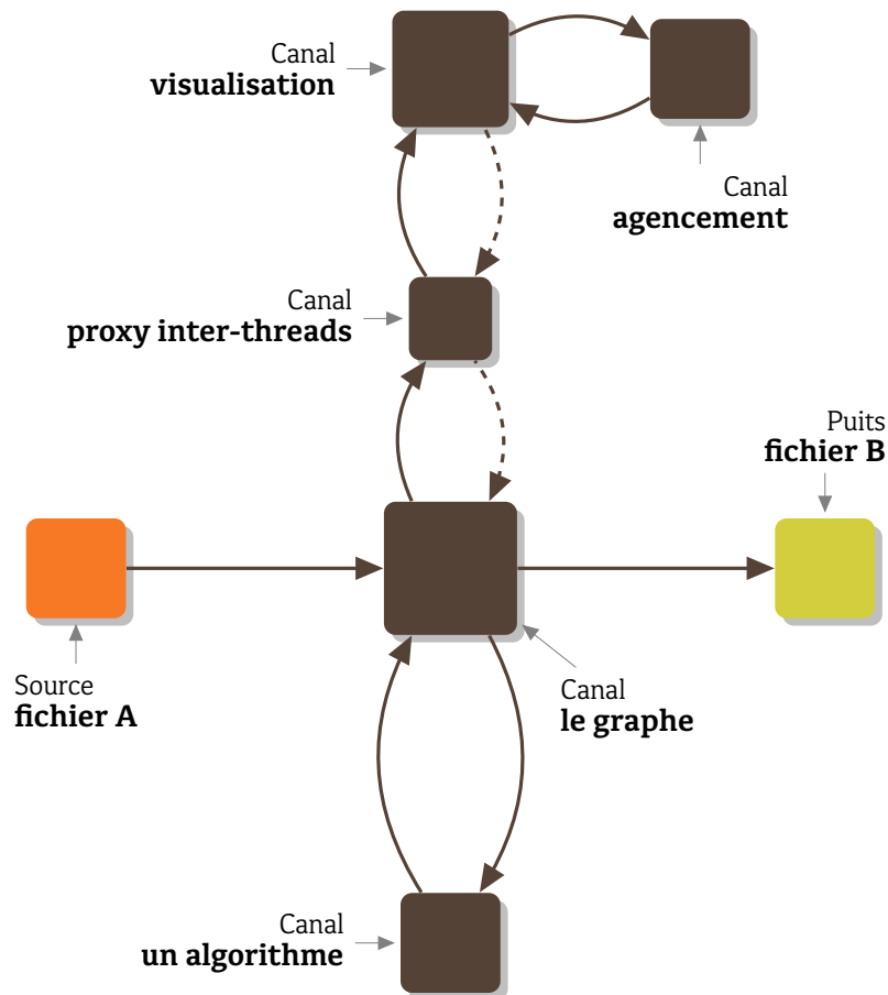
FIGURE 9.1 : Un exemple basique de réseau composé d'une source, de canaux, et d'un puits. Un fichier "A" est lu par une source afin de créer un graphe. On initialise une vue sur ce graphe dans un thread dédié aux graphismes. La vue communique avec le graphe au travers d'un proxy inter-threads. Elle utilise un algorithme d'agencement afin de positionner les nœuds. De plus, on exécute un algorithme sur le graphe qui répercute le fruit de son calcul directement dans le graphe. Enfin, le graphe, augmenté des données de l'algorithme, est stocké dans un fichier "B".
