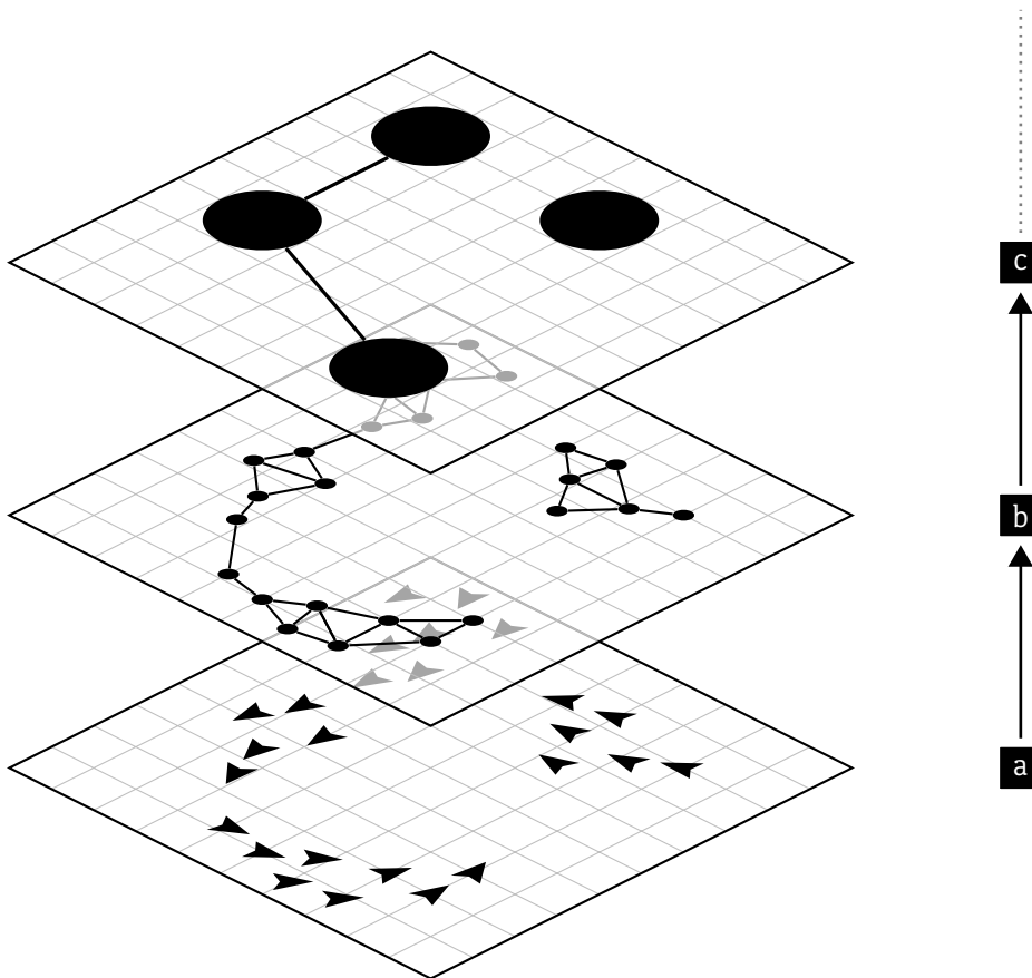
FIGURE 3.3 : Présentation des différentes couches en se basant sur une simulation de boïds : (a) le réseau d'interactions, (b) le graphe dynamique initial modélisant le réseau, (c) une vue macroscopique du graphe dynamique
