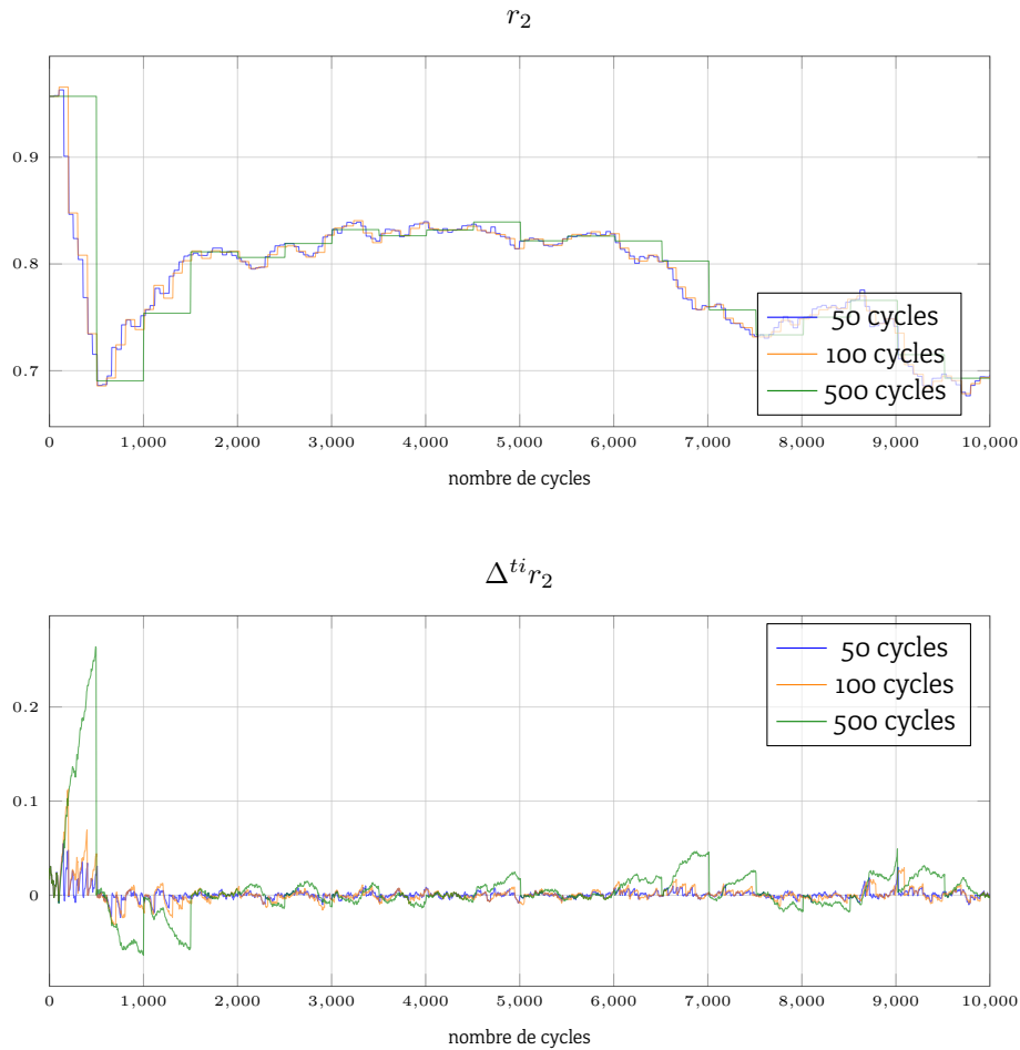
FIGURE 10.7 : Impact de la valeur du délai sur l'évolution de r_2 pour la simulation S_1 .
