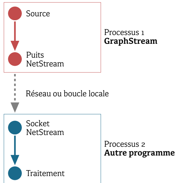
FIGURE 9.6 : Le protocole NetStream. Un programme GRAPHSTREAM est lancé dans lequel une source produit un graphe qui est envoyé à un puits NetStream. Un autre programme est lancé, éventuellement sur une machine différente. Ce programme inclut un socket qui se connecte au puits NetStream et qui va être capable d'interpréter le protocole et de traiter le graphe dynamique reçu.
