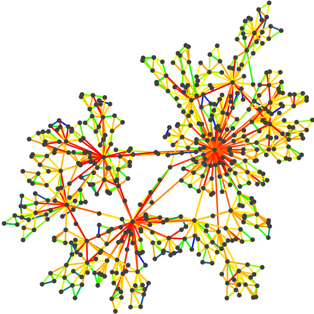
FIGURE 9.3 : Résultat d'une marche aléatoire sur un graphe généré à l'aide de l'algorithme de DOROGOVTSSEV-MENDES. Les couleurs indiquent la fréquence de passage des entités sur l'arête, plus la couleur tend vers la rouge, plus le passage est important. On peut interpréter ceci en terme de centralité : plus un nœud est connecté à des arêtes dont la fréquence est forte, plus sa centralité est élevée.
