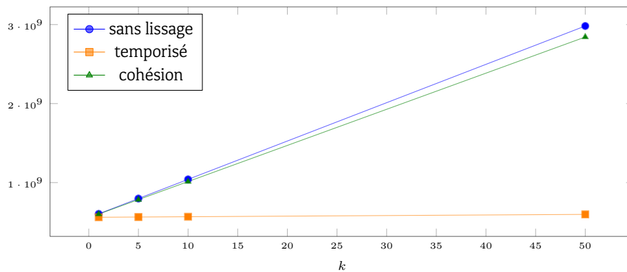
FIGURE 10.15 : Évolution de C en fonction de k pour la simulation S_2
