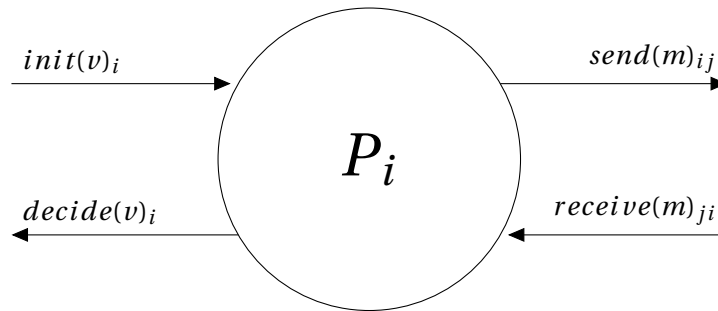
FIGURE 5.4 : Un automate e/s de processus
