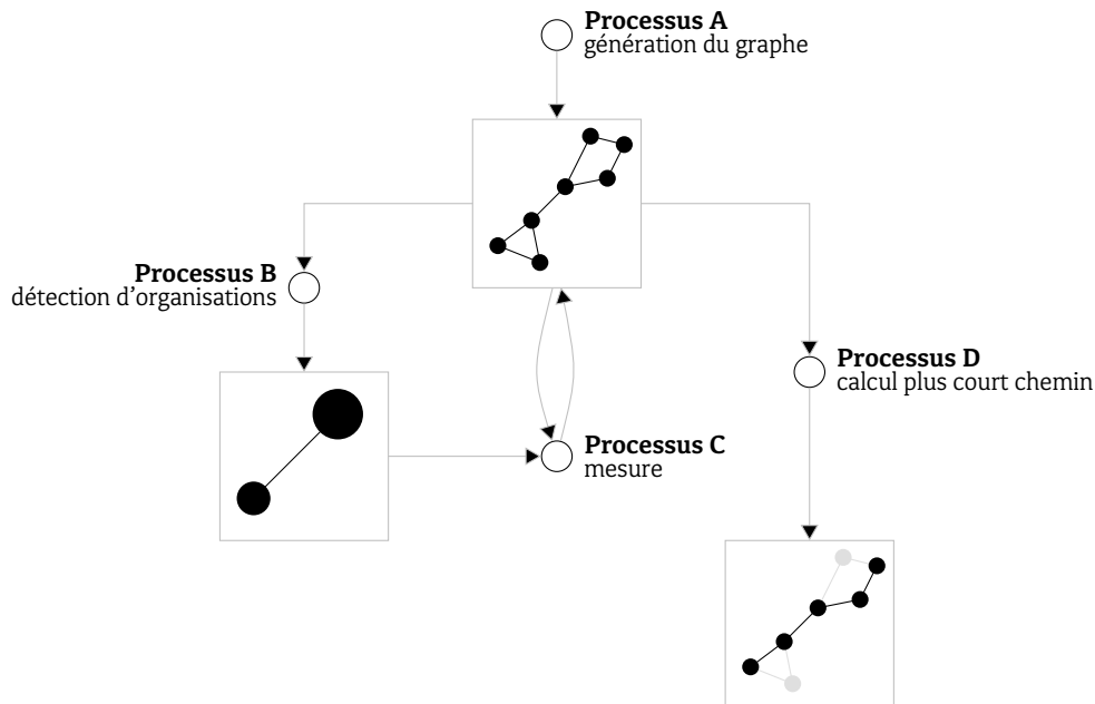
FIGURE 3.15 : Un graphe dynamique vu comme le résultat d'un ensemble de processus
