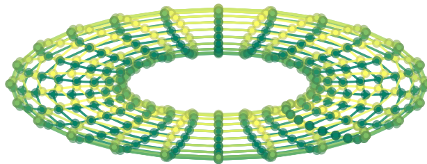
FIGURE B.2 : Un exemple de grille plaquée sur un tore
