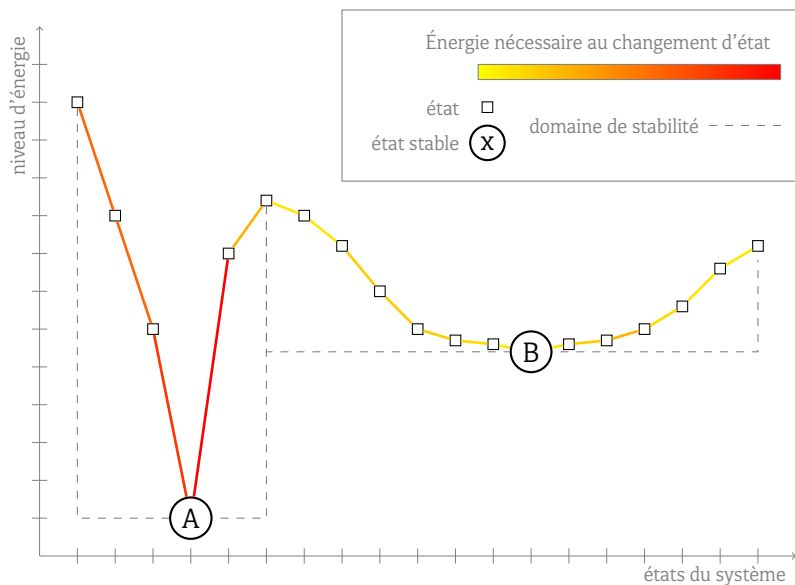
FIGURE 2.2 : Résilience d'ingénierie et résilience écologique. On constate qu'il faut plus d'énergie au système pour quitter l'état d'équilibre A que pour quitter l'état B : la résilience d'ingénierie est plus forte en A que en B . En revanche, le domaine de stabilité associé à l'état B est plus important que celui associé à l'état A : la résilience écologique de B est plus forte que celle de A .
