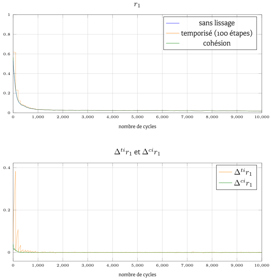
FIGURE 10.4 : Tracé de la mesure r_1 pour la simulation S_1 . La différence moyenne entre la mesure de r_1 pour le lissage temporisé et celle de la méthode sans lissage est 3.87 \cdot 10^{-3} avec un écart type de 2.81 \cdot 10^{-2} . Pour le lissage par cohésion, cette différence moyenne est de 1.65 \cdot 10^{-4} avec un écart type de 1.88 \cdot 10^{-3}
