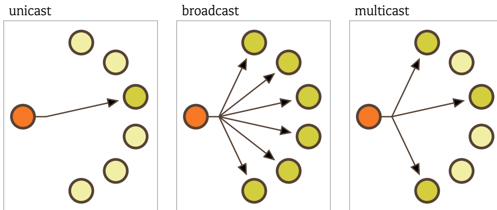
FIGURE 11.4 : Différences entre unicast, broadcast et multicast. Une source ● diffuse de l'information aux cibles ● .
