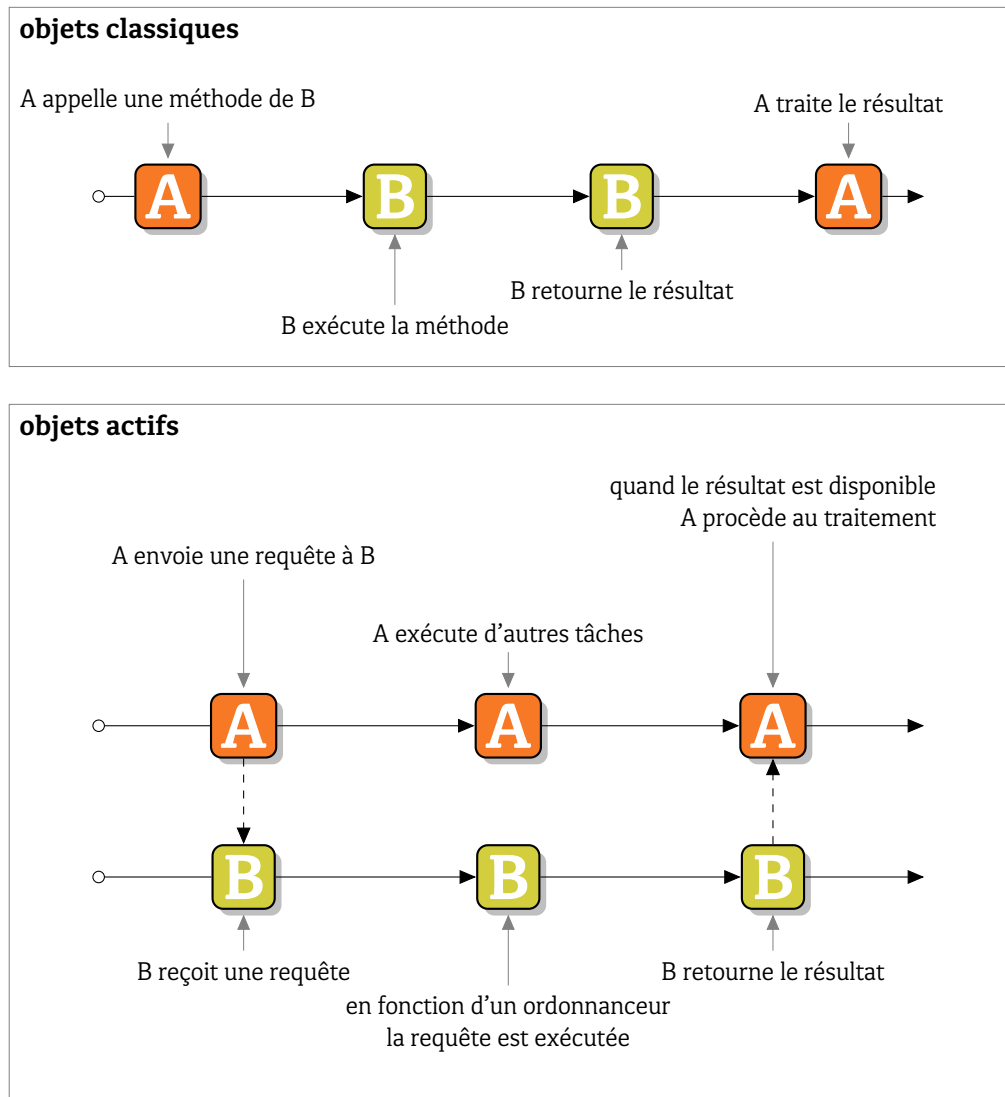
FIGURE 11.1 : Appel de méthode entre objets classiques et objets actifs. Un objet A appelle une méthode d'un objet B. B exécute alors cette méthode et retourne un résultat à A qui effectue alors un traitement.
