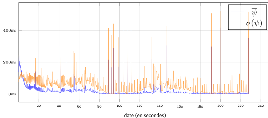
FIGURE 11.6 : Synchronisation des lucioles. La valeur moyenne \bar{\psi} de la mesure \psi , ainsi que son écart type \sigma(\psi) .
