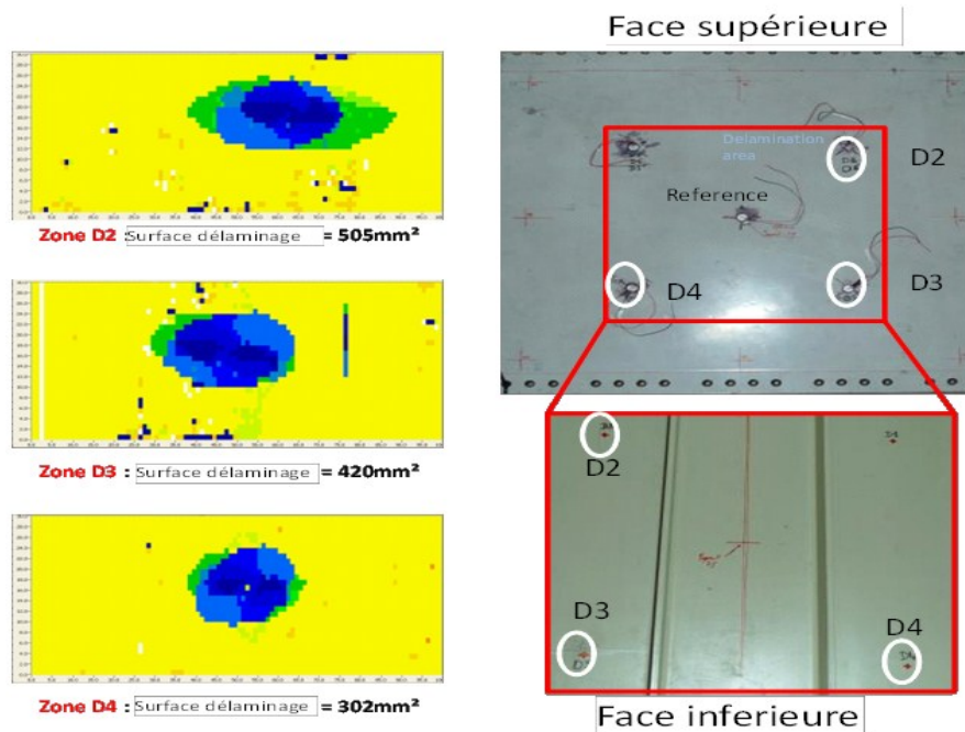
Figure 101 C-scan des différents délaminages ainsi que leurs localisations sur la structure composite
