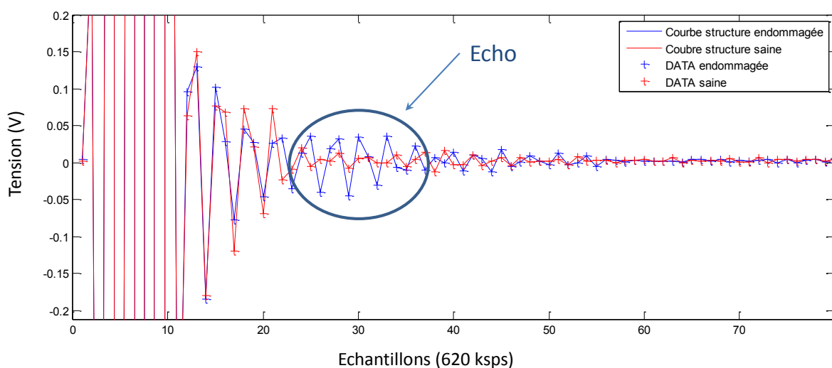
Figure 128 : affichages des données reçues
