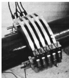
Emetteur peigne. Les transducteurs sont en contact direct avec la structure. Le collage est assuré par un serrage mécanique
