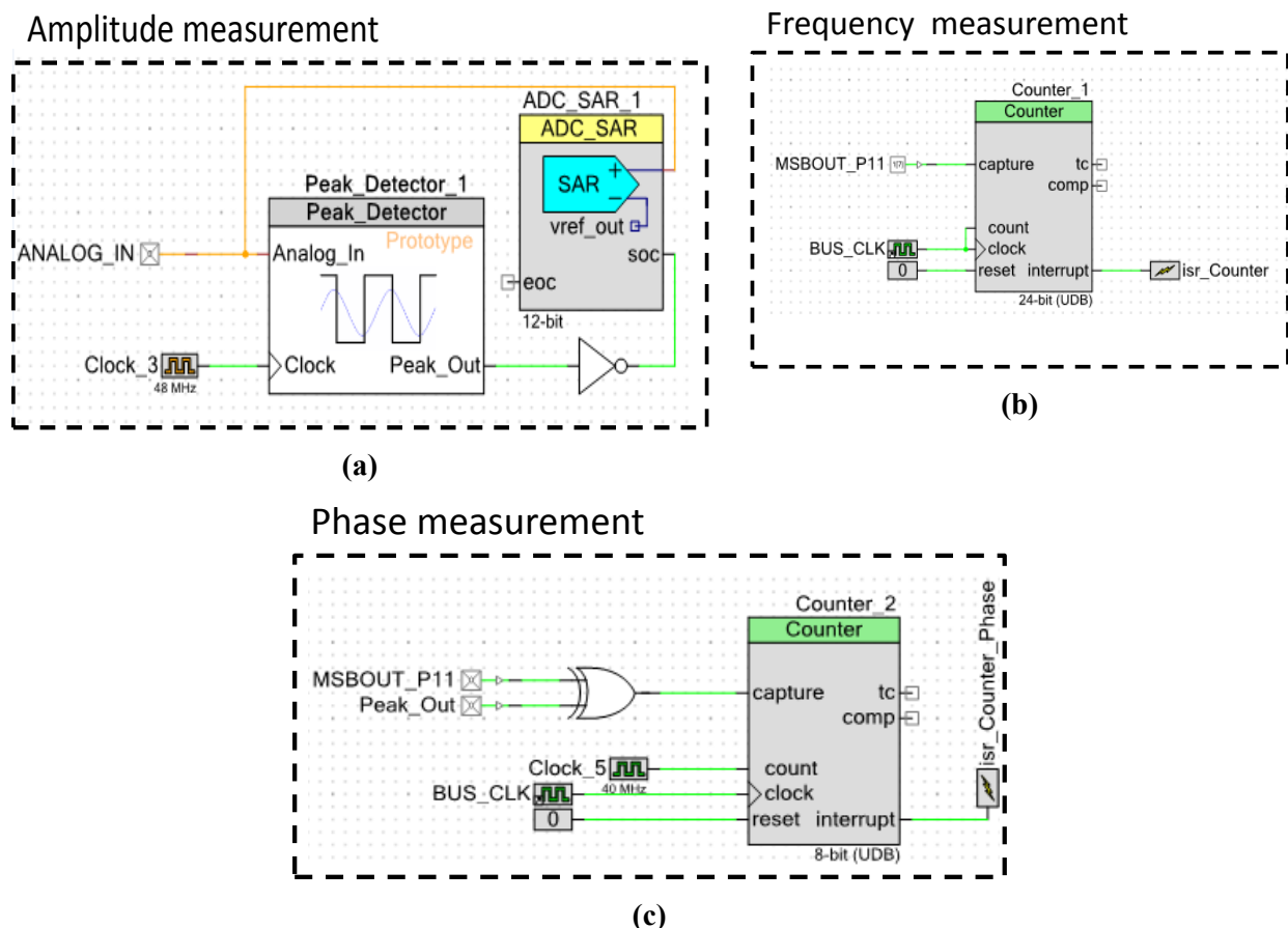
Figure 131 : (a) Mesure de l'amplitude par l'ADC. Le détecteur de pic déclenche l'acquisition (b) Mesure de fréquence par comptage. Résolution de 0.66ns.(c) Calcul de phase. Résolution de \Delta T égale à 0.25ns
