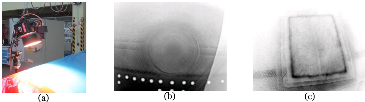
Figure 31 : Thermographie par spot IR : structures horizontales. (a) le dispositif (b) et (c) identification par contrast [44]
