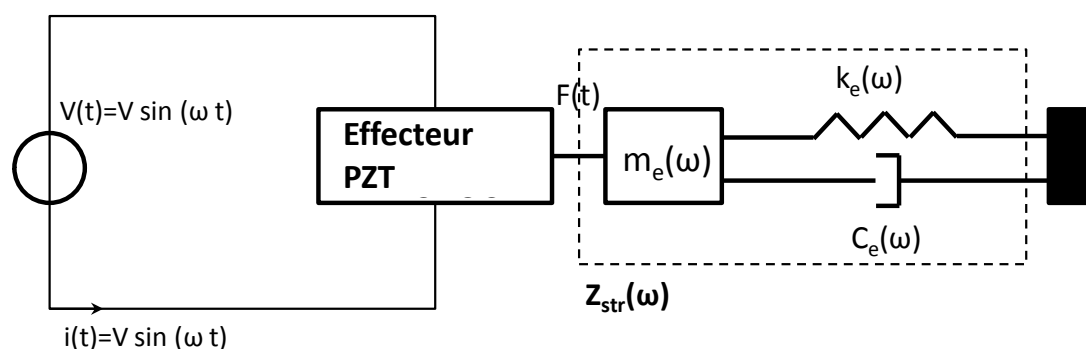
Figure 88 : Schéma équivalent mécanique de l'ensemble effecteur structure
