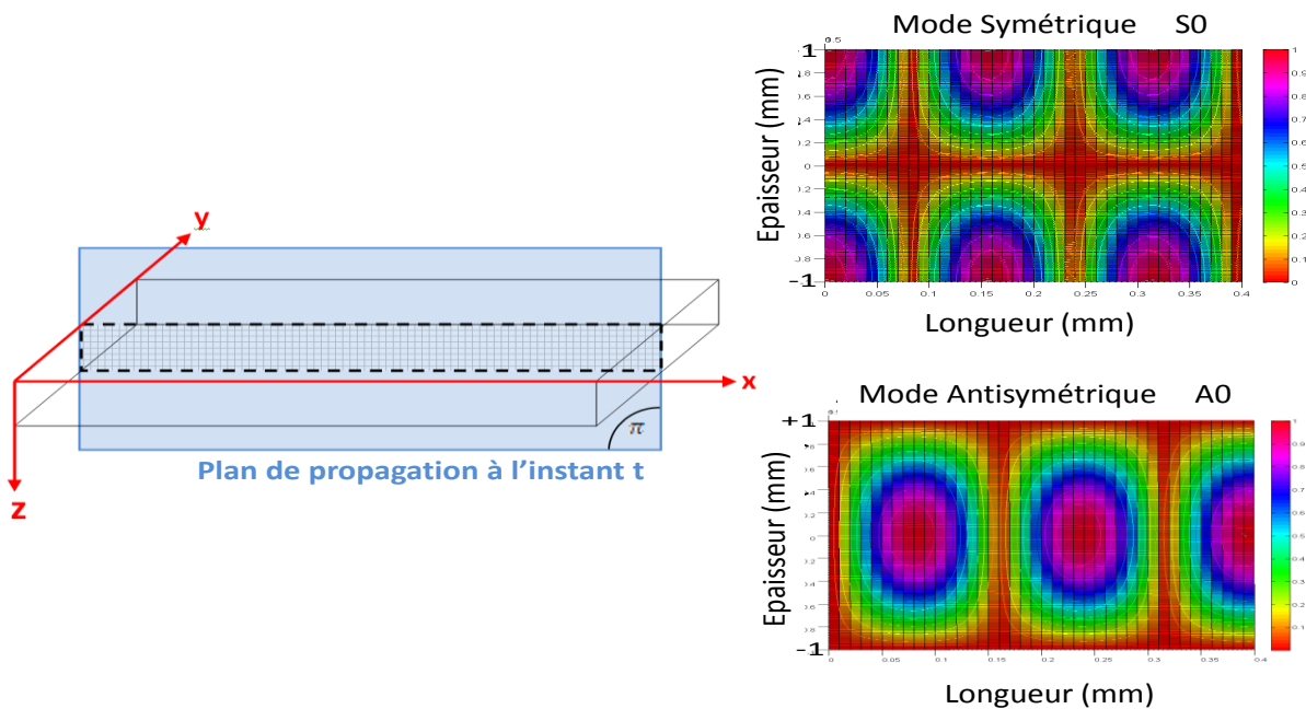
Figure 45 : Champs de déformations produites par les modes fondamentaux A0 et S0 à l'intérieur d'une plaque d'AL2024 d'épaisseur 2mm.
