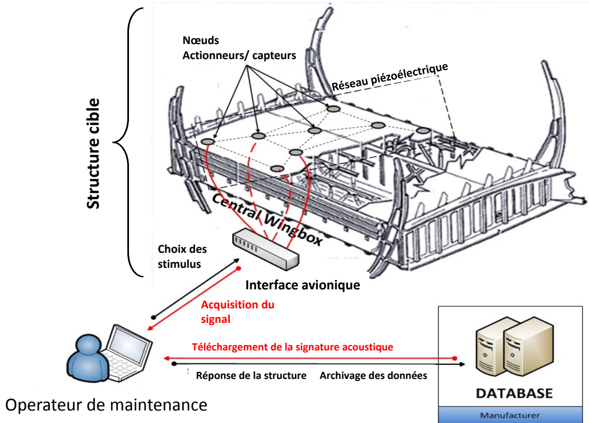
Figure 114 : Descriptif sommaire de l'intégration SHM et méthodologie de diagnostic
