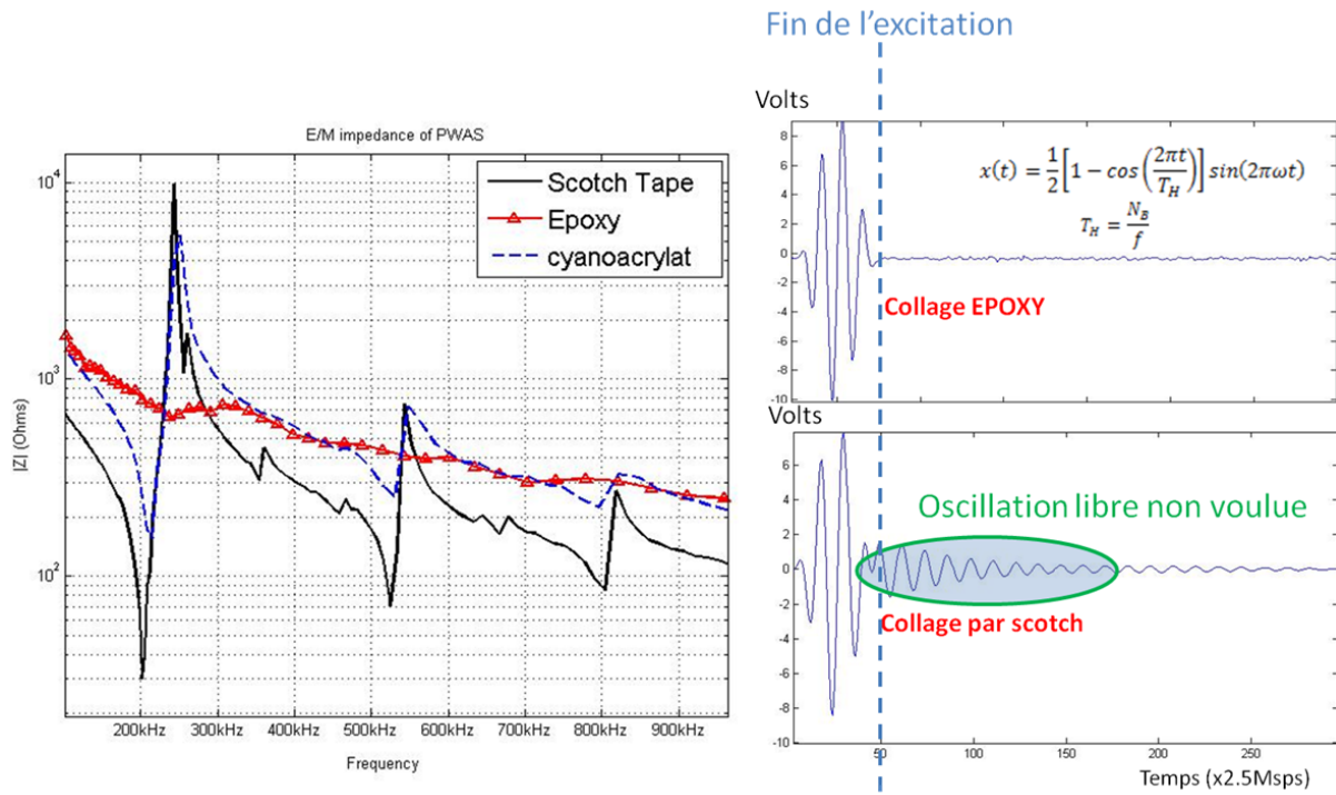
Figure 53 : caractéristiques fréquentielle et temporelle d'un collage par époxy et d'un collage par simple scotch
