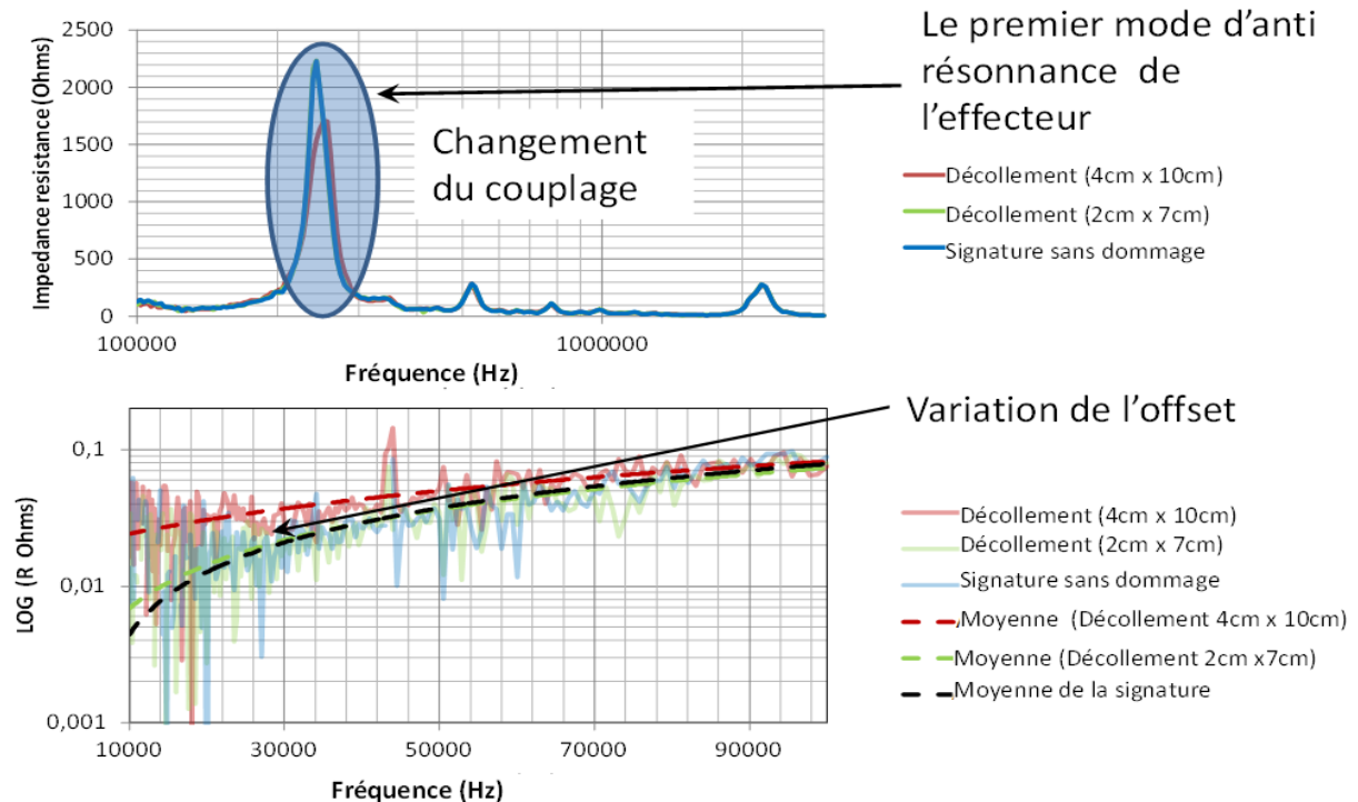
Figure 107 : Mesure de l'Impédance électromécanique de l'effecteur 3. (a) Premier mode d'antirésonance de l'effecteur ; (b) variation de l'offset
