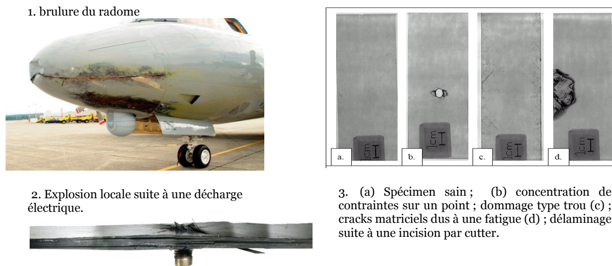
Figure 25 : Photos montrant différents dommages sur des matériaux composites de structures d'avion. (1) Brûlure du radome d'un Lockheed P-3 Orion. (2) Explosion suite à un foudroiement. (3) Radiographie X de différents types de dommages sur matériaux composites
