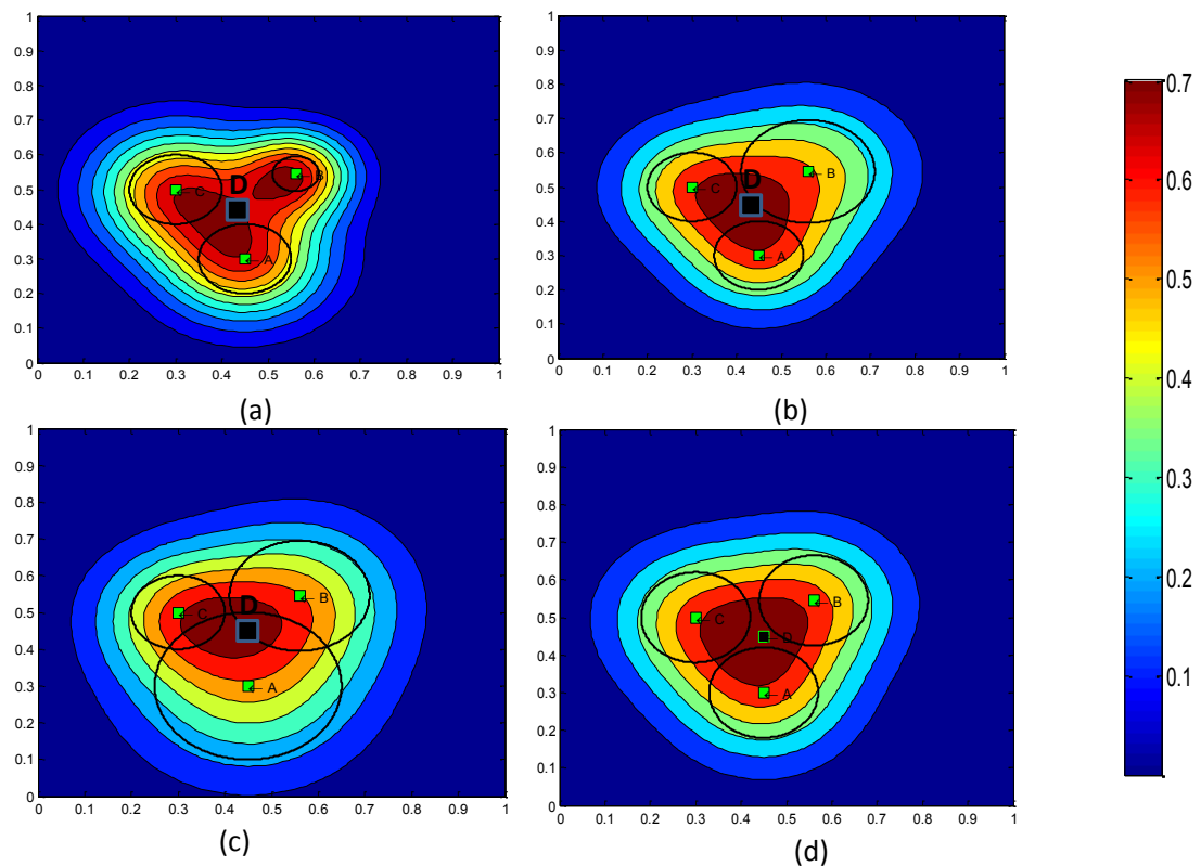
Figure 73 : Différents cas d'estimation de la probabilité de localisation d'un défaut par la technique de triangulation.
