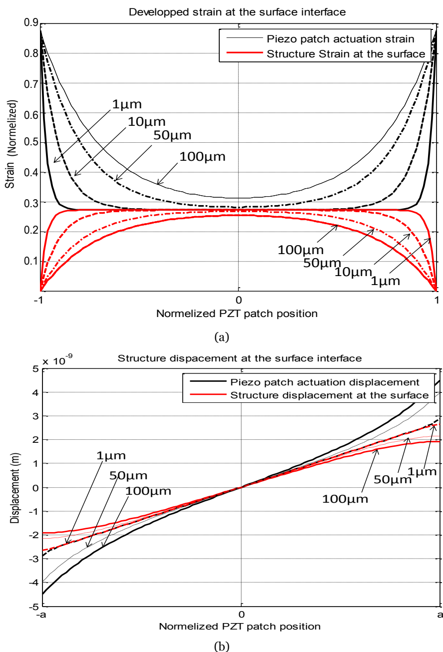
Figure 52 : (a) Courbes donnant la déformation calculée à l'interface effecteur / structure (b) Déplacement de matière à l'interface effecteur / matière. Pour une interface de 1\mu\text{m} , la totalité du déplacement de matière produit par l'effecteur est transmise à la structure
