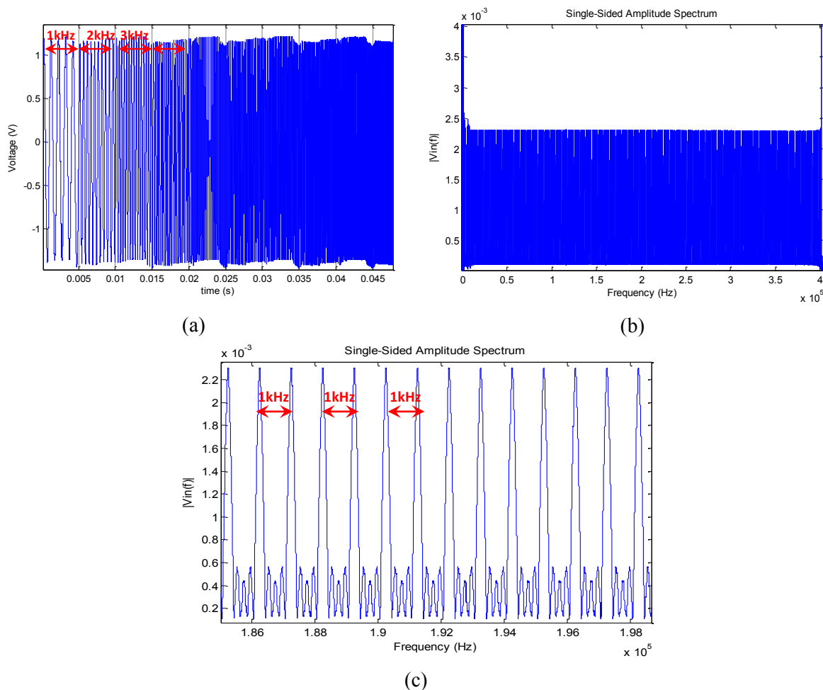
Figure 130 : (a) Stimulus généré sur l'intervalle temporel [0 ; 0.045s]. (b) Réponse spectrale du stimulus (c) zoom sur la réponse spectrale.
