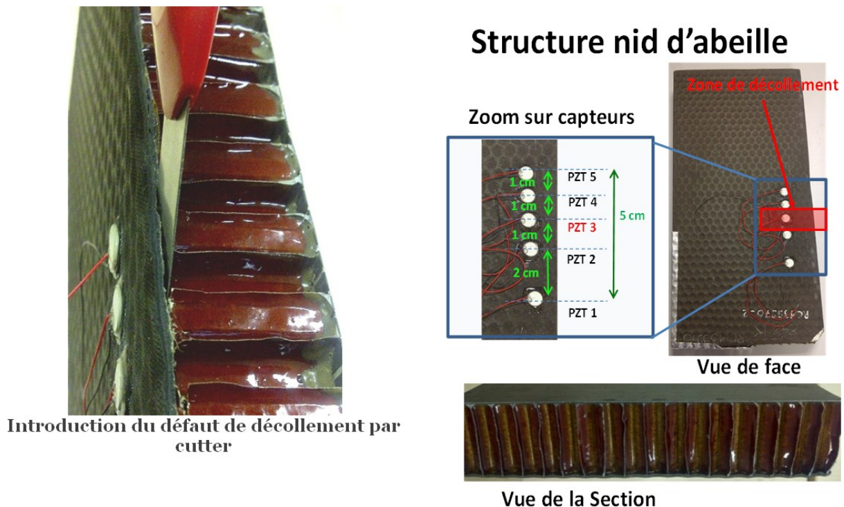
Figure 106 : Spécimen de structure en nid d'abeilles utilisée pour nos tests
