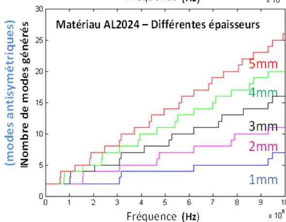
Figure 44: Nombre de modes générés dans le cas des propagations symétriques et antisymétriques dans une plaque d'AL2024 d'épaisseur variable.
