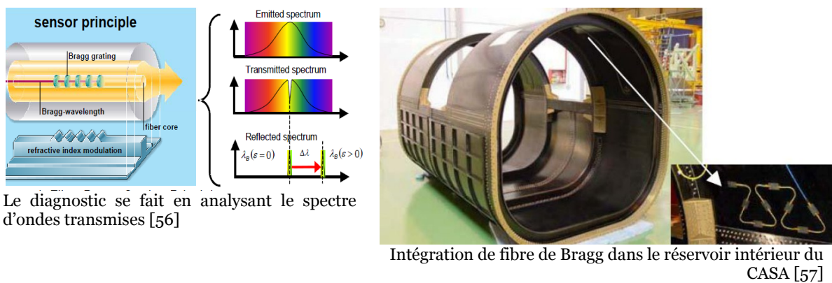
Figure 35 : Principe et intégration de la fibre de Bragg
