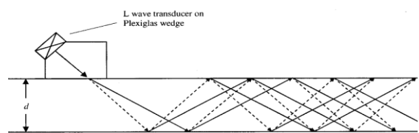
Génération d'ondes avec un angle oblique assuré par une cale en Perspex
