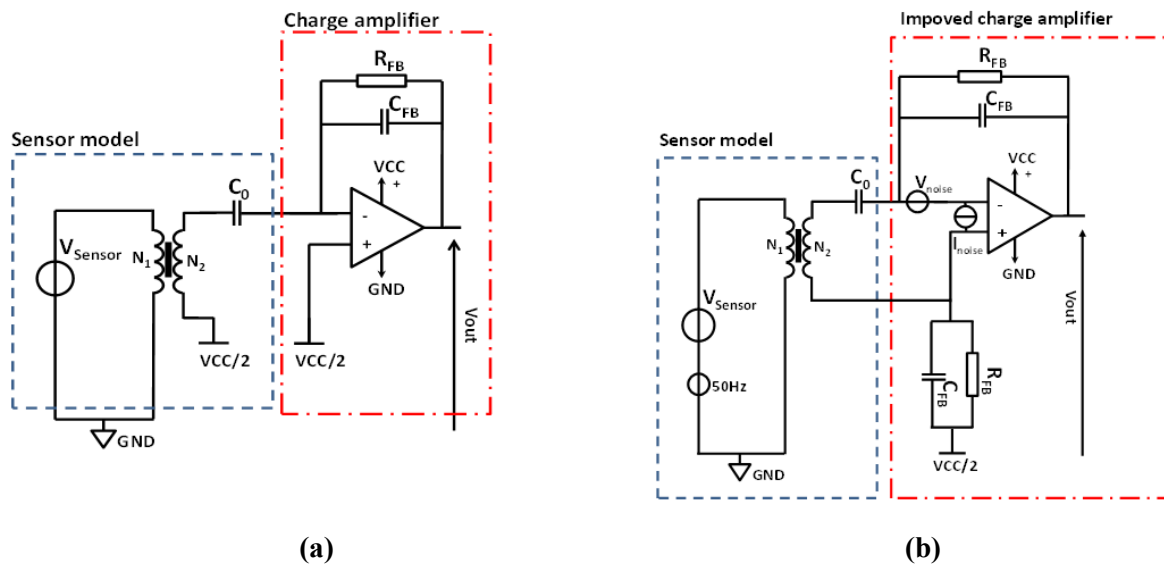
Figure 117 : Modélisation du capteur piézoélectrique avec son interface de collage et l'amplificateur de charges. (a) : modèle de base. (b) : Amplificateur avec des entrées différentielles équilibrées en impédance.
