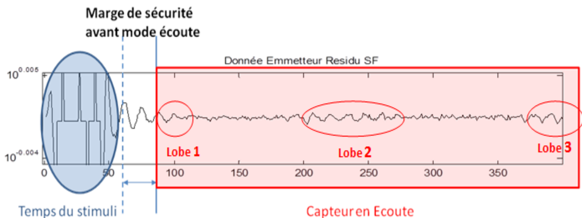
Figure 68 : Courbe représentant le résidu de la soustraction entre la signature et le signal temporel en semi-log de la plaque avec défauts pour le piezo actif : PZT B
