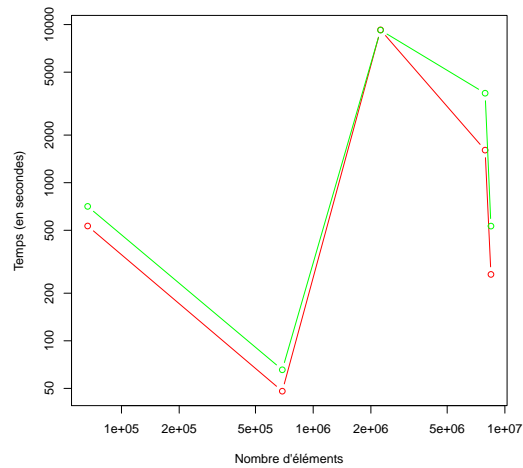
FIGURE 4.5 – Temps d'exécution du remaillieur en fonction du nombre d'éléments après remaillage, sans renumérotation préalable (en vert) et avec renumérotation préalable au moyen de l'outil SCOTCH (en rouge).
