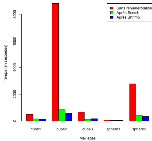
FIGURE 4.18 – Comparaison des temps d'exécution de la phase P_2 du remaillageur sur des maillages bruts, renumérotés avec SCOTCH et avec SHRIMP.
