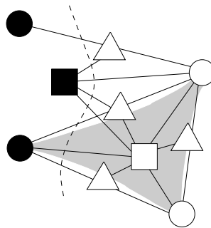
FIGURE 3.19 – Exemple de graphe enrichi distribué sans recouvrement restreint au processeur 2.
