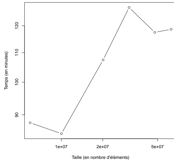
FIGURE 3.28 – Temps d'exécution de l'implémentation de l'équation de Poisson en utilisant Jacobi comme méthode de résolution, pour des maillages de tailles croissantes en gardant une charge moyenne de deux millions d'éléments par processeur.
