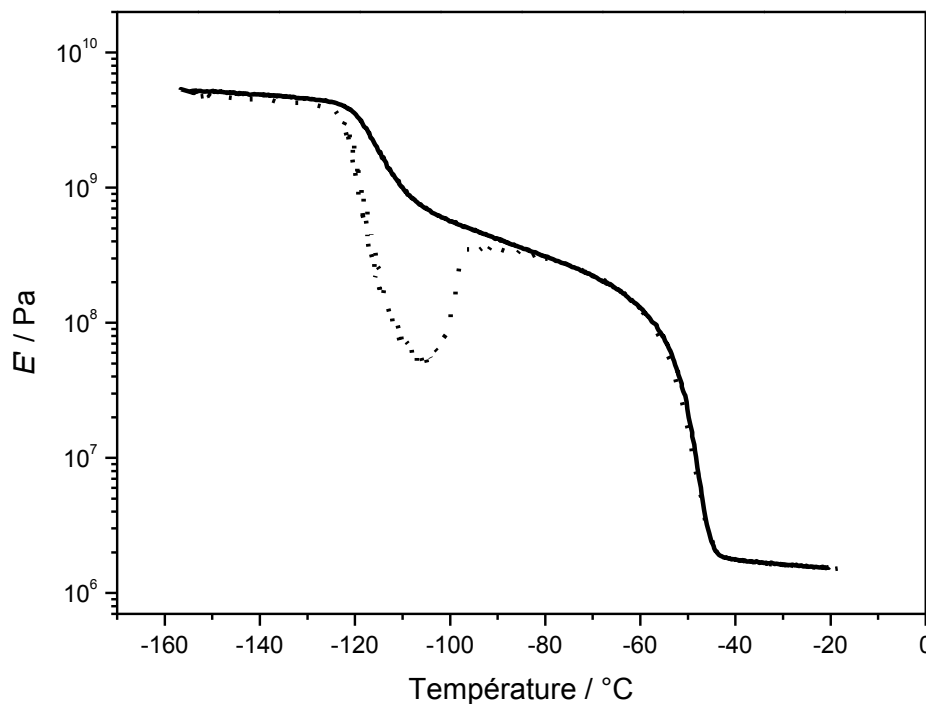
Figure V-11 : Evolution de E' pour le PDMS en fonction de la température (ligne : échantillon semi-cristallin, points : échantillon amorphe) lors de la chauffe ( 1 \text{ K}\cdot\text{min}^{-1} )
