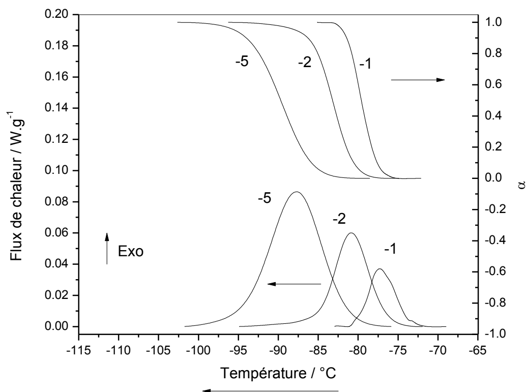
Figure V-27 : Thermogrammes et taux de cristallinité relatifs ( \alpha ) du PDMS/SiO 2 (c) en fonction de la température obtenus à différentes vitesses de refroidissement (K.min -1 )
