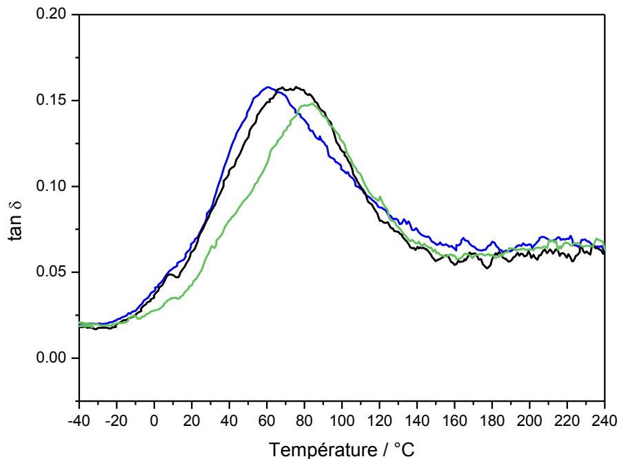
Figure III-21 : Evolution de \tan \delta du PFA (noir), du PFA/ SiO 2 (s) (bleu) et du PFA/SiO 2 (s)-furane (vert) en fonction de la température
