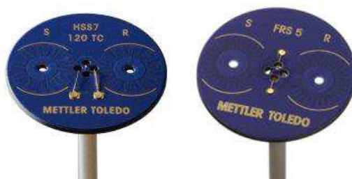
Figure II-16: Capteurs Mettler-Toledo HSS7 et FRS5
