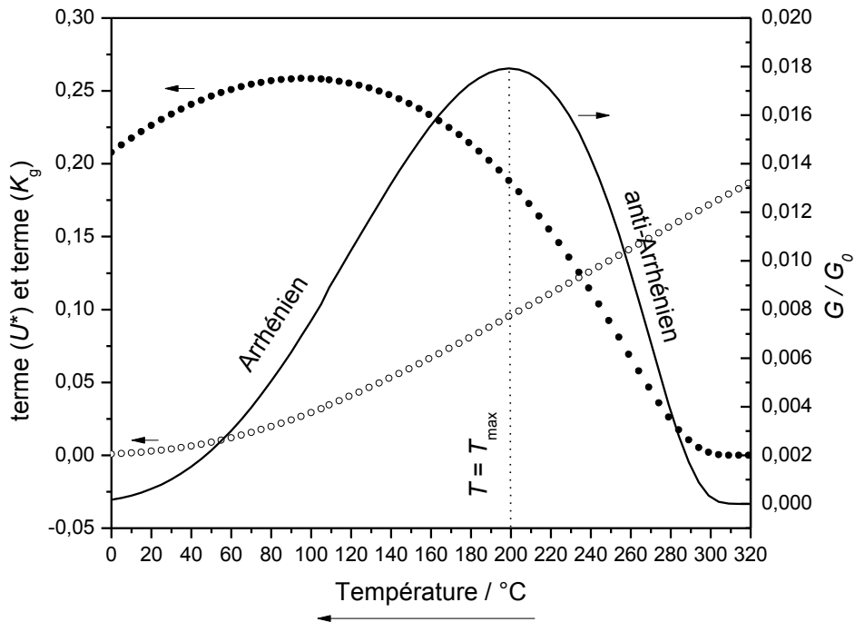
Figure IV-11 : Evolution de la vitesse de croissance des cristaux ( G/G_0 ), de la nucléation (cercles pleins : terme ( K_g )) et de la diffusion (cercles vides : terme ( U^* )) en fonction de la température
