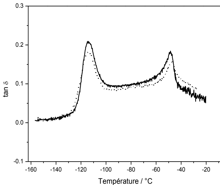
Figure V-13 : Evolution de \tan \delta du PDMS (ligne) et du PDMS/SiO 2 (c) (points) semi-cristallins en fonction de la température
