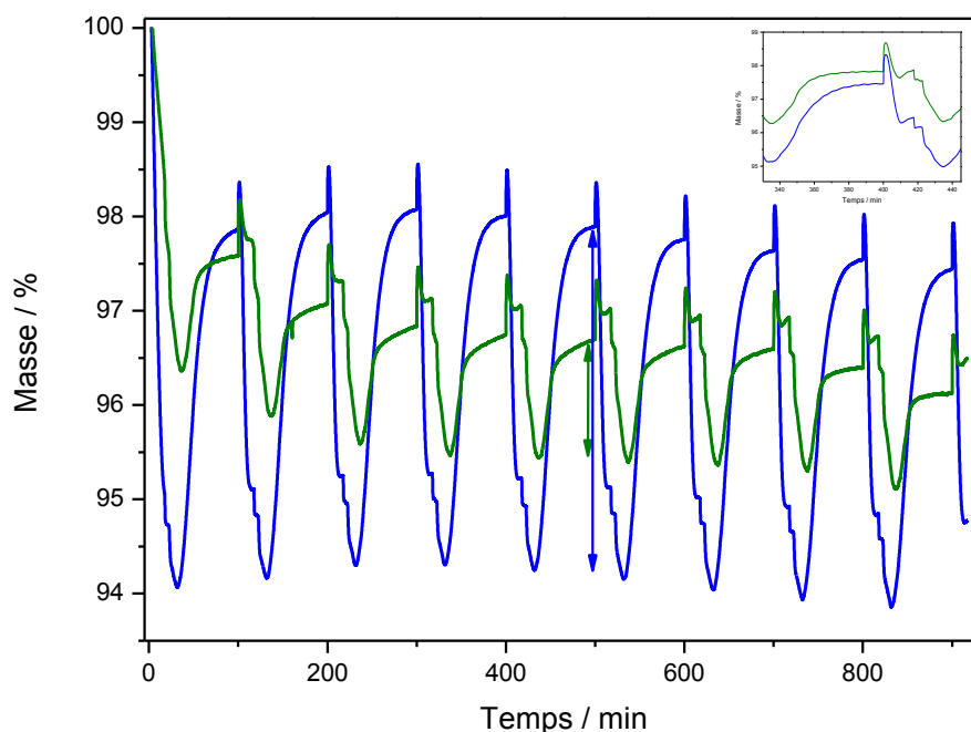
Figure III-14 : Thermogramme des silices SiO 2 (s) (bleu) et SiO 2 (s)-furane (vert) lors des cycles d'adsorption/désorption
