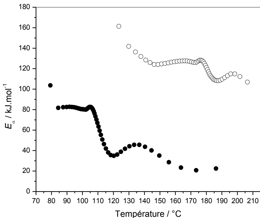
Figure III-39 : Dépendance de E_a pour la polymérisation du FA/SiO 2 (c) (cercles blancs) et du FA/SiO 2 (c)/MA (cercles noirs) en fonction de la température
