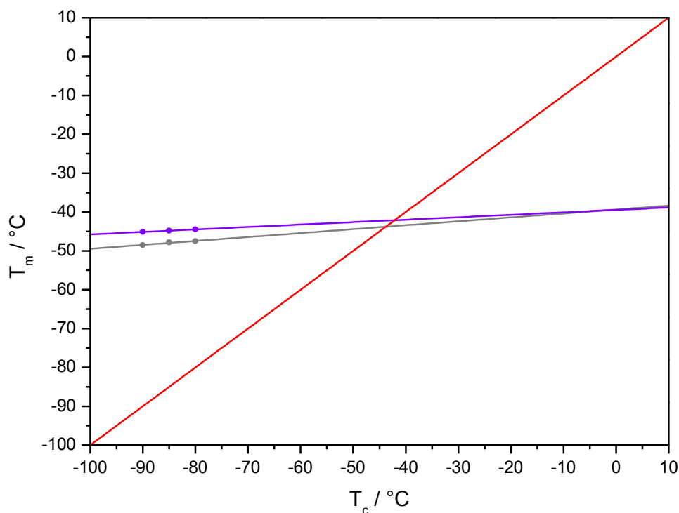
Figure V-25 : Evaluation de T_m^0 pour le PDMS (gris) et le PDMS/SiO 2 (c) (violet) à l'intersection de la droite d'équation T_m = T_c (rouge)
