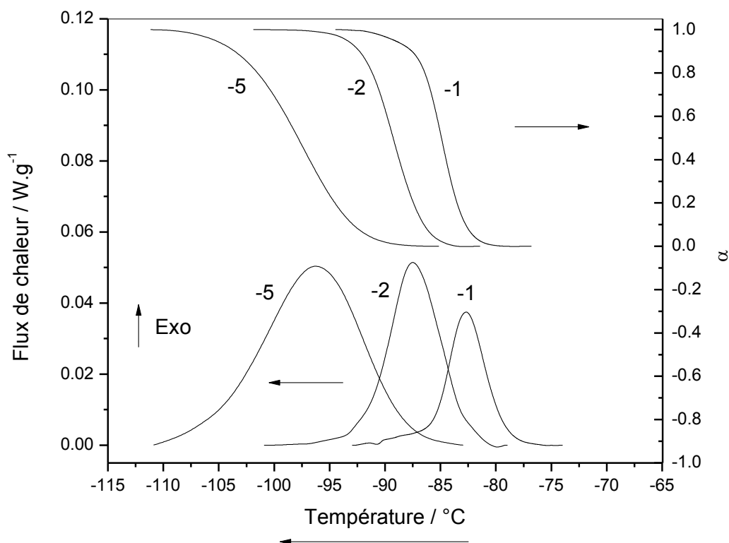
Figure V-26 : Thermogrammes et taux de cristallinité relatifs ( \alpha ) du PDMS en fonction de la température obtenus à différentes vitesses de refroidissement ( \text{K}\cdot\text{min}^{-1} )
