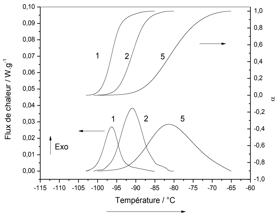
Figure V-29 : Thermogrammes et taux de cristallinité relatifs ( \alpha ) du PDMS en fonction de la température obtenus à différentes vitesses de chauffe ( \text{K}\cdot\text{min}^{-1} )
