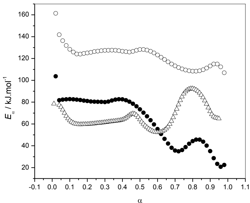
Figure III-38 : Dépendance de E_\alpha pour la polymérisation du FA/MA (triangles), FA/SiO 2 (c) (cercles vides) et du FA/SiO 2 (c)/MA (cercles pleins) en fonction du taux de conversion \alpha
