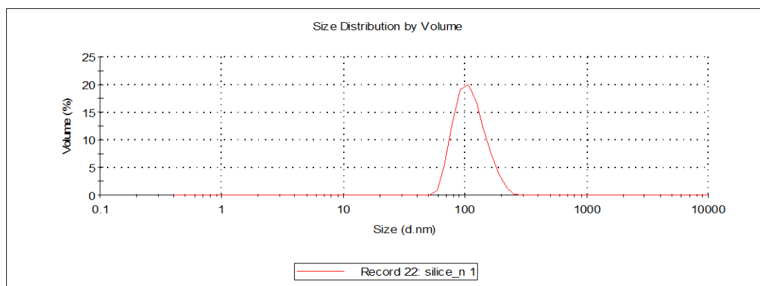
Figure III-10 : Distribution en volume de la taille des particules de silice SiO 2 (s)
