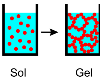
Figure II-8 : Formation du réseau de silice lors de la transition sol-gel
