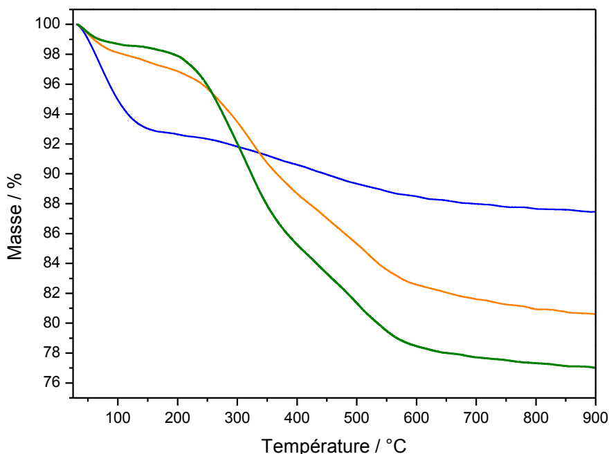
Figure III-13 : Thermogramme des silices \text{SiO}_2(\text{s}) (bleu), \text{SiO}_2(\text{s}) -epoxy (orange) et \text{SiO}_2(\text{s}) -furane (vert)
