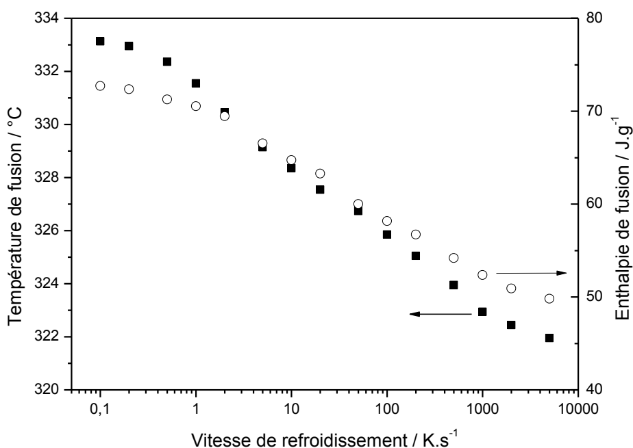
Figure IV-6 : Température (carrés) et enthalpie (cercles) de fusion (mesurées par FSC à 1000 \text{ K.s}^{-1} ) en fonction de la vitesse de refroidissement employée lors de la cristallisation
