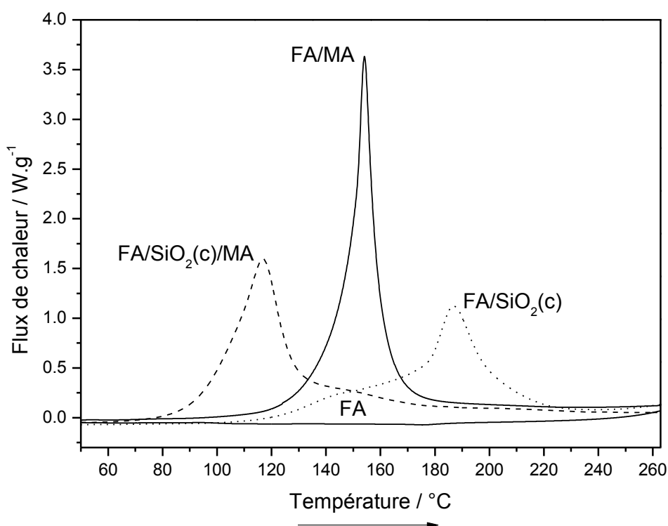
Figure III-36 : Evolution du flux de chaleur en fonction de la température lors de la polymérisation ( 6 \text{ K}\cdot\text{min}^{-1} )
