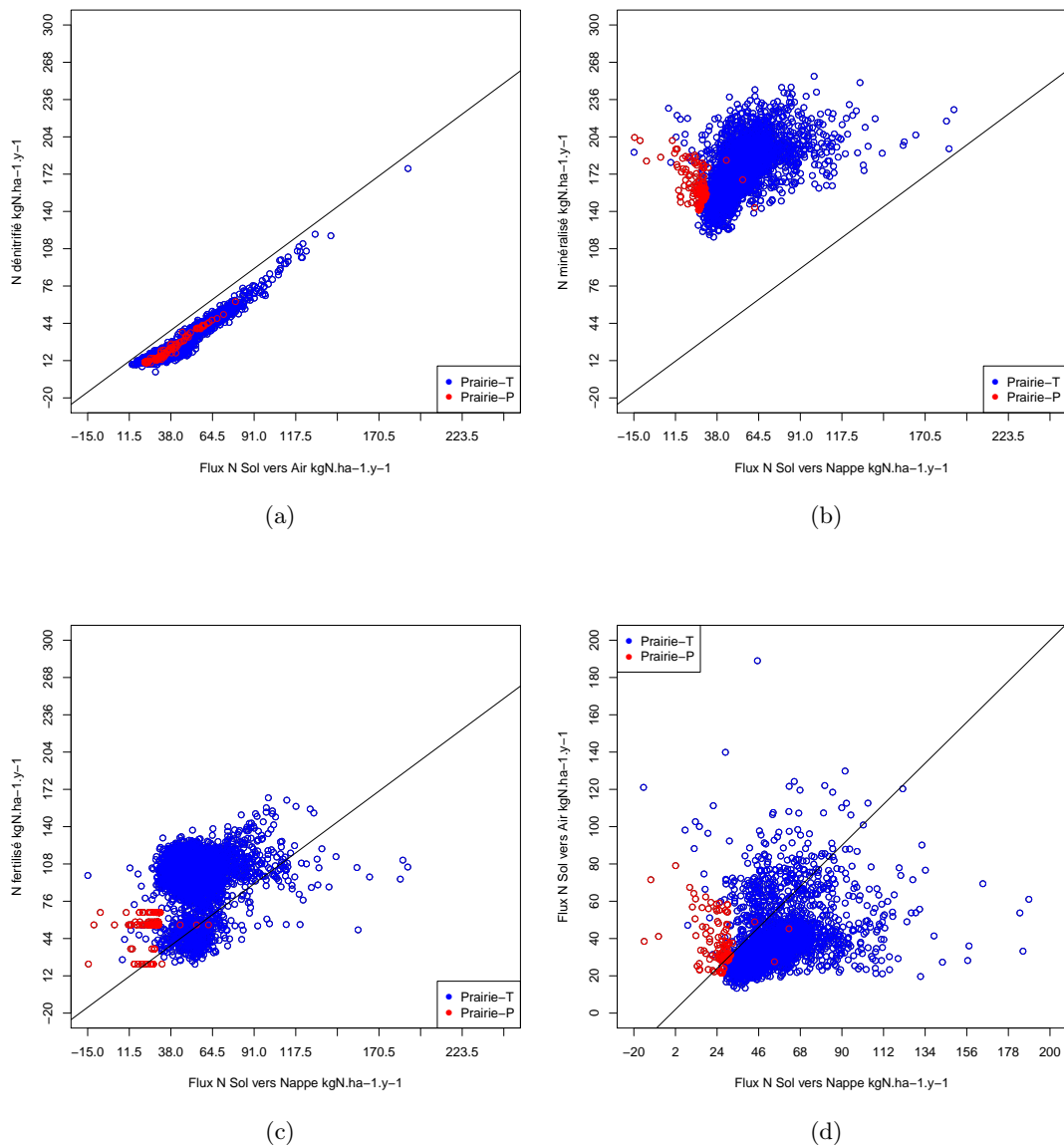
FIGURE 3.8 – Analyse de processus à l'échelle de la parcelle : (a) N dénitriqué vs. Flux N Sol vers Air, (b) N minéralisé vs. Flux N Sol vers Nappe, (c) N fertilisé vs. Flux N Sol vers Nappe, et (d) Flux N Sol vers Nappe vs. Flux N Sol vers Air
