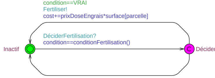
FIGURE 6.3 – Automate de coût de contrôle de fertilisation
