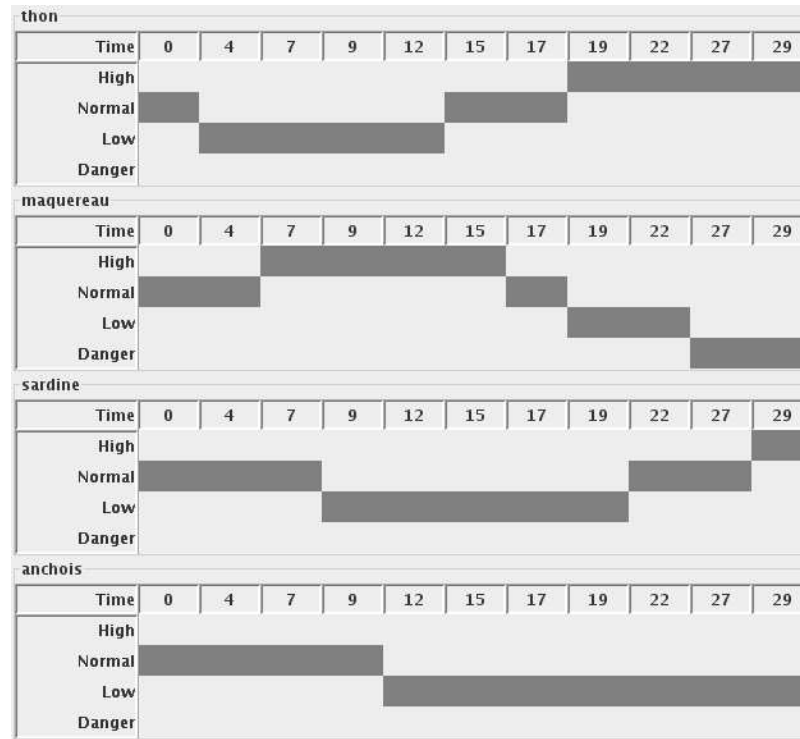
FIGURE 3.13 – Trace menant à la situation 1 (thon : High , maquereau : Danger , sardine : High , anchois : Low )
