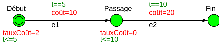
FIGURE 6.2 – Un exemple d'automate temporisé de coût
