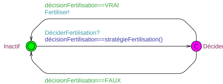
FIGURE 5.7 – Automate de contrôleur de fertilisation
