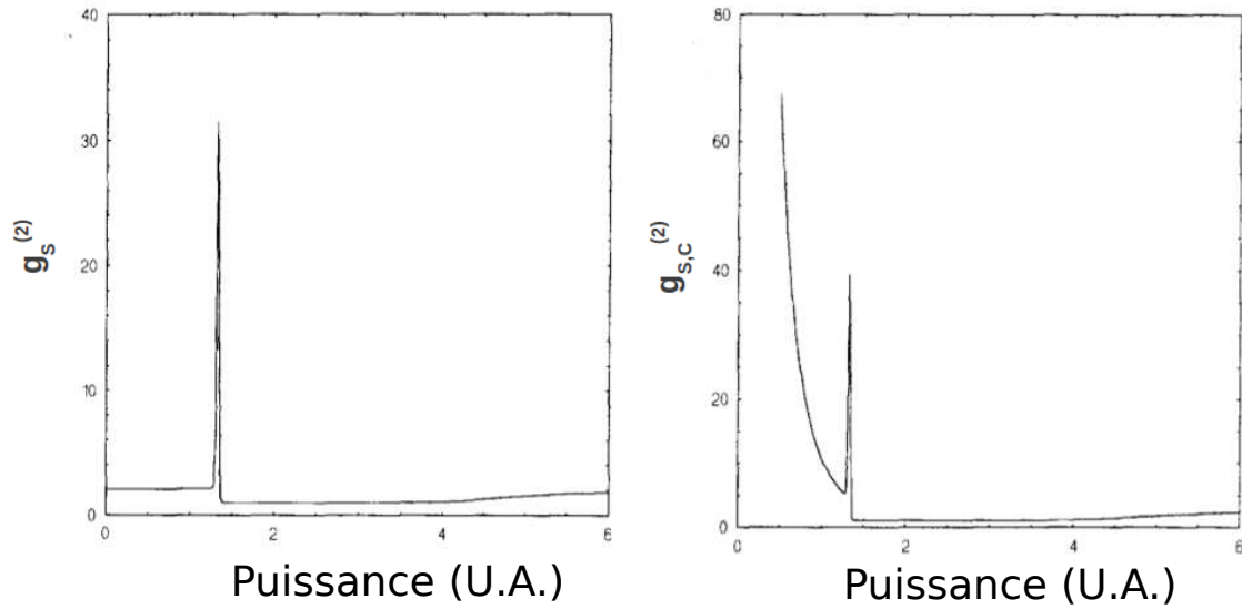
Figure 1.12 : Figure adaptée de la référence [63]. A gauche g_s^{(2)}(0) , à droite g_{s,c}^{(2)}(0) en fonction de la puissance d'excitation. La valeur de puissance de seuil est environ 1.5 (U.A.).
