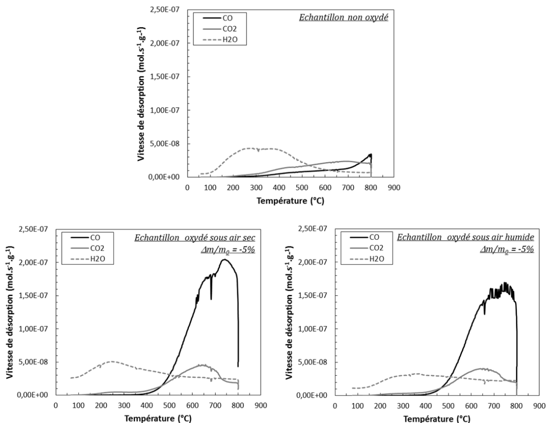
Figure 26 : Profil des principaux gaz désorbés lors d'un cycle de TPD pour des échantillons de carbone ex-résine non oxydés et oxydés sous air sec et air humide à T = 400^{\circ}C ( \Delta m/m_0 = -5\% ).
