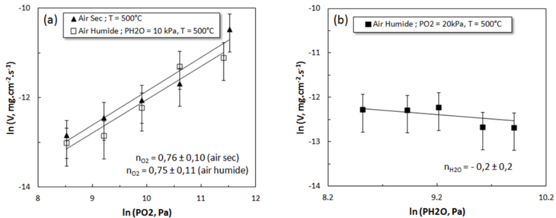
Figure 16 : Dépendance de la vitesse d'oxydation du pyrocarbone à T = 500^{\circ}\text{C} en fonction des pressions partielles en espèces oxydantes. (a) dépendance en fonction de \text{PO}_2 . (b) dépendance en fonction de \text{PH}_2\text{O} .
