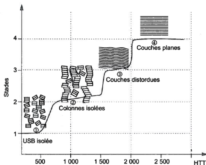
Figure 7 : Principaux stades d'organisation structurale de carbone en fonction de la température de traitement thermique [Oberlin 1984].
