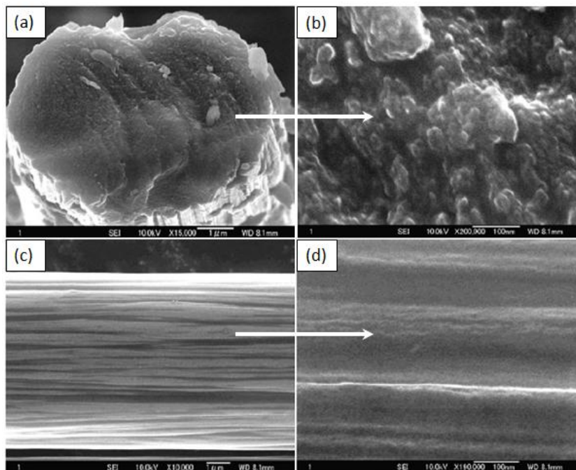
Figure 19 : Morphologie de la fibre de carbone ex-PAN T300. (a) et (b) morphologie transversale. (c) et (d) morphologie longitudinale. [Li 2012].
