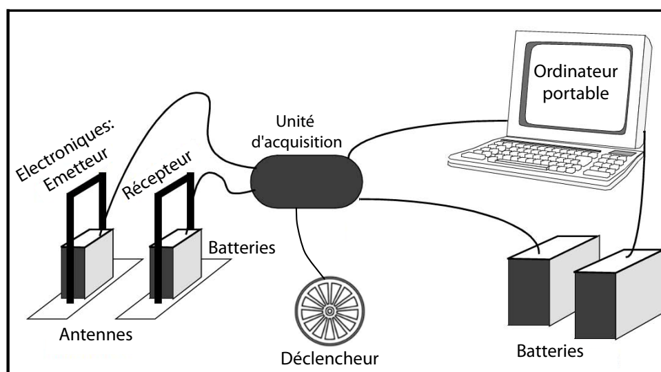
FIGURE 2.6 – Les différents composants d'un système GPR [d'après Bano, 2000 ].
