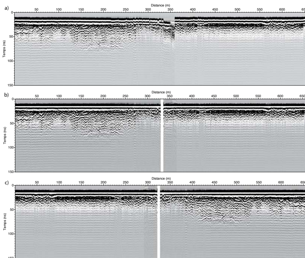
FIGURE 2.9 – a) Exemple de profil GPR brut avant traitement ; b) Profil GPR après correction du TO et ajout de traces blanches ; c) Profil GPR après édition.
