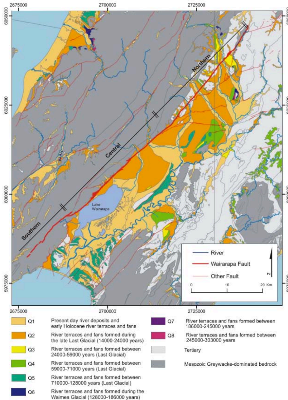
FIGURE 6.4 – Carte géologique simplifiée de la vallée de Wairarapa [Villamor et al., 2008].
