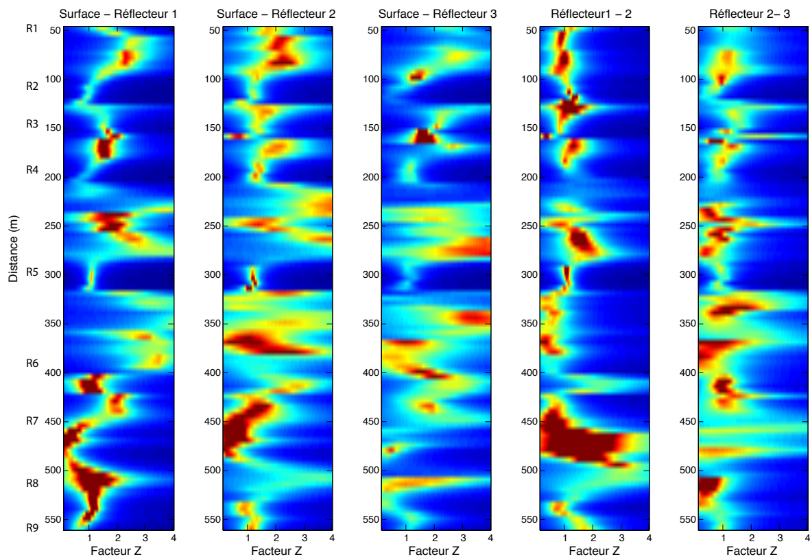
FIGURE 4.24 – Qualité de l’ajustement en fonction du facteur Z. L’ajustement est fait entre les profils topographiques de deux interfaces dont le nom est indiqué en haut de chaque graphique. Cet ajustement est calculé tous les 5 mètres le long de la coupe 4 (Fig. 4.9) sur une fenêtre large de 30 m. L’axe vertical représente la distance le long du profil avec indiqués la position et le nom des bords de terrasses. Les qualités d’ajustement, c’est à dire l’inverse de la moyenne des différences entre profils, croissent du bleu vers le rouge.
