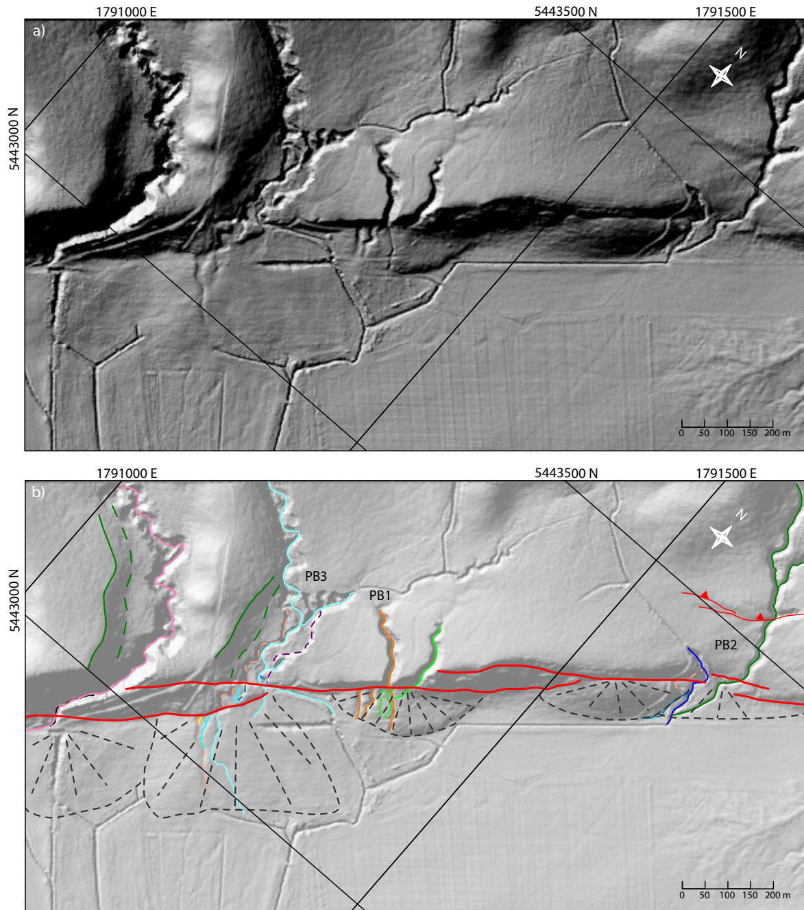
FIGURE 6.26 – Analyse de la surface du site de Pigeon Bush; a) MNT ombré LiDAR de la surface du site, illuminé depuis l'ouest; b) Cartographie préliminaire des traces de failles (en rouge) et des marqueurs morphologiques visibles en surface; les différentes couleurs distinguent les différents marqueurs; la base des talus est représentée en traits pointillés et les cônes alluviaux sont représentés par des traits pointillés gris.
