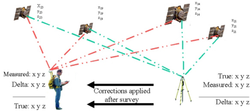
Supplement B- 1: Principe du GPS différentiel
