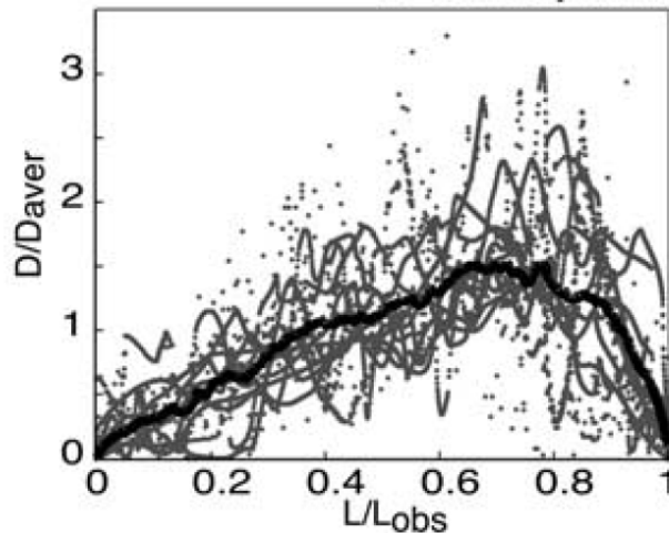
FIGURE 1 – Profils de déplacements cosismiques ( D , mesurés en surface) versus longueur ( L ) de 23 ruptures sismiques [d’après Manighetti et al., 2005 ]. Les profils ont été normalisés par la longueur de rupture ( L_{obs} ) et le déplacement moyen ( D_{aver} ). Les 23 profils montrent la même forme enveloppe, représentée par la fonction en trait épais qui moyenne l’ensemble des profils. Cette forme enveloppe générique est globalement triangulaire et fortement asymétrique. Elle montre que le déplacement cosismique varie fortement, mais néanmoins pas aléatoirement, le long des ruptures.
