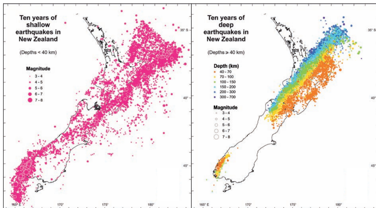
FIGURE 1.22 – Distribution de la sismicité ( M_w \geq 3 ) superficielle (< 40 km) à gauche et profonde (> 40 km) à droite ( http://www.gns.cri.nz/ ). Les cercles représentant les séismes de M_w > 5 sont bordés de traits blancs. La sismicité superficielle se répartie selon un axe SW-NE, depuis la fosse de Puysegur, puis le long de la faille Alpine, de la zone de failles de Marlborough, du faisceau de failles de l'île du Nord, jusqu'à la fosse d'Hikurangi au nord. La sismicité profonde décrit la géométrie de l'interface de subduction, qui s'interrompt sous l'île du Sud, au niveau de la chaîne des Alpes du Sud.
