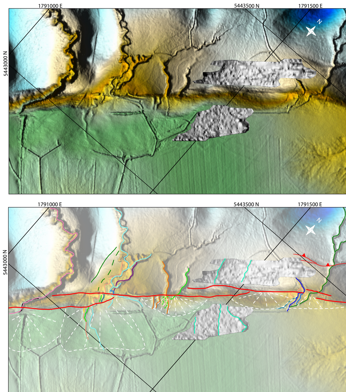
FIGURE 6.31 – MNT ombré de l'Horizon 2 pointé sur les données GPR 250 MHz sur le site de Pigeon Bush (a). b) Cartographie préliminaire des marqueurs identifiés en sub-surface sur les différents MNT. Les marqueurs visibles en surface sont rappelés en arrière plan (Fig. 6.8).
