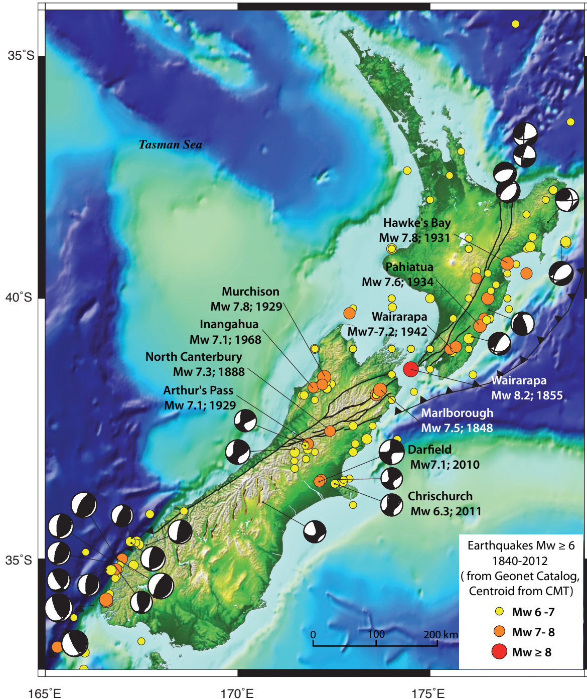
FIGURE 1.21 – Carte de localisation des séismes historiques superficiels de magnitude M_w \geq 6 ( http://www.geonet.org.nz/ ). Les mécanismes au foyer sont indiqués (Catalogue CMT). Des ruptures en surface sont généralement rapportées pour les séismes de M_w \geq 7 (rupture en surface du séisme de Darfield par exemple : http://www.youtube.com/watch?v=Npqx3WmNkv4 ). Le nom, la magnitude et la date des séismes sont précisés lorsqu'ils ont causé des victimes (Fond de carte réalisé à partir des données ASTER GDEM et GEBCO).
