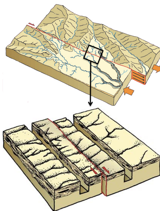
FIGURE 2 – Blocs diagrammes décrivant l'interaction du réseau de drainage avec une faille décrochante (en haut) et l'enfouissement progressif de chenaux abandonnés (en bas), préservés sous la sédimentation, accumulant passivement du déplacement (figures de J. Malavieille).
