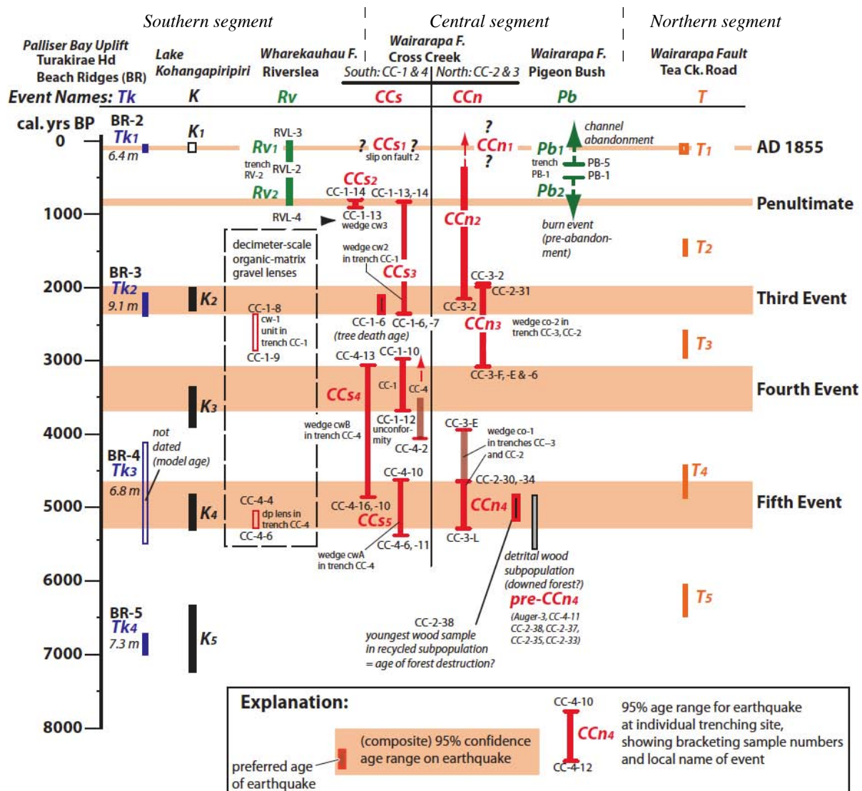
FIGURE 6.5 – Ages des séismes déduits des observations et des datations faites sur les plages soulevées de Turikae Head [McSaveney et al., 2006], sur des sédiments lacustres [Cochran et al., 2007], et dans différentes tranchées sur 4 sites [Little et al., 2009, Van Dissen and Berryman, 1996] le long des 3 segments de la faille de Wairarapa (Fig. 6.3) [d’après Little et al., 2009]. Les bandes horizontales colorées représentent les gammes d’âges de chaque séisme déduites de la combinaison de l’ensemble des données exceptées celles de Tea Creek Road, où les événements 2, 3 et 4 semblent s’intercaler entre ceux trouvés plus au sud.
