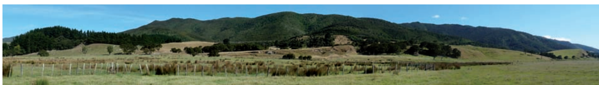
FIGURE 6.24 – Panorama du site de Pigeon Bush. Au premier plan, les joncs surlignent une zone marécageuse qui couvre une grande partie de la zone investiguée dans le compartiment inférieur de la faille. Ces marécages et la tourbe qu'ils contiennent, peuvent être responsables d'une diminution de la profondeur de pénétration. Au second plan apparaît l'escarpement de faille dont la hauteur varie de 0-20 m et dans lequel affleurent les dépôts de la terrasse d'aggradation. A l'arrière plan s'élèvent les montagnes de la chaîne Rimutaka (Fig. 6.3).
