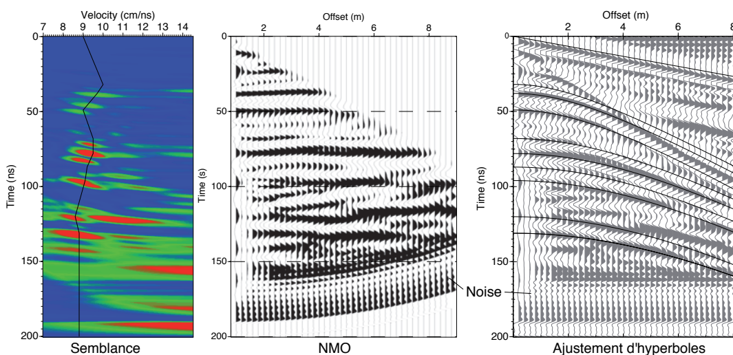
FIGURE 2.12 – Analyse de vitesse par semblance, Normal Moveout (NMO), et ajustement d'hyperboles.
