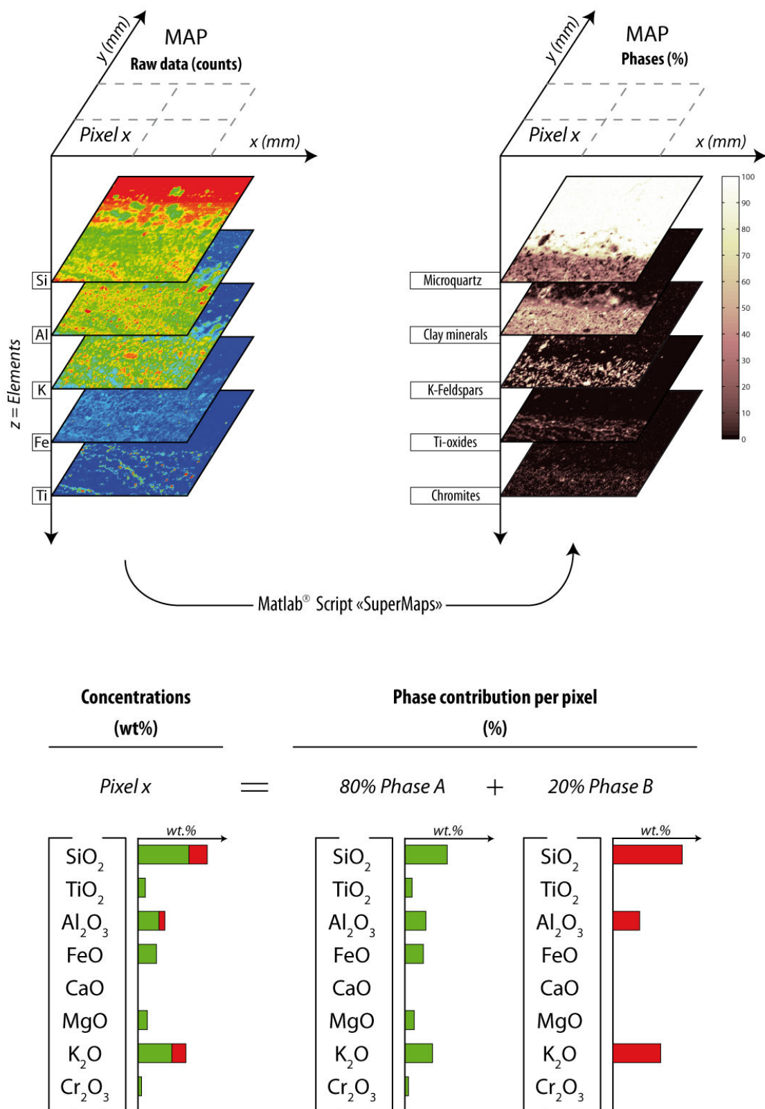
FIGURE A.4 – Schéma simplifié inspiré de Ulrich (2010) et représentant la conversion des cartographies élémentaires en cartographies de phases. Méthode basée sur le script Matlab "Supermaps" développé par Emmanuel Muñoz et Marc Ulrich à ISTerre, Grenoble (voir la description de la méthode dans Ulrich et al. submitted). Les données brutes sont préalablement converties en concentrations de poids d'oxydes grâce au logiciel Vision 32.
