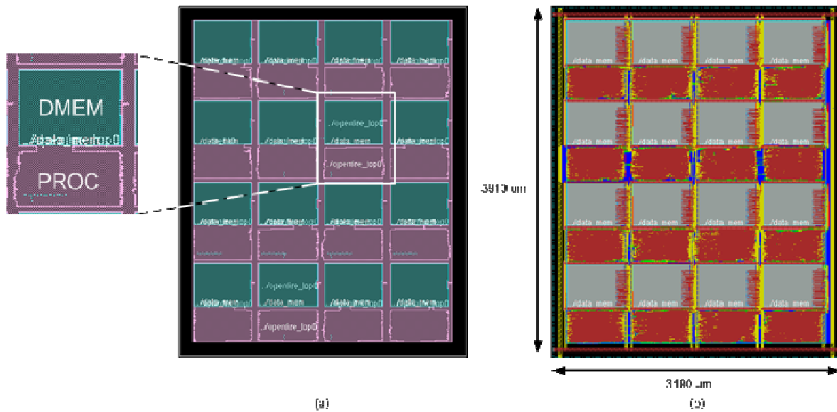
Figure 16: Étage inférieur de la 3D hétérogène d'empilement (a) vue amibes du plan de masse (b) mise en dérouté
