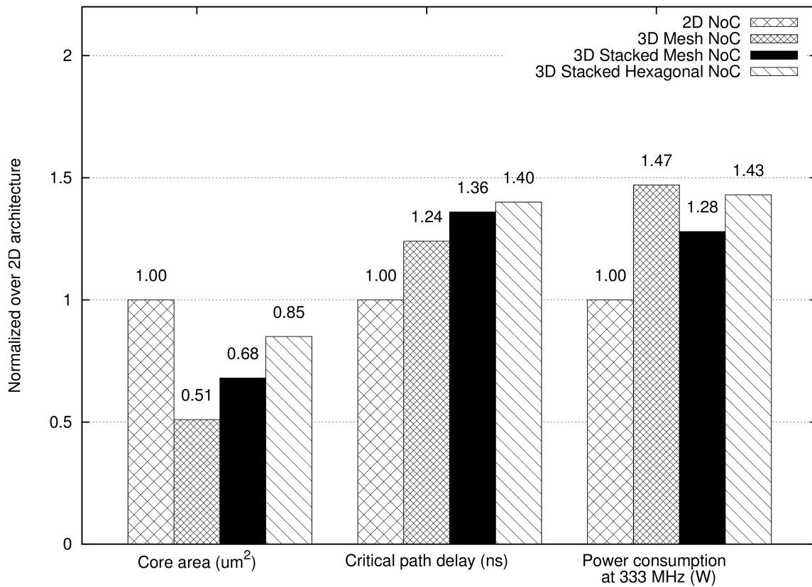
Figure 12: Comparaison des performances des architectures NoC 3D sur 2D NoC en 130 nm technologie
