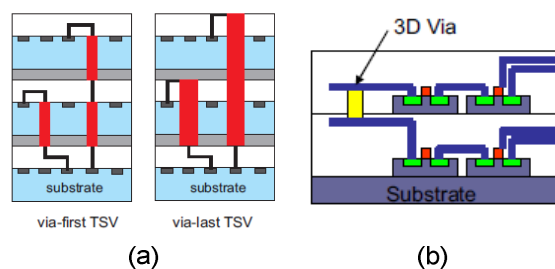
Figure 3: TSV méthodes d'empilage (A) par-premier-dernier et par l'intermédiaire d'CMOS en nombre (b) par l'intermédiaire de premier TSV-CMOS SOI dans [26]
