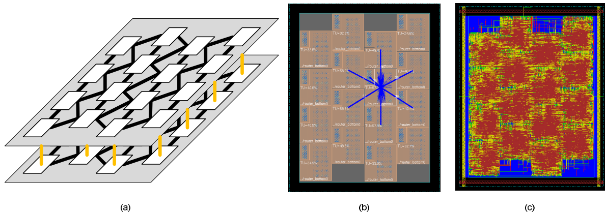
Figure 11: 3D Stacked Hexagonal NoC (a) diagramme (b) floorplan (c) mise en dérouté
