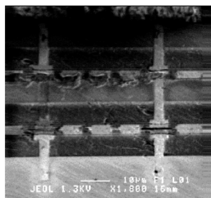
Figure 6: Tezzaron face-to-face superposition à l'aide de microbumps
