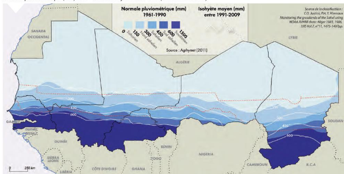
Normale pluviométrique (mm) 1961-1990 et isohyètes 1991-2009 (données mesurées)
