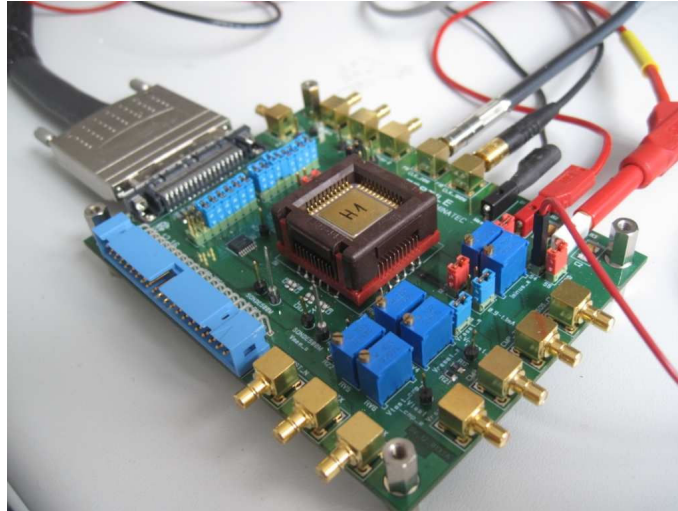
Figure II.31: Carte de caractérisation et circuit Reptile
