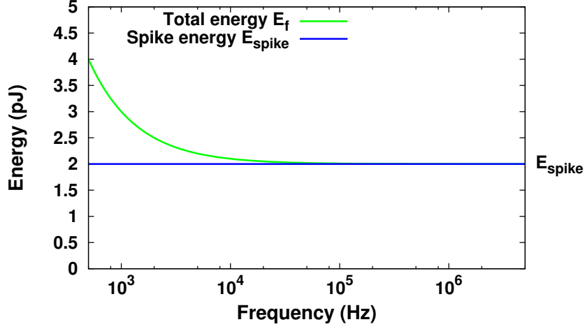
Figure II.24: E_f correspond à l'énergie dissipée pour la génération de potentiels d'action à une fréquence f . Elle inclue l'énergie nécessaire à l'émission du potentiel d'action (puissance active fonction de la fréquence) et la puissance statique. A partir de f = 50 \text{ kHz} , la dissipation d'énergie causée par les courants de fuite est négligeable pour considérer E_f = E_{spike}
