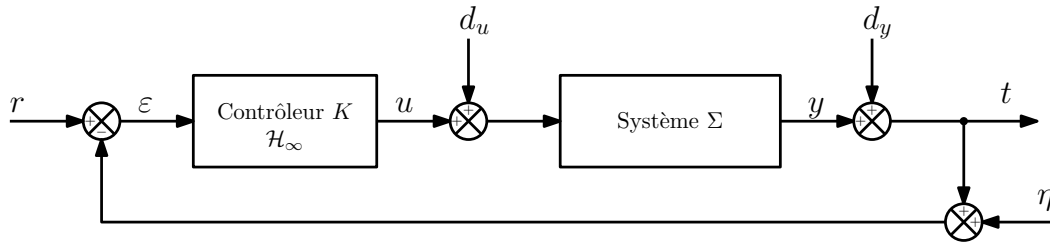
FIGURE II.3 – Schéma de l'interconnexion
