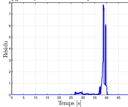
(d) Résidu pour v = 90km.h^{-1}
