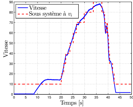
(a) Adaptation du résidu
