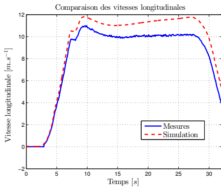
(c) Vitesse longitudinale
