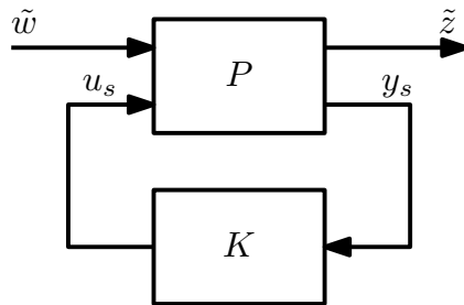
FIGURE II.7 – Problème sous forme standard
