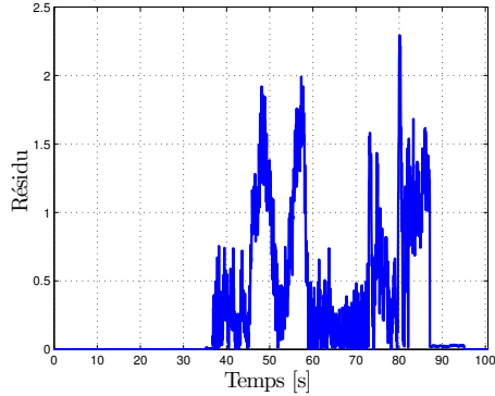
(b) Résidu pour v = 30km.h^{-1}
