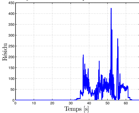
(c) Résidu pour v = 60km.h^{-1}
