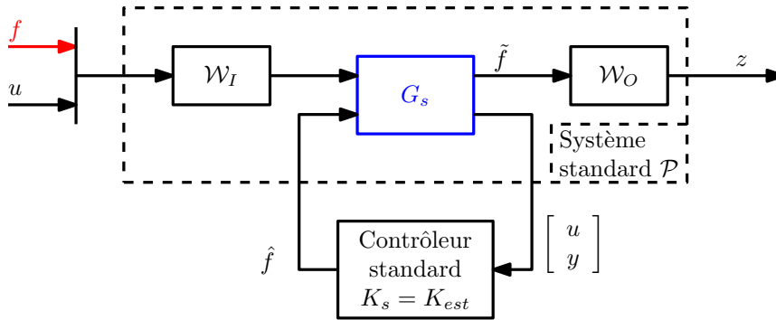
FIGURE II.9 – Principe de l’estimateur de défauts \mathcal{H}_\infty
