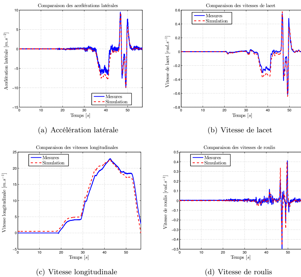
FIGURE III.18 – Comparaison des signaux réels et du simulateur pour v = 80km.h^{-1}
