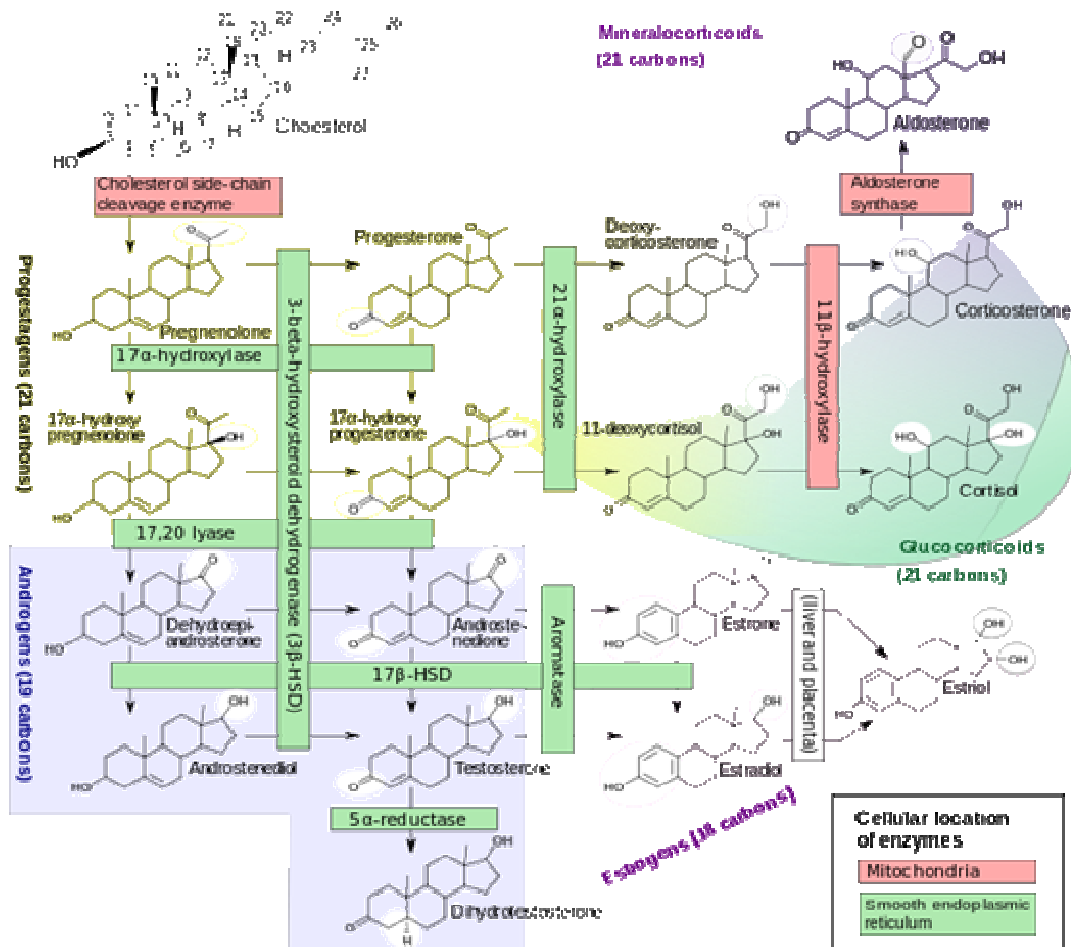
Figure 19 : Biosynthèse des hormones stéroïdes (Boron et Boulpaep, 2003).
