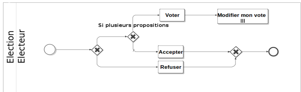
FIGURE 91: Le processus métier « Election »
