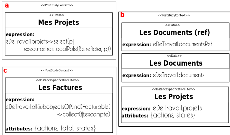
FIGURE 81: Les contextes de post-étude associés aux actions « Voir ET-Client » (a), « Voir ET-Developpeur » (b) et « Voir ET-Chef d'équipe » (c)
