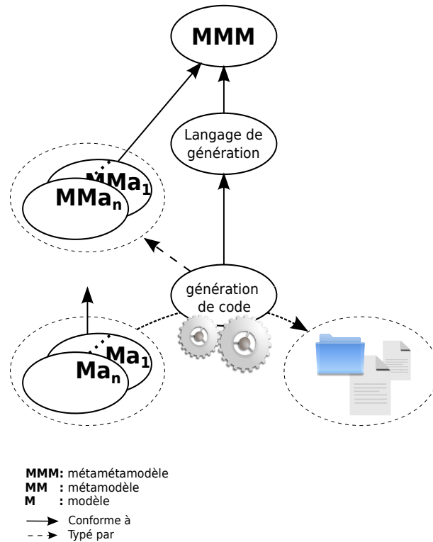
FIGURE 14: Relation entre les générations de code et les modèles (modèle, métamodelle et métamétamodelle)
