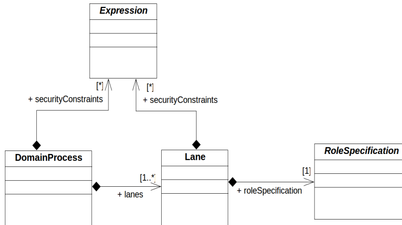
FIGURE 45: Une partie du métamodèle des processus métier
