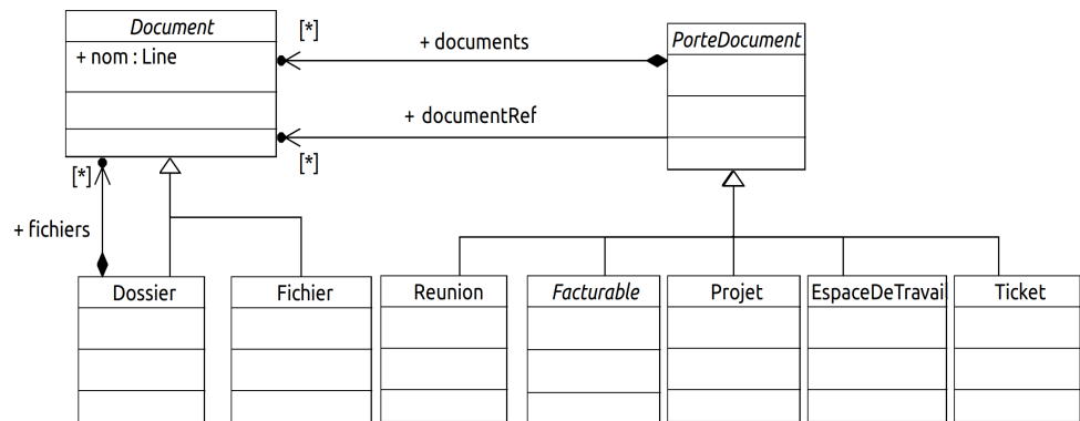
FIGURE 69: Modèle de la vue informationnelle « PorteDocument »
