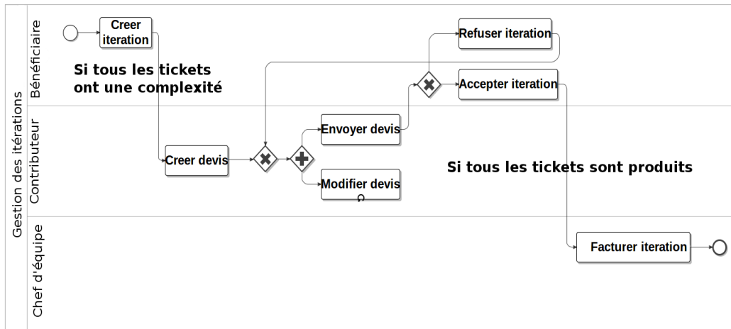
FIGURE 74: Le processus métier « Gestion des itérations »
