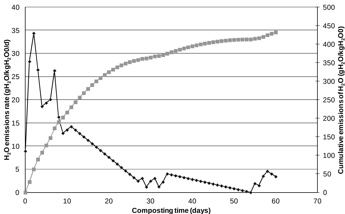
Figure 17. Cinétique d'émission d'eau (en gH 2 O kg -1 H 2 O 0 jr -1 ; en noir) et émissions cumulées (en gH 2 O kg -1 H 2 O 0 ; en gris) du tas CO_D
