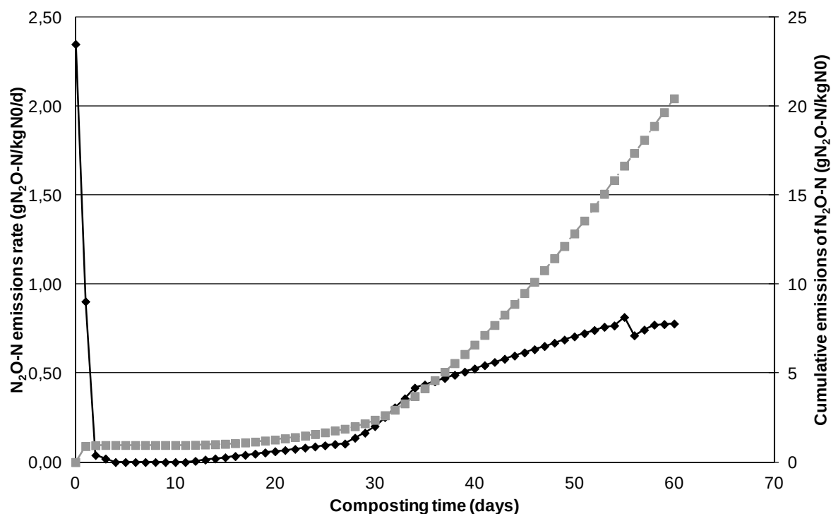
Figure 19. Cinétique d'émission de protoxyde d'azote (en gN-N_2O\ kg^{-1}\ N_0\ jr^{-1} ; en noir) et émissions cumulées (en gN-N_2O\ kg^{-1}\ N_0 ; en gris) du tas CO_D
