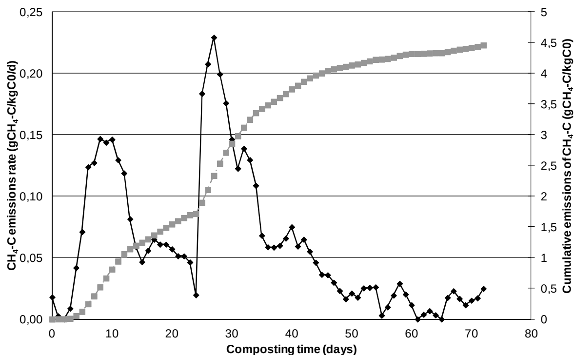
Figure 35. Cinétique d'émission de méthane (en gC-CH 4 kg -1 C 0 jr -1 ; en noir) et émissions cumulées (en gC-CH 4 kg -1 C 0 ; en gris) du tas CO_G
