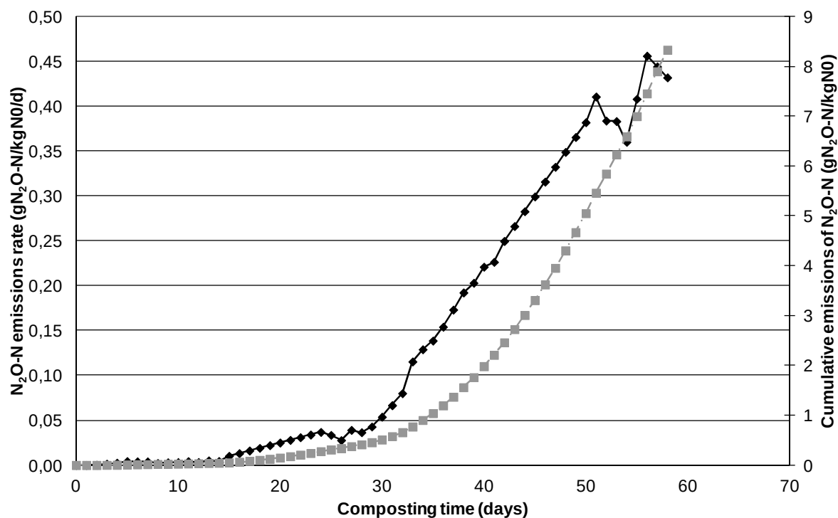
Figure 24. Cinétique d'émission de protoxyde d'azote (en gN-N 2 O kg -1 N 0 jr -1 ; en noir) et émissions cumulées (en gN-N 2 O kg -1 N 0 ; en gris) du tas CO_E
