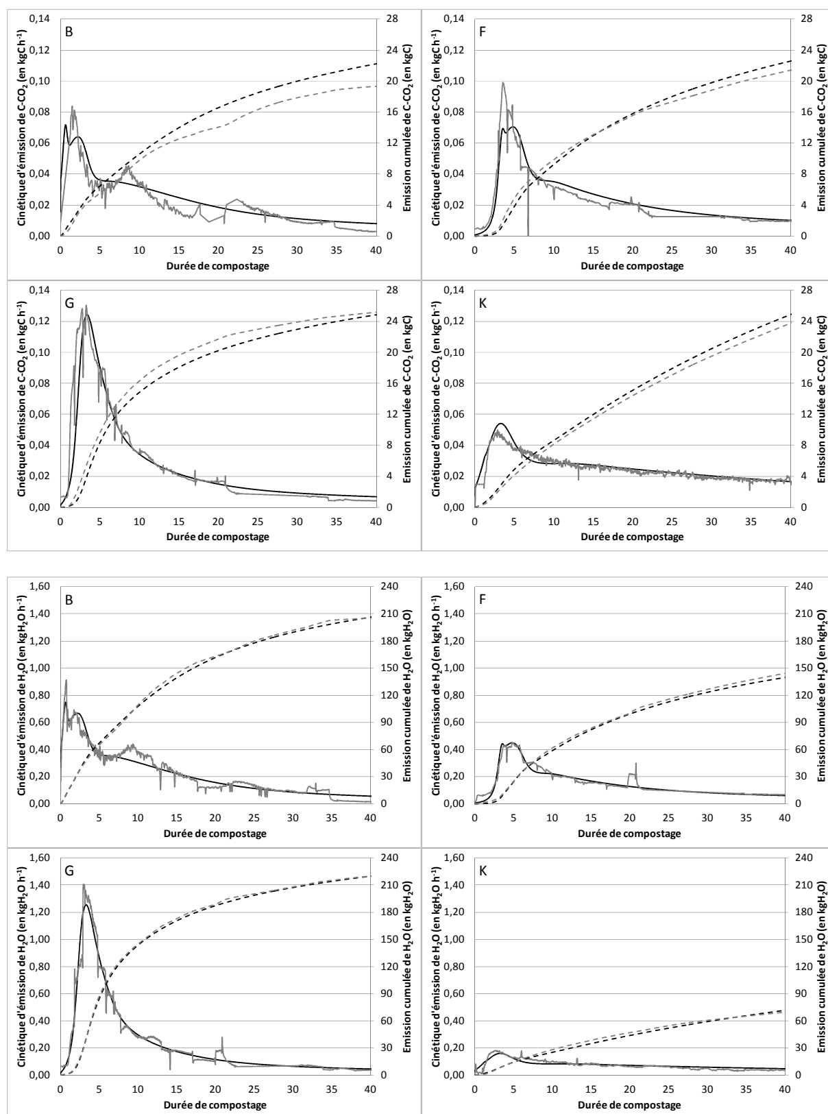
Figure 37. Comparaisons des cinétiques d'émissions simulées (noir), instantanées (trait plein) et cumulées (tirets) pour le dioxyde de carbone (haut) et la vapeur d'eau (bas)
