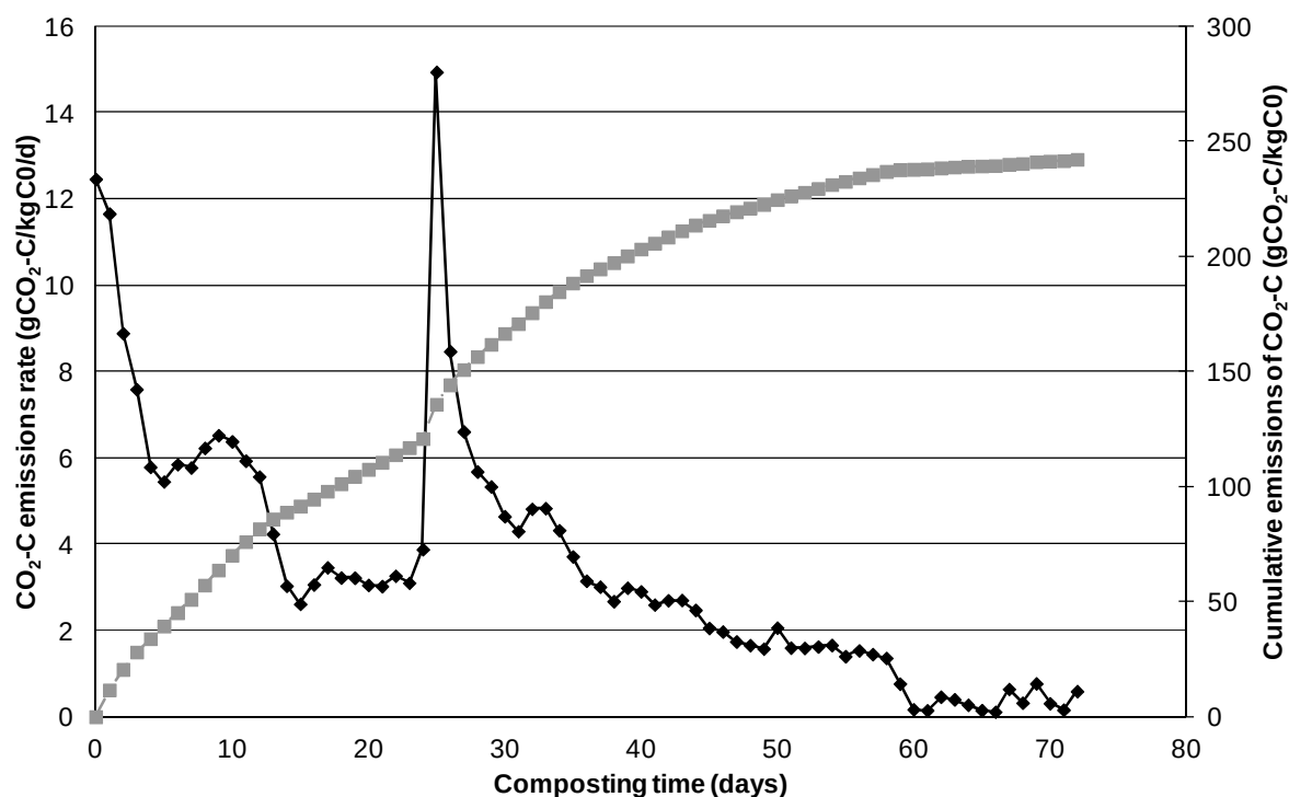
Figure 31. Cinétique d'émission de dioxyde de carbone (en gC-CO 2 kg -1 C 0 jr -1 ; en noir) et émissions cumulées (en gC-CO 2 kg -1 C 0 ; en gris) du tas CO_G
