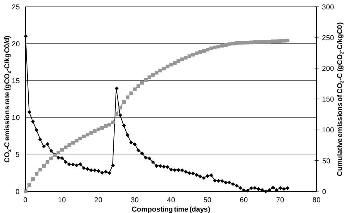
Figure 36. Cinétique d'émission de dioxyde de carbone (en gC-CO 2 kg -1 C 0 jr -1 ; en noir) et émissions cumulées (en gC-CO 2 kg -1 C 0 ; en gris) du tas CO_H
