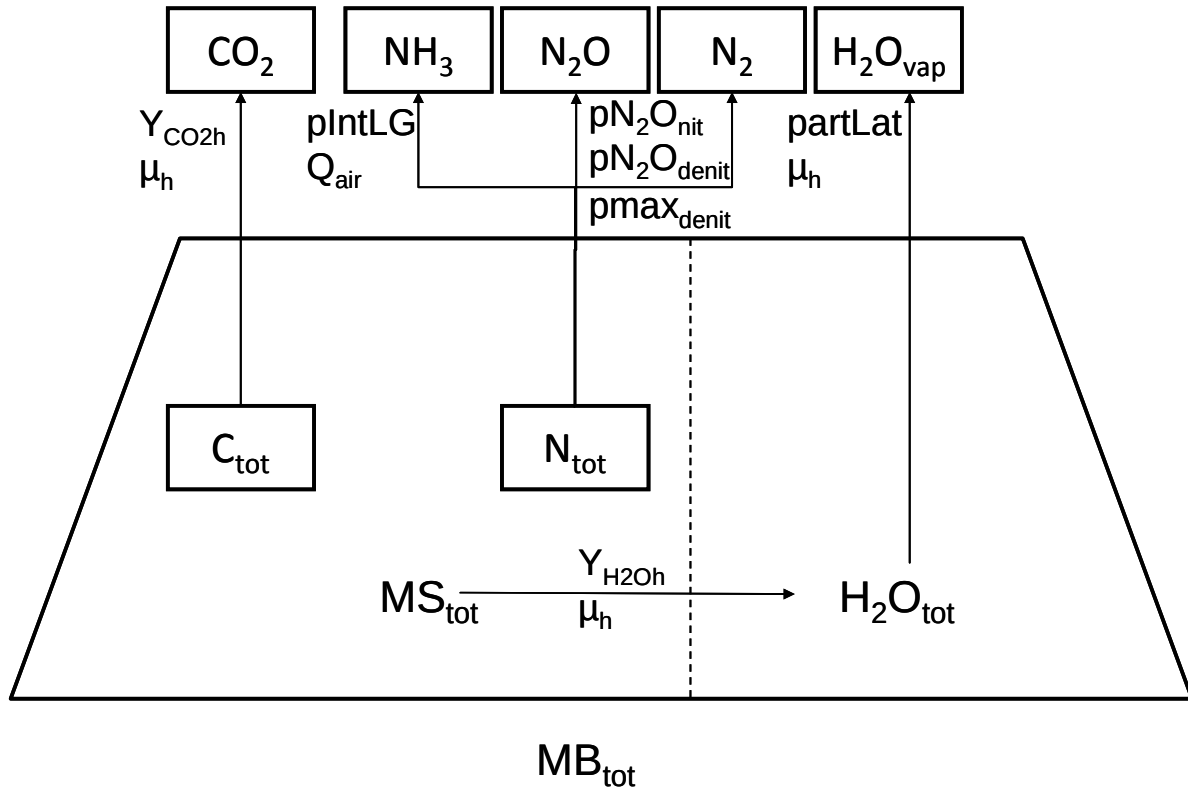
Figure 34. Représentation schématique du bilan massique d'un andain
