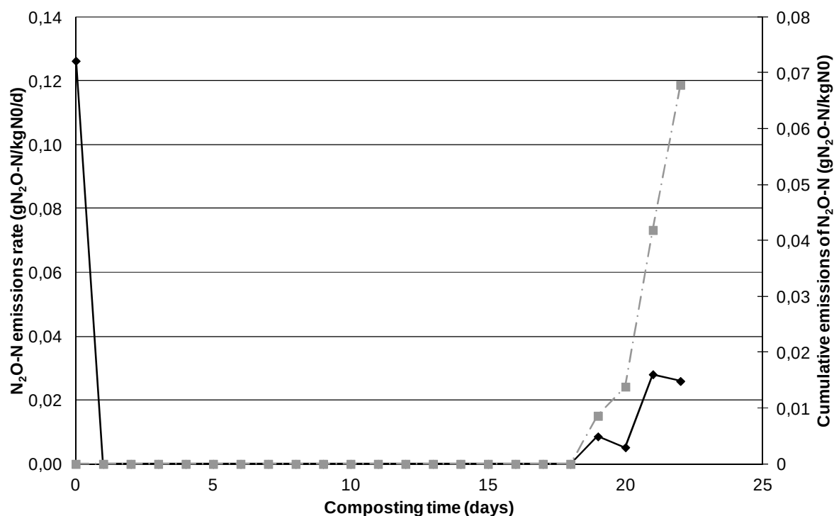
Figure 9. Cinétique d'émission de protoxyde d'azote (en gN-N_2O\ kg^{-1}\ N_0\ jr^{-1} ; en noir) et émissions cumulées (en gN-N_2O\ kg^{-1}\ N_0 ; en gris) du tas CO_B
