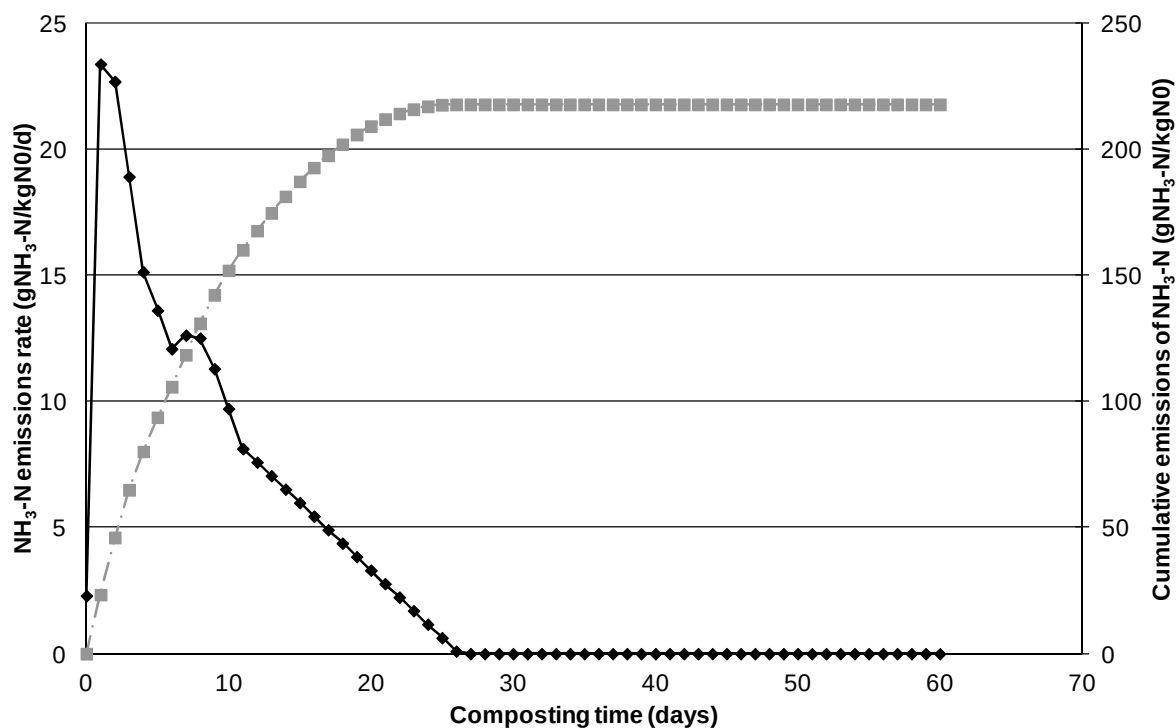
Figure 18. Cinétique d'émission d'ammoniac (en gN-NH 3 kg -1 N 0 jr -1 ; en noir) et émissions cumulées (en gN-NH 3 kg -1 N 0 ; en gris) du tas CO_D
