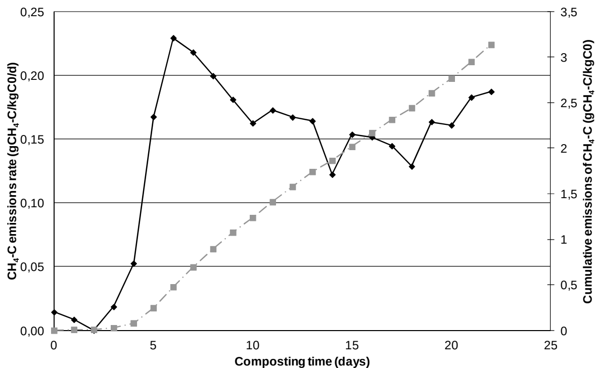
Figure 10. Cinétique d'émission de méthane (en gC-CH_4\ kg^{-1}\ C_0\ jr^{-1} ; en noir) et émissions cumulées (en gC-CH_4\ kg^{-1}\ C_0 ; en gris) du tas CO_B
