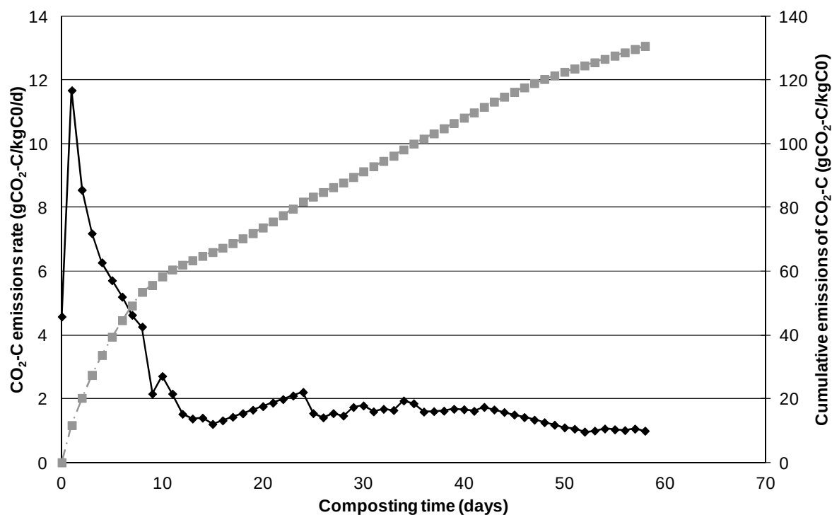
Figure 26. Cinétique d'émission de dioxyde de carbone (en gC-CO 2 kg -1 C 0 jr -1 ; en noir) et émissions cumulées (en gC-CO 2 kg -1 C 0 ; en gris) du tas CO_F
