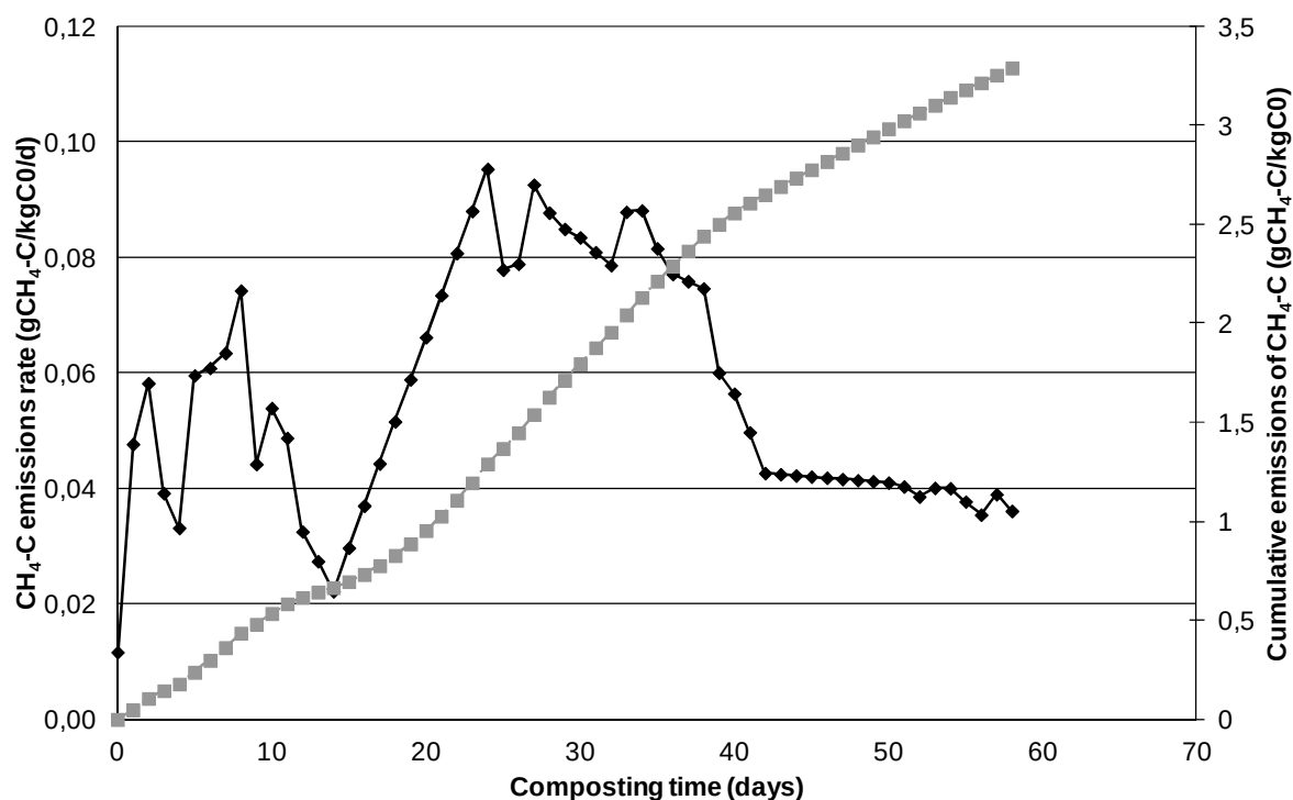
Figure 25. Cinétique d'émission de méthane (en gC-CH 4 kg -1 C 0 jr -1 ; en noir) et émissions cumulées (en gC-CH 4 kg -1 C 0 ; en gris) du tas CO_E
