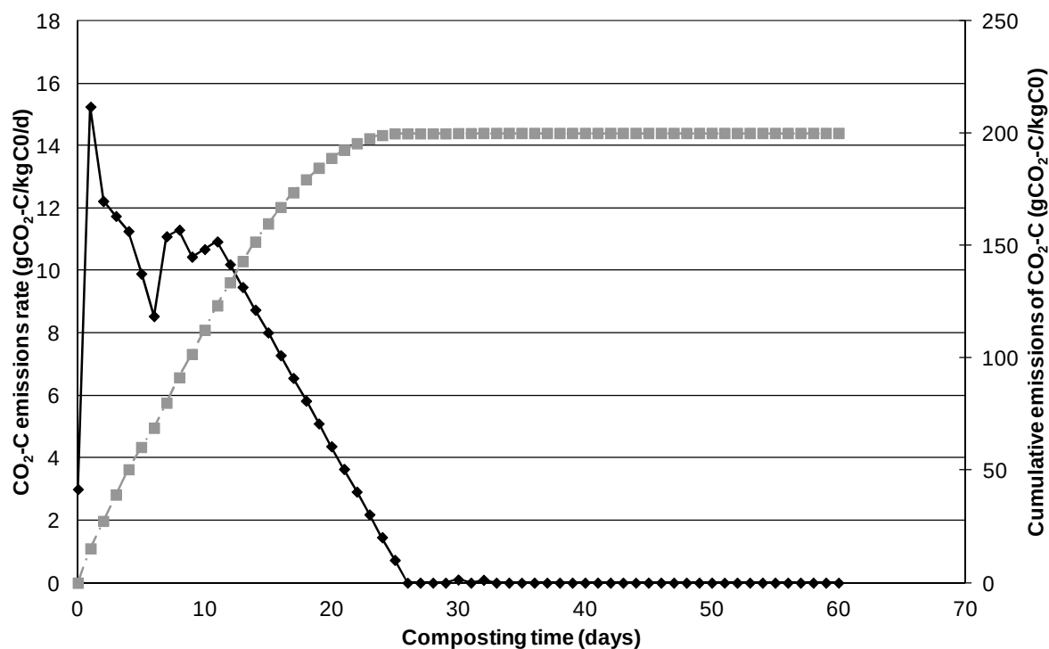
Figure 16. Cinétique d'émission de dioxyde de carbone (en gC-CO 2 kg -1 C 0 jr -1 ; en noir) et émissions cumulées (en gC-CO 2 kg -1 C 0 ; en gris) du tas CO_D
