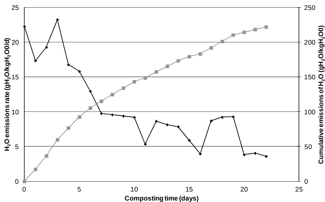
Figure 2. Cinétique d'émission d'eau (en \text{gH}_2\text{O kg}^{-1} \text{H}_2\text{O}_0 \text{ jr}^{-1} ; en noir) et émissions cumulées (en \text{gH}_2\text{O kg}^{-1} \text{H}_2\text{O}_0 ; en gris) du tas CO_A
