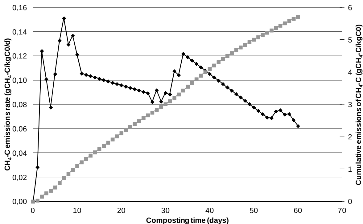
Figure 15. Cinétique d'émission de méthane (en gC-CH 4 kg -1 C 0 jr -1 ; en noir) et émissions cumulées (en gC-CH 4 kg -1 C 0 ; en gris) du tas CO_C
