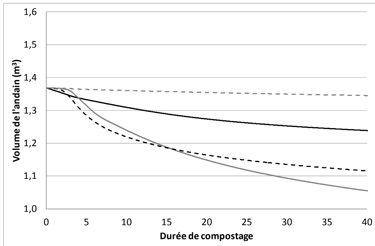
Figure 1. Simulation des évolutions du volume total des tas B (trait noir), F (trait gris), G (tirets noirs) et K (tirets gris)
