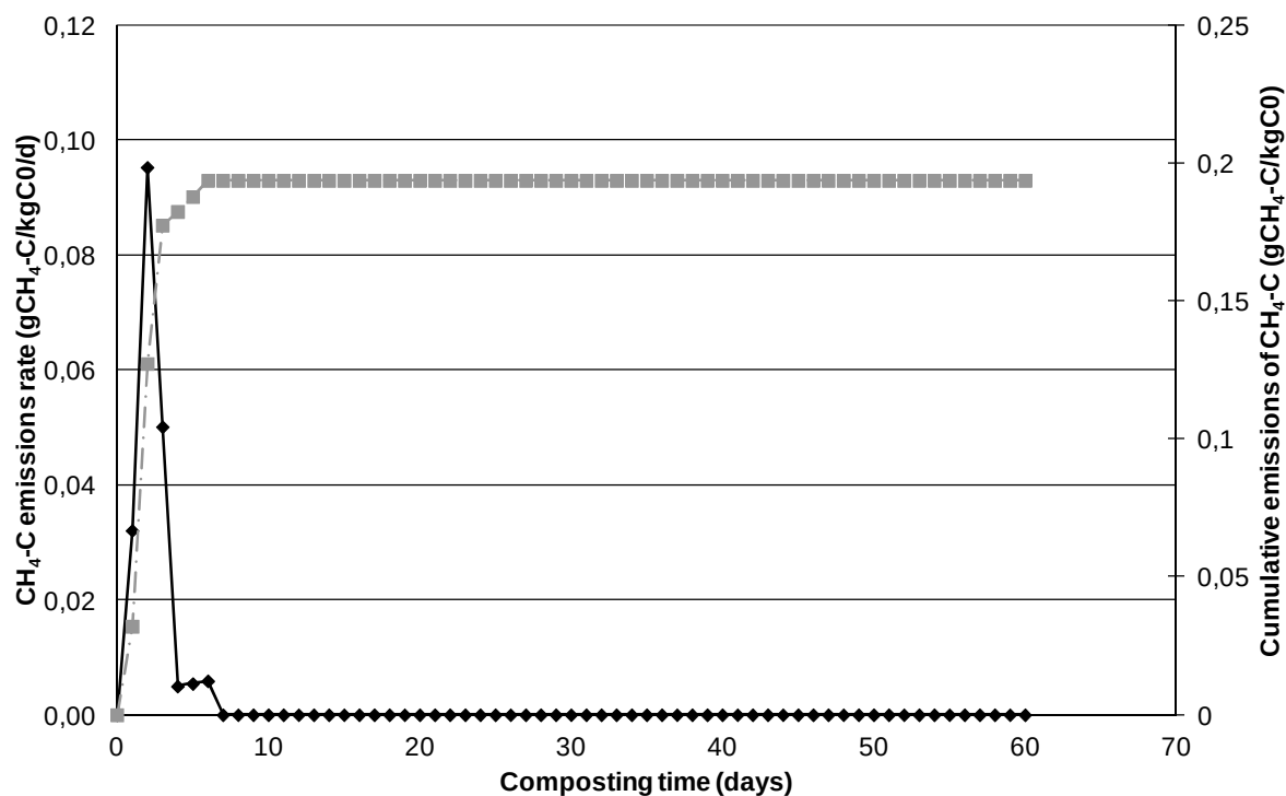
Figure 20. Cinétique d'émission de méthane (en gC-CH_4\ kg^{-1}\ C_0\ jr^{-1} ; en noir) et émissions cumulées (en gC-CH_4\ kg^{-1}\ C_0 ; en gris) du tas CO_D
