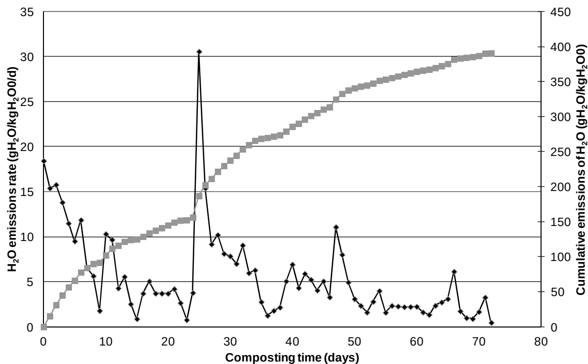
Figure 32. Cinétique d'émission d'eau (en gH 2 O kg -1 H 2 O 0 jr -1 ; en noir) et émissions cumulées (en gH 2 O kg -1 H 2 O 0 ; en gris) du tas CO_G
