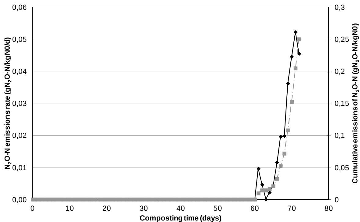
Figure 34. Cinétique d'émission de protoxyde d'azote (en \text{gN-N}_2\text{O} \text{ kg}^{-1} \text{ N}_0 \text{ jr}^{-1} ; en noir) et émissions cumulées (en \text{gN-N}_2\text{O} \text{ kg}^{-1} \text{ N}_0 ; en gris) du tas CO_G
