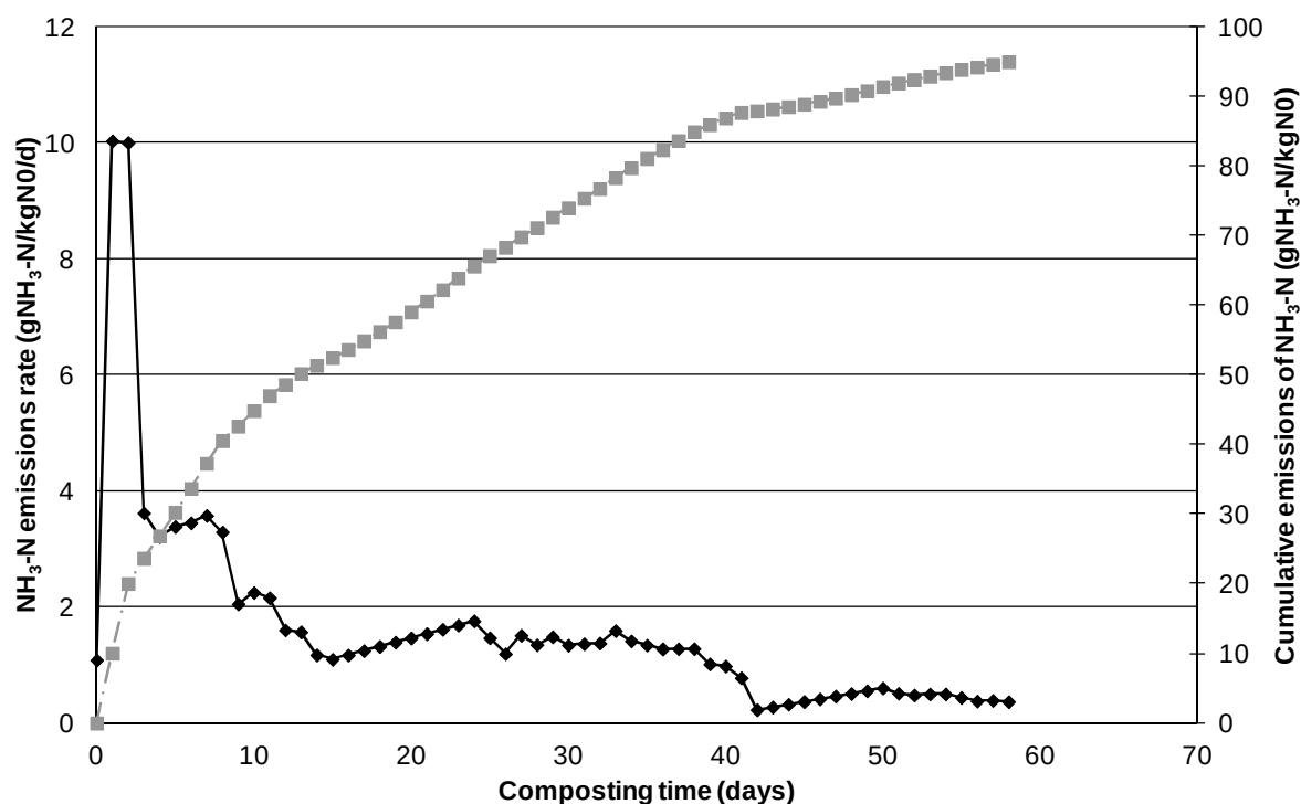
Figure 23. Cinétique d'émission d'ammoniac (en gN-NH 3 kg -1 N 0 jr -1 ; en noir) et émissions cumulées (en gN-NH 3 kg -1 N 0 ; en gris) du tas CO_E
