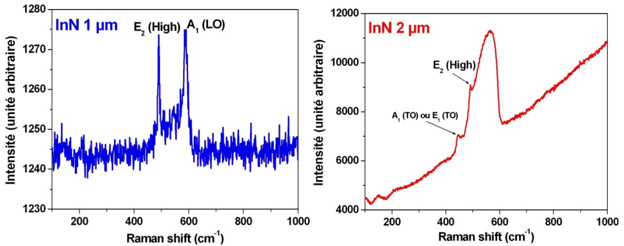
Figure II.8 : Spectres Raman d'échantillons d'InN issus des wafers de 1 μm et 2 μm d'épaisseur.
