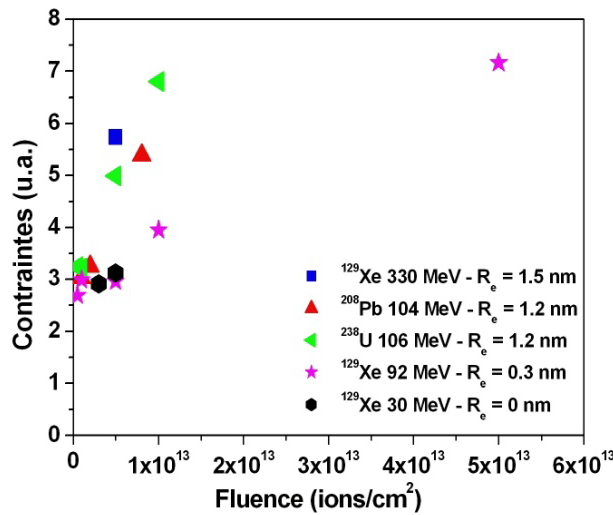
Figure IV.20 : Evolutions des contraintes biaxiales dans le plan de base du GaN en fonction de la fluence. Les rayons des traces produites par les différents ions sont indiqués.
