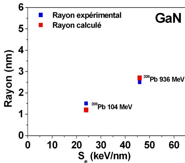
Figure IV.40 : Rayons expérimentaux et calculés par a-TS de traces produites par des projectiles ioniques dans le GaN.
