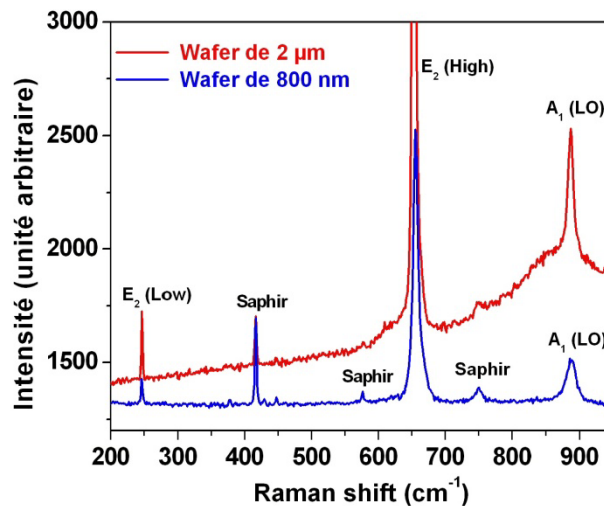
Figure II.4 : Spectres Raman d’échantillons d’AlN/Saphir issus des wafers 1 (800 nm) et 2 (2 \mu\text{m} ).
