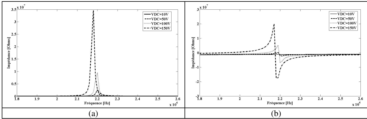
Figure.2. 27. Evolution de l'impédance d'entrée électrique en fonction de la fréquence pour différentes tensions continues appliquées pour une membrane CMUT ( 50\mu\text{m} , FF=0\% ) fonctionnant dans l'air (a) partie réelle (b) partie imaginaire.
