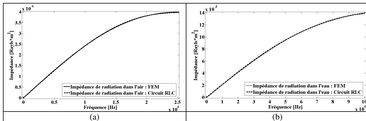
Figure.2. 23. Modélisation électrique en circuit RLC de l'impédance de radiation d'une membrane CMUT (50 \mu m, FF=0%) dans (a) l'air : ( R=3.96\mu\Omega , L=0.41pH , C=9.7mF ) (b) l'eau : ( R=14.5m\Omega , L=340.86pH , C=432.9nF ).
