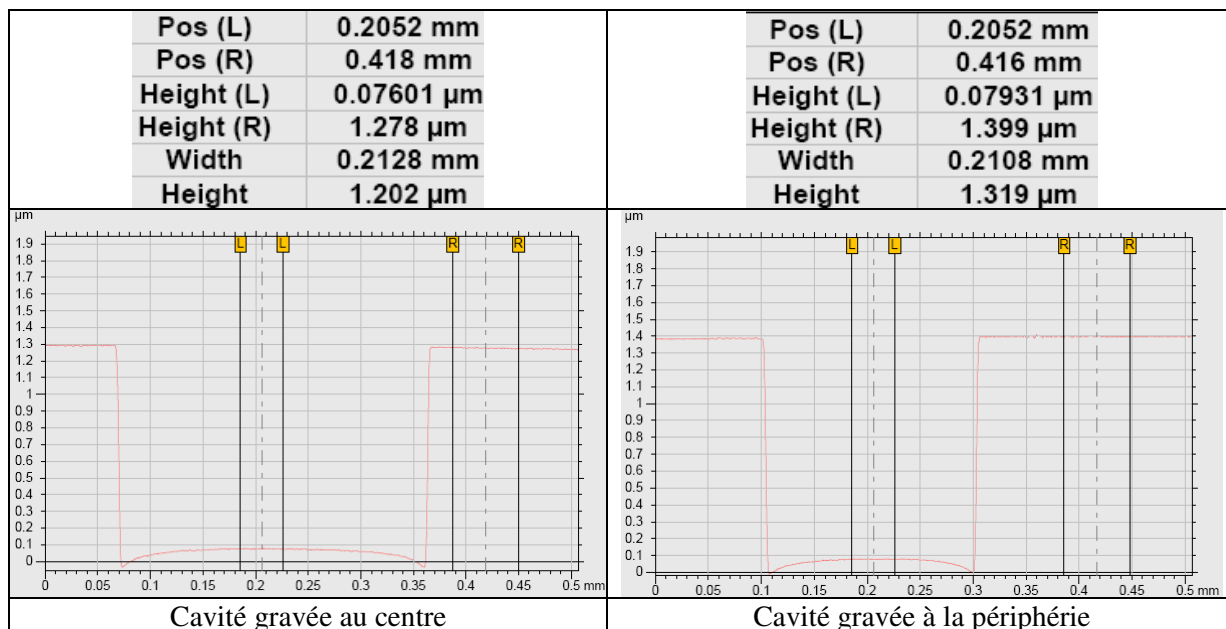
Figure.3. 9. Profils de gravure différents obtenus par gravure sèche DRIE.
