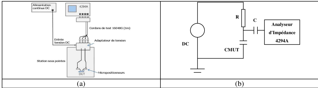
Figure.4. 17. (a) Banc de mesure utilisé pour la caractérisation électrique des dispositifs CMUTs. Le 16048G (1m de long) est un dispositif de fils de test 4-terminaux spécialement utilisé avec le 4294A (jusqu'à 110MHz) (b) Représentation schématique simplifiée de l'installation expérimentale de mesure.
