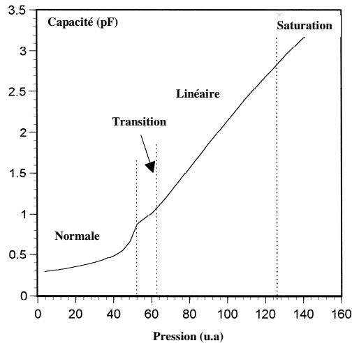
Figure.4. 22. Réponse caractéristique d'un capteur de pression capacitif en fonction de la pression appliquée sur la membrane [82].
