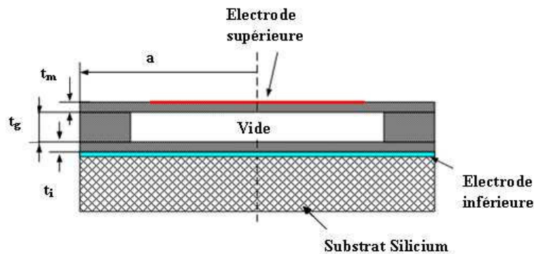
Figure.1. 1. Représentation schématique d'une cellule CMUT [1].
