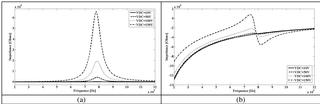
Figure.2. 28. Evolution de l'impédance d'entrée électrique en fonction de la fréquence pour différentes tensions continues appliquées pour une membrane CMUT ( 50\mu\text{m} , FF=0\% ) fonctionnant dans l'eau (a) partie réelle (b) partie imaginaire.
