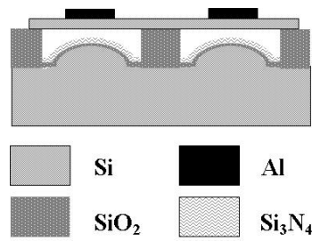
Figure.1. 17. Représentation schématique d'un LOCOS-CMUT [31].
