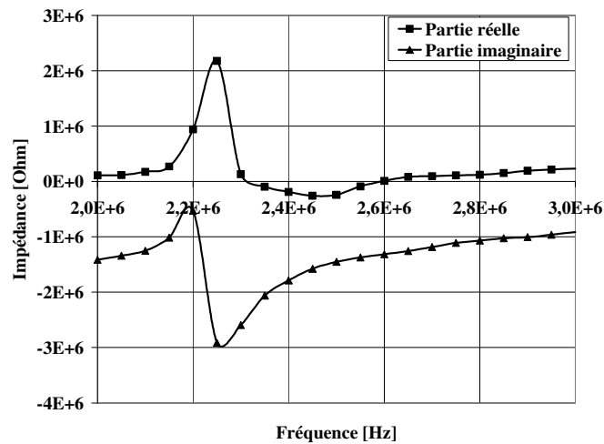
Figure.4. 19. Parties réelles et imaginaires de l’impédance électrique d’une cellule CMUT R=50\mu\text{m} et t_m=1.5\mu\text{m} pour une tension appliquée V_{DC}=80V .
