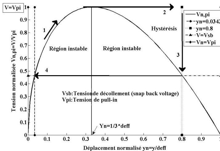
Figure.1. 8. Détermination de la tension de décolllement et apparition de l'hystérésis.
