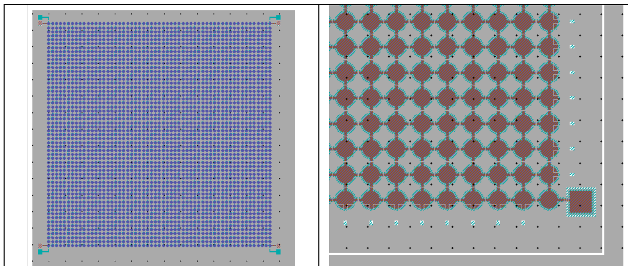
Figure.3. 6. Exemple d'un réseau de cellule de rayon 50µm avec une capacité de 200pF.
