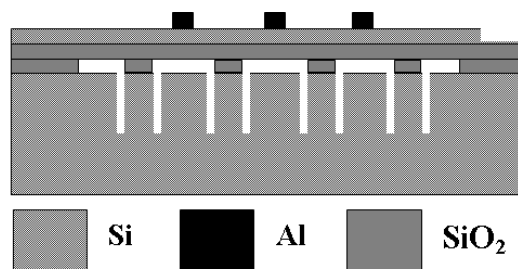
Figure.1. 18. Représentation schématique d'un CMUT à supports flexibles [48].
