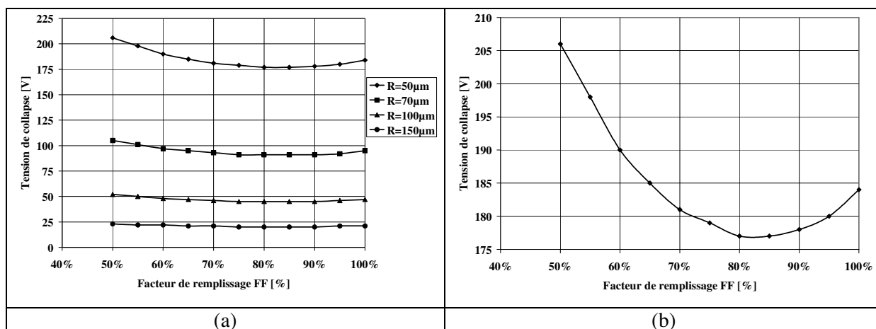
Figure.2. 3. Variations de la tension de collapse en fonction du facteur de forme de l'électrode supérieure pour (a) des rayons de membrane variant de 50µm à 150µm (b) une membrane de rayon 50µm.
