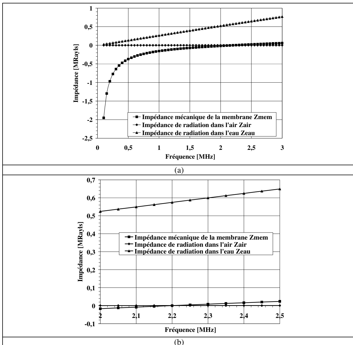
Figure.2. 22. Comparaison entre l'impédance mécanique et les impédances de rayonnement dans l'air et dans l'eau d'une membrane CMUT avec R=50\mu\text{m} (a) Vue globale (b) Vue agrandie autour de la fréquence de résonance de la membrane.
