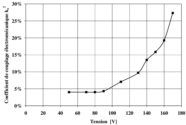
Figure.4. 24. Coefficient de couplage électromécanique mesuré pour une cellule unitaire R=50\mu\text{m} et t_m=1.5\mu\text{m} .
