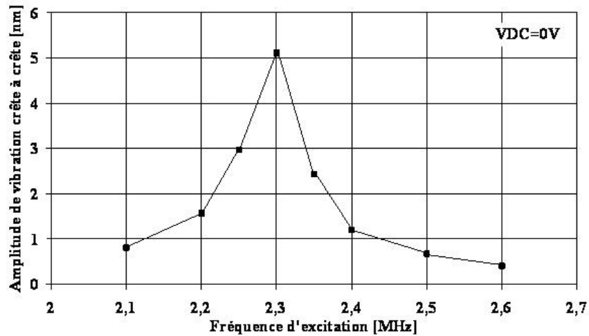
Figure.4. 12. Réponse fréquentielle obtenue par balayage fréquentiel pour une cellule unitaire. R=50\mu\text{m} et t_m=1.5\mu\text{m} .
