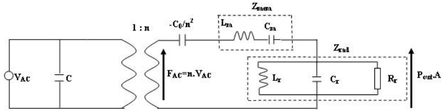
Figure.2. 24. Modèle en circuit équivalent d'une membrane CMUT ( 50\mu\text{m} , FF=0\% ), fonctionnant dans l'air ou dans l'eau.
