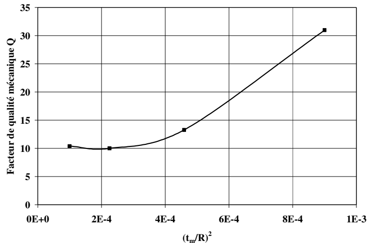
Figure.4. 13. Variation du facteur de qualité en fonction du rapport (t_m/R)^2 pour une membrane CMUT de rayon 50 \mu\text{m} et d'épaisseur t_m=1.5\mu\text{m} .
