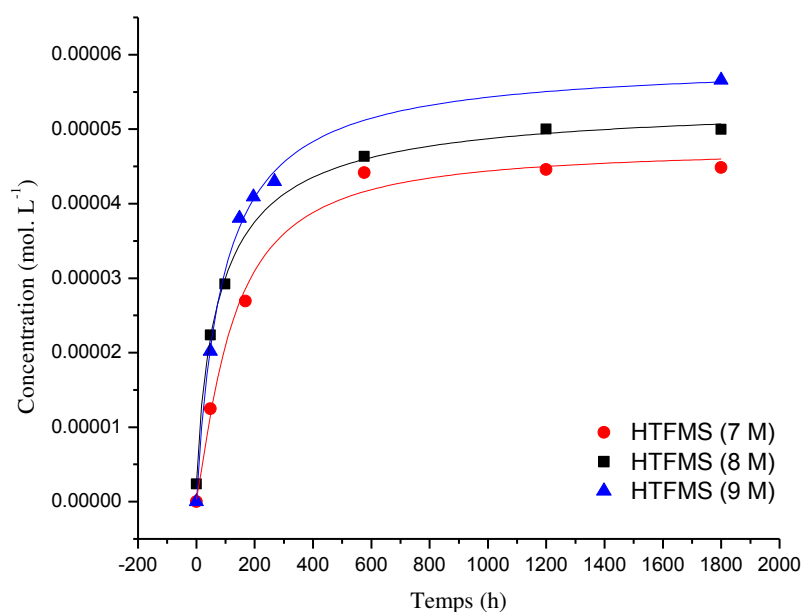
Figure III. 7. Courbes de formation de Tc(IV) polymère en fonction du temps.
