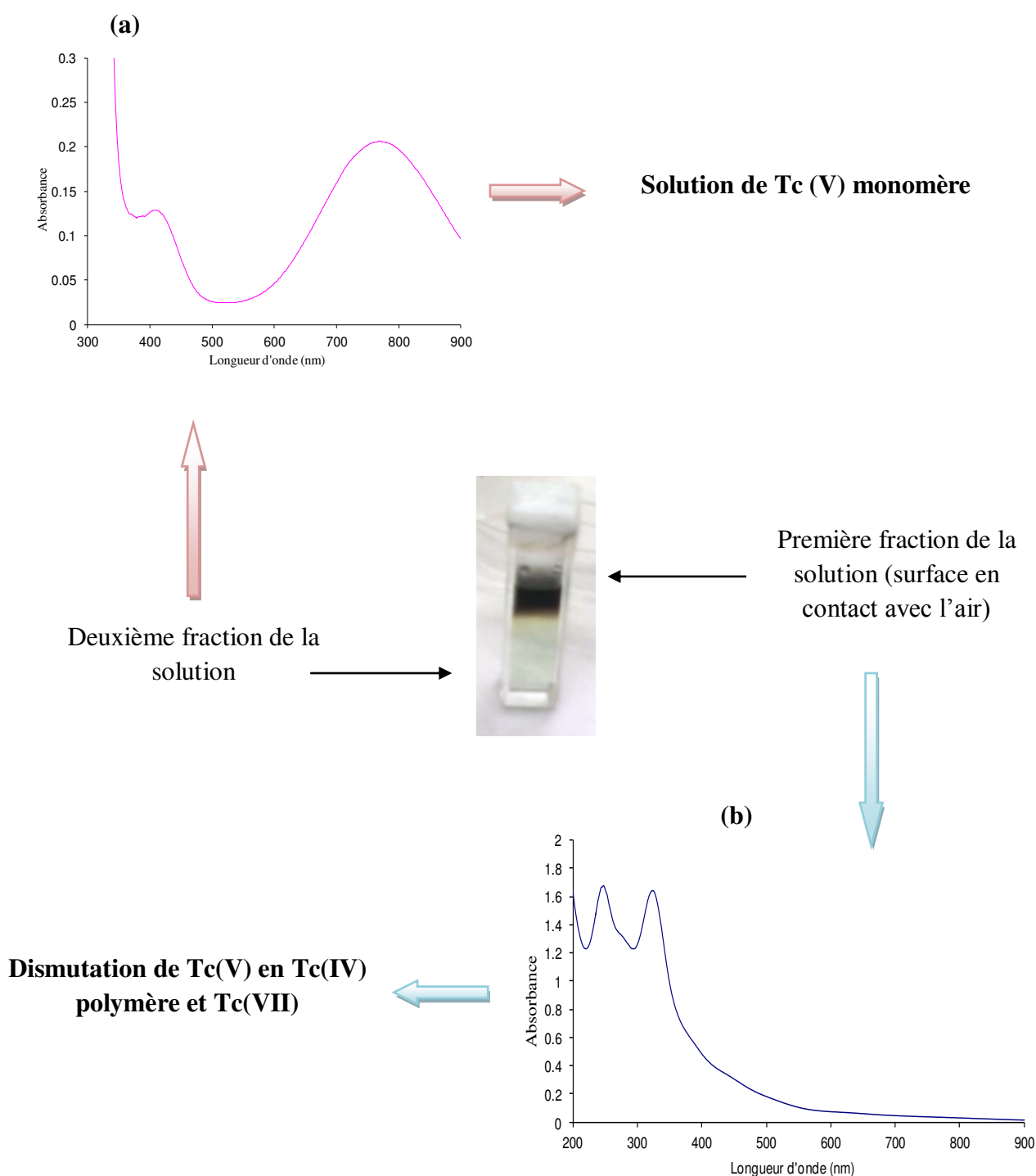
Figure V. 5. Changement de la couleur et du spectre UV-visible de la solution Tc ( 5,11 \times 10^{-3} M) barbotée avec \text{SO}_2(\text{g}) à la surface, (a) trajet optique = 1cm, (b) trajet optique = 1 mm.
