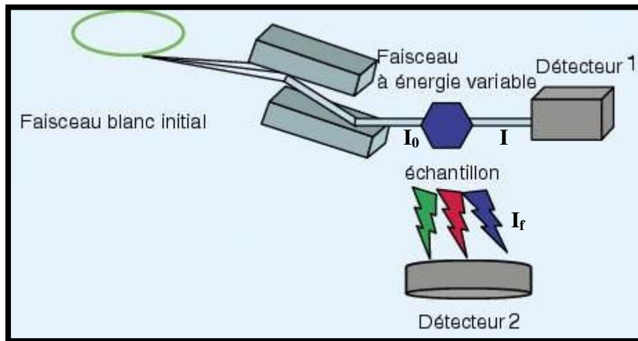
Figure II. 11. Montage simplifié de la chaîne d'expérimentation XAS en transmission (détecteur 1) et en détection de fluorescence (détecteur 2).
