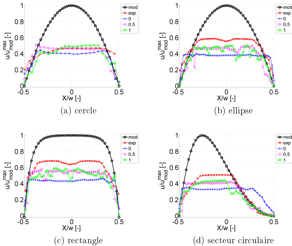
Figure H.14: Illustration de la distribution des vitesses normalisées transversales le long de la direction X : modélisées (mod), expérimentale (exp) et simulées (IB). Profils simulés sont présentés pour différentes positions de streamwise dans la constriction: à l'entrée ( Z/L_C = 0 ), au milieu ( Z/L_C = 0,5 ) et à la sortie ( Z/L_C = 1 ). Profils simulés instantanées sont évalués au temps t = 43\text{ms} pour la forme circulaire de rétrécissement et au temps t = 50\text{ms} pour les autres formes. La coordonnée X est normalisée par la largeur de la partie rétrécie w le long de la dimension X .
