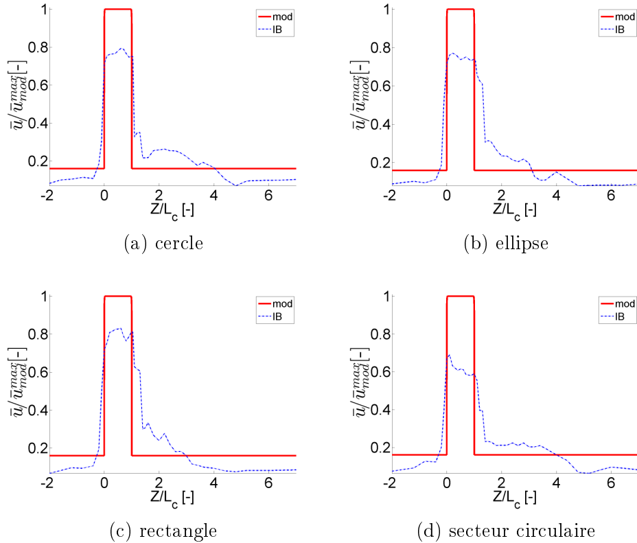
Figure H.13: Modélisé (mod) et simulé (IB) streamwise moyen ou distributions de vitesse locales sont normalisées par la vitesse local maximale modélisée \bar{u}_{mod}^{max} . Valeurs de vitesse modélisées correspondent à la vitesse apparente locale Q_{mod}/A(Z) avec Q_{mod} le débit de volume résultant du modèle quasi-tridimensionnel et A(Z) la streamwise variable la zone de canal. Pour la méthode de l'IB, les valeurs indiquées correspondent à la valeur moyenne transversale à chaque position par fractions Z . Valeurs simulées instantanées sont évalués au temps t = 43\text{ms} pour la forme circulaire de rétrécissement et au temps t = 50\text{ms} pour les autres formes de constriction.
