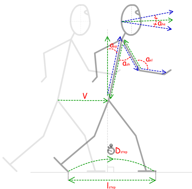
Figure 2.8 – Paramètres ségmentaires
