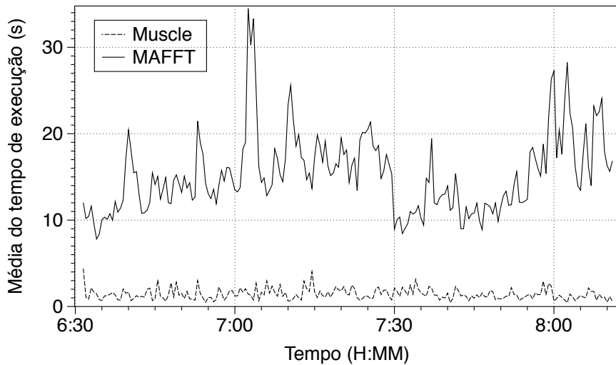
Figura 27. Tempo de execução médio das tarefas do Muscle versus MAFFT.
