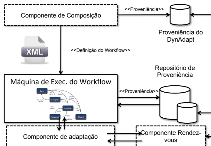
Figura 15. Arquitetura do DynAdapt.
