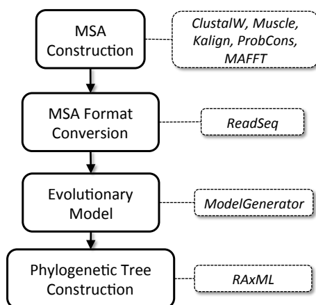
Figura 19. Workflow SciPhy como definido em Ocaña et. al. (2011b)
