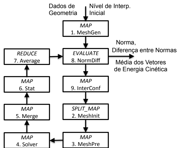
Figura 24. Workflow de QI iterativo (e dinâmico).
