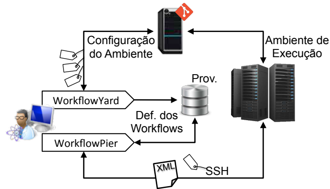
Figura 14. Funcionamento dos módulos de composição e disparo do workflow.
