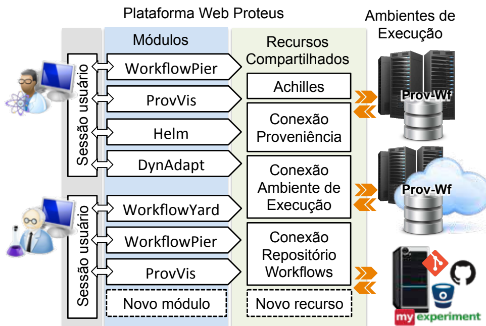
Figura 13. Estrutura da plataforma Proteus.
