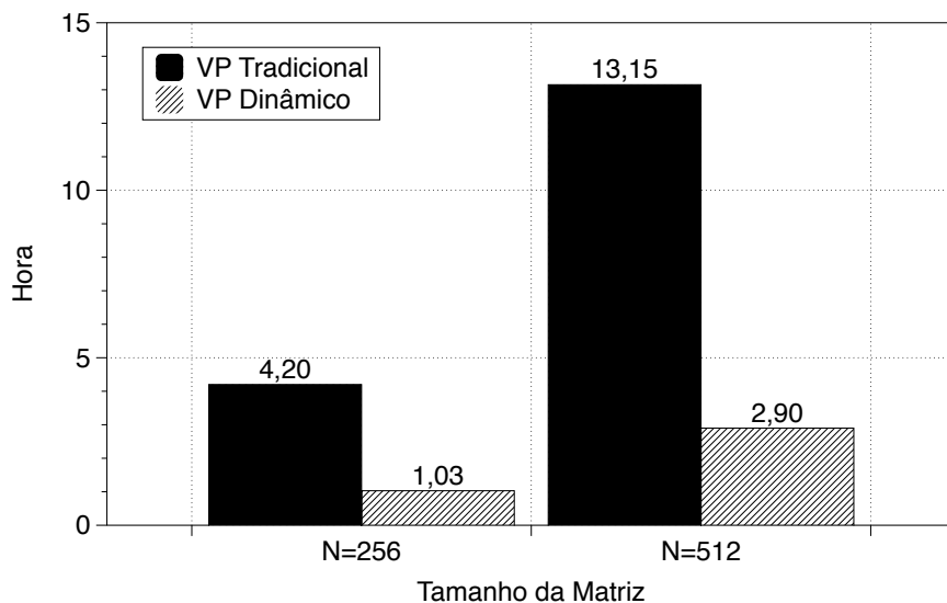
Figura 25. Economia do tempo de execução ao realizar interações com o workflow.
