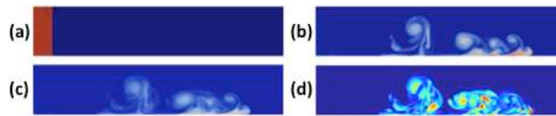
Figura 22. (a) Condição inicial heterogênea; (b) evolução da concentração; (c) média da concentração e (d) desvio padrão da concentração no final da execução.
