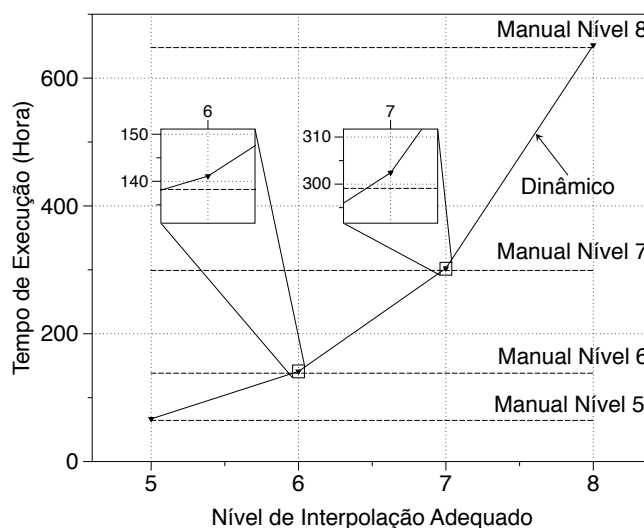
Figura 31. Eficiência da abordagem dinâmica comparada com a abordagem manual.
