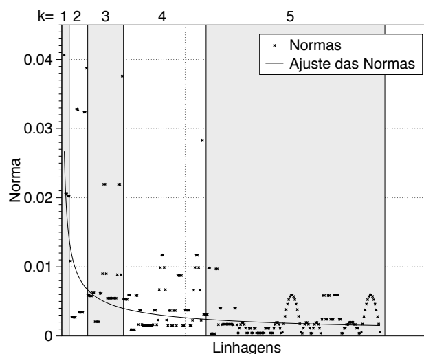
Figura 33. Valores das normas dos vetores para todas as linhagens do experimento.
