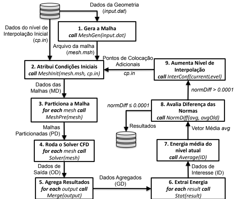
Figura 21. Workflow conceitual de Quantificação de Incertezas.
