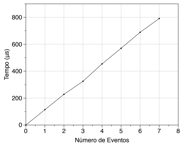
Figura 35. Desempenho do algoritmo Interação-Ômega.
