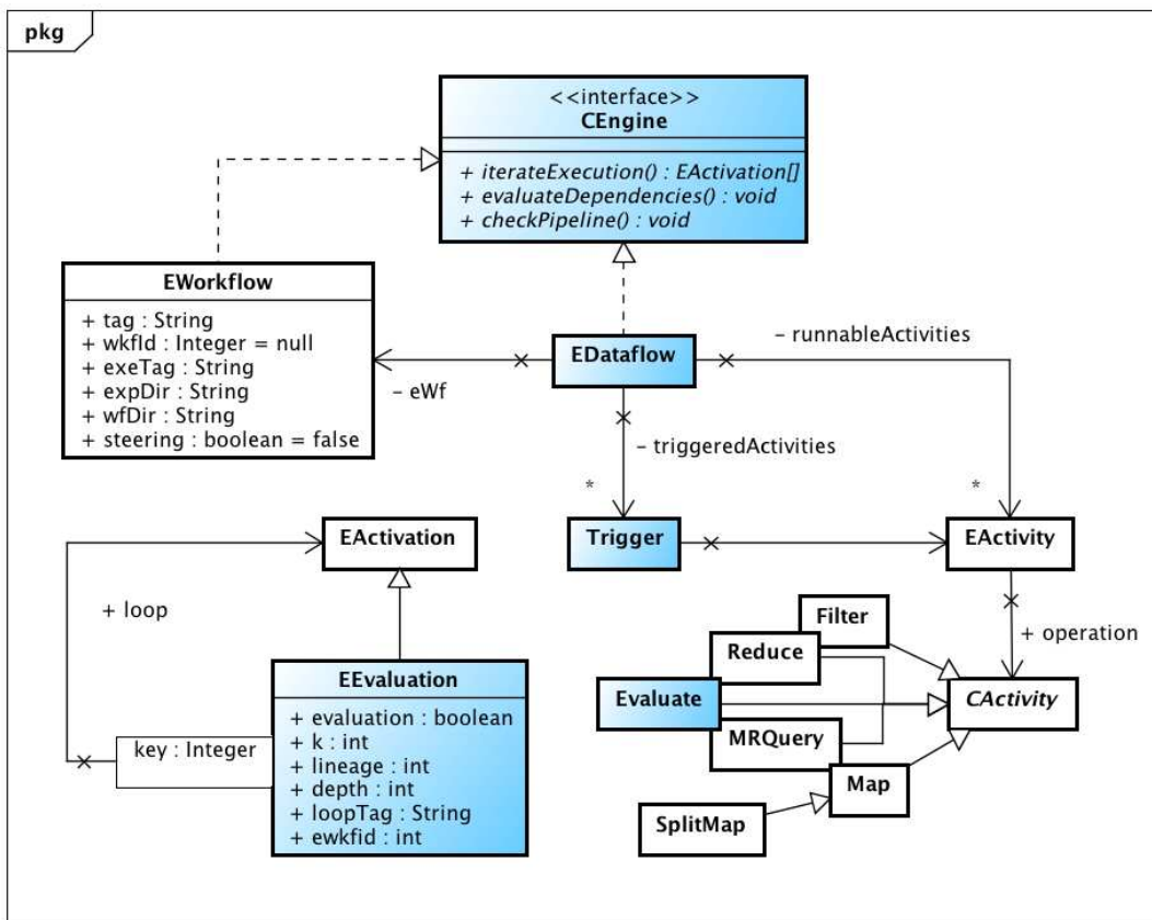
Figura 11. Diagrama simplificado de classes do Chiron com novas classes para ciclos dinâmicos destacadas em azul.
