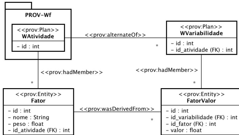
Figura 16. Fragmento da proveniência do DynAdapt.
