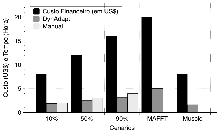
Figura 29. Comparação de tempo de execução e custo financeiro.
