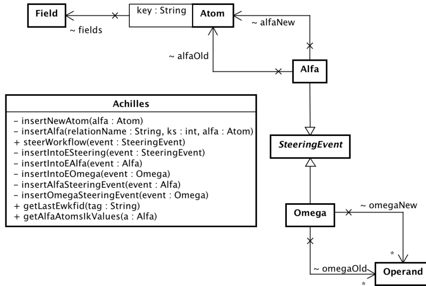
Figura 17. Diagrama de classes UML da API Achilles.
