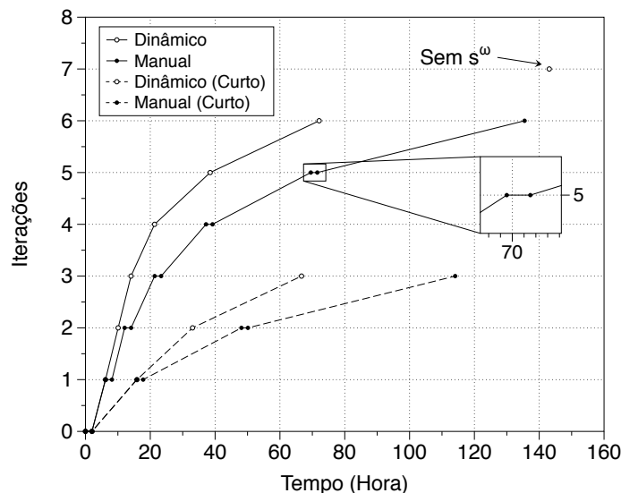
Figura 30. Tempo de execução das abordagens manual e dinâmica.
