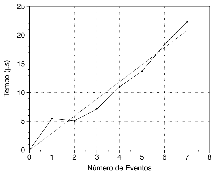
Figura 34. Desempenho do algoritmo Interação-Alfa.
