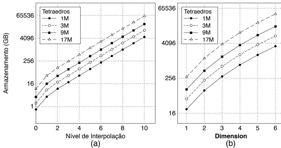
Figura 20. Crescimento do volume de dados em função do (a) nível de interpolação e da (b) dimensão do problema.
