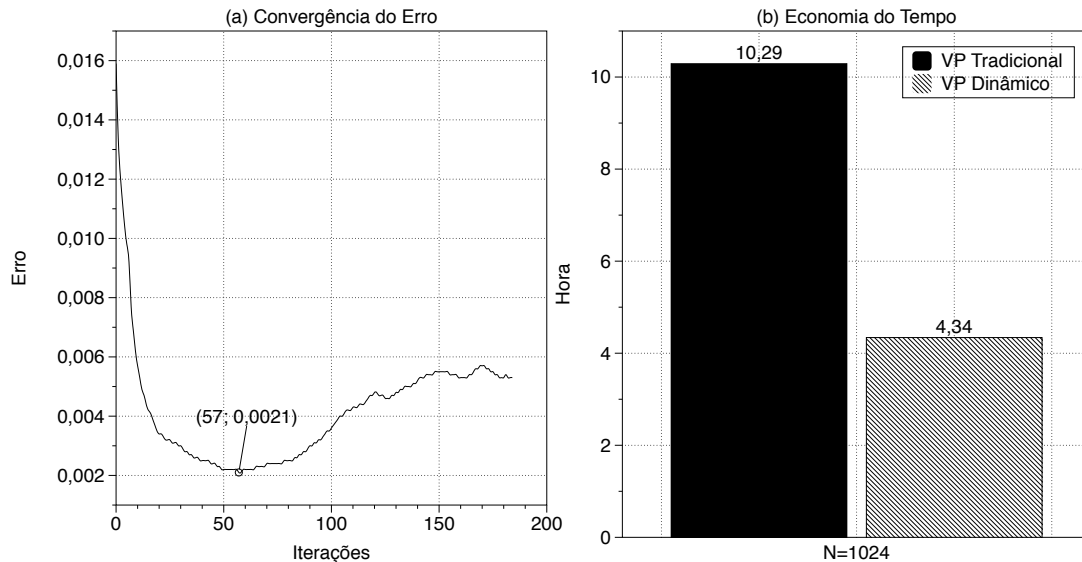
Figura 26. (a) Convergência do erro no segundo estudo e (b) o tempo economizado com o processo iterativo.
