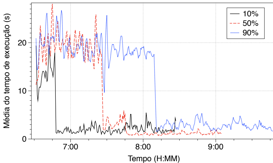
Figura 28. Mudanças dinâmicas no SciPhy.
