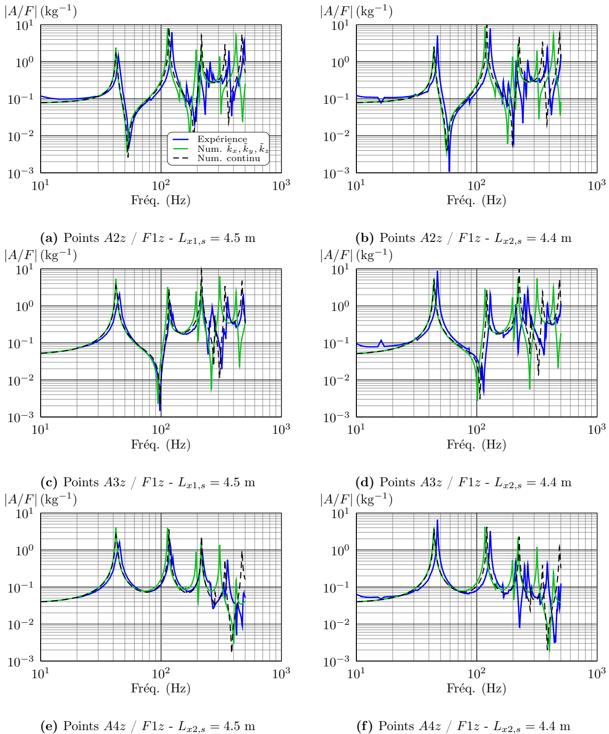
FIGURE B.9 – Réponse en fréquence \left| \frac{A}{F} \right| selon la direction de l'effort suivant \vec{x} du modèle numérique et expérimental - Test sur l'assemblage aux points F1z - A2z, A3z et A4z et selon deux longueurs de solive L_{x1,s} = 4.5 m et L_{x2,s} = 4.4 m.
