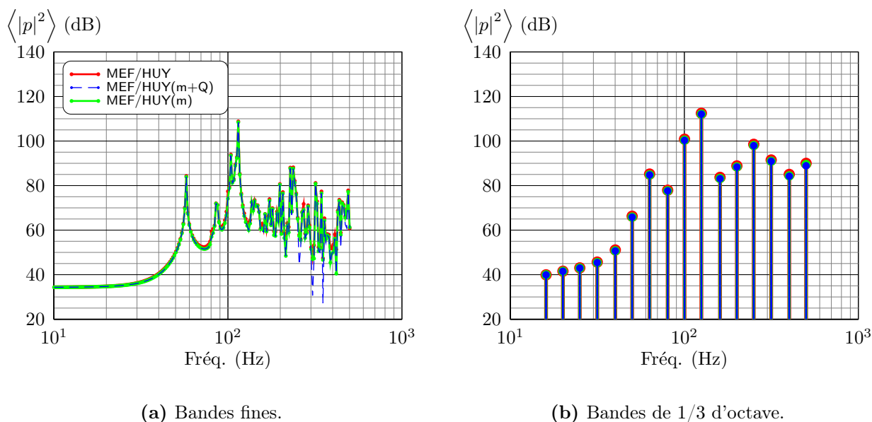
FIGURE 2.23 – Comparaison des pressions quadratiques moyennes issues du calcul par formulation intégrale initiale MEF/HUY et selon deux formulations réduites MEF/HUY(m) et MEF/HUY(m+Q).
