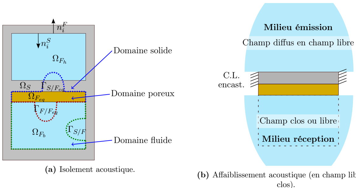
FIGURE 2.1 – Différents domaines et interfaces dans le calcul vibro-acoustique en acoustique du bâtiment.
