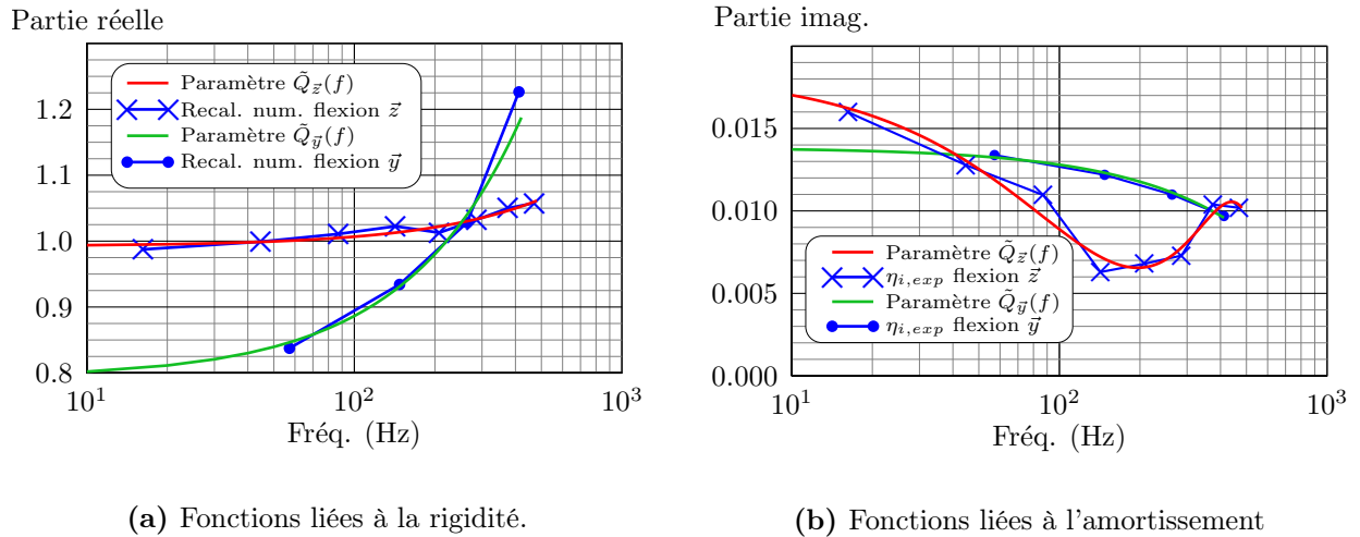
FIGURE 3.28 – Comparaison des deux paramètres de recalage \tilde{Q}_y(f) et \tilde{Q}_z(f) en fonction de la fréquence (recalage numérique effectué sur modes de flexion de la solive selon les directions \vec{y} et \vec{z} ).
