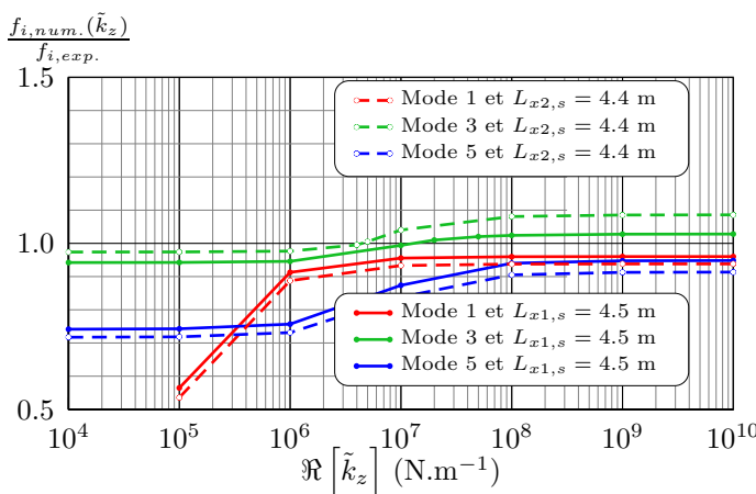
(a) Ratio des fréquences propres numériques et expérimentales en fonction de la raideur \tilde{k}_z du modèle numérique.
