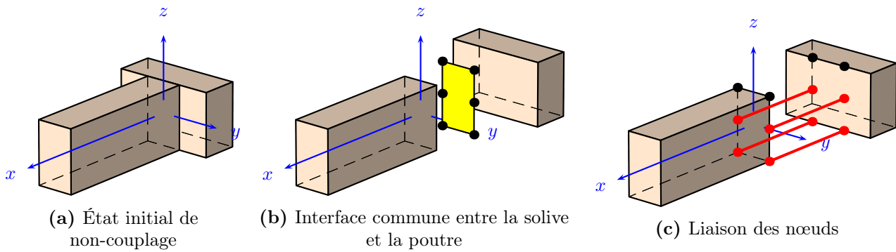
FIGURE 4.3 – Identification des nœuds pour le couplage structurel dans le maillage de la solive et de la poutre.
