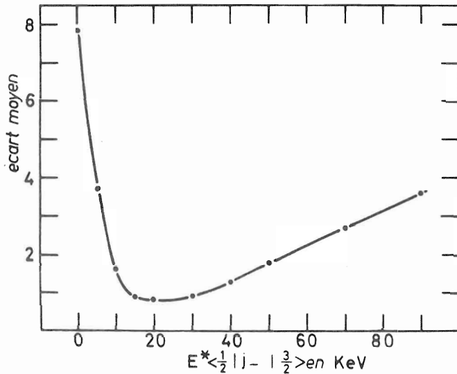
Fig. IV.14 - \frac{B(M1) - B(M1)_{calc.}}{\Delta B(M1)} \cdot \frac{1}{N}
