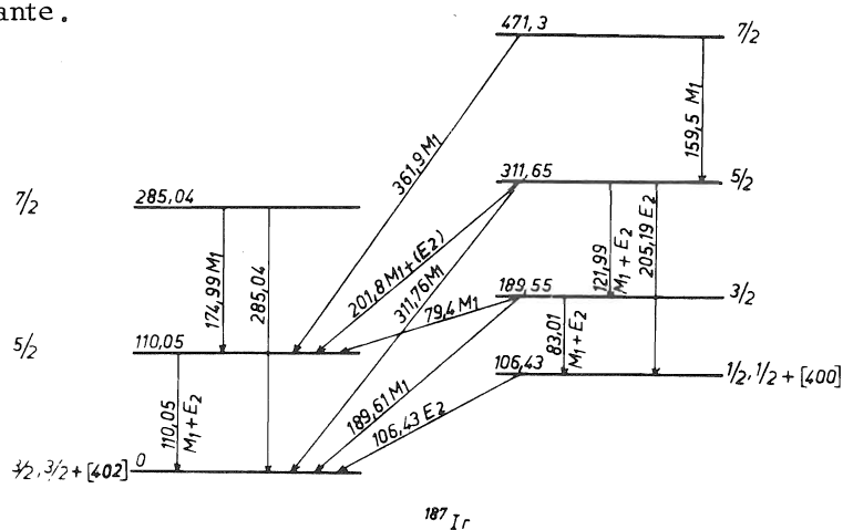
Fig. IV.12 - Niveaux de parité positive de basse énergie.
