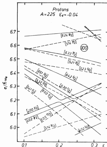
Fig. I.2 - Etats de protons A = 225 .
