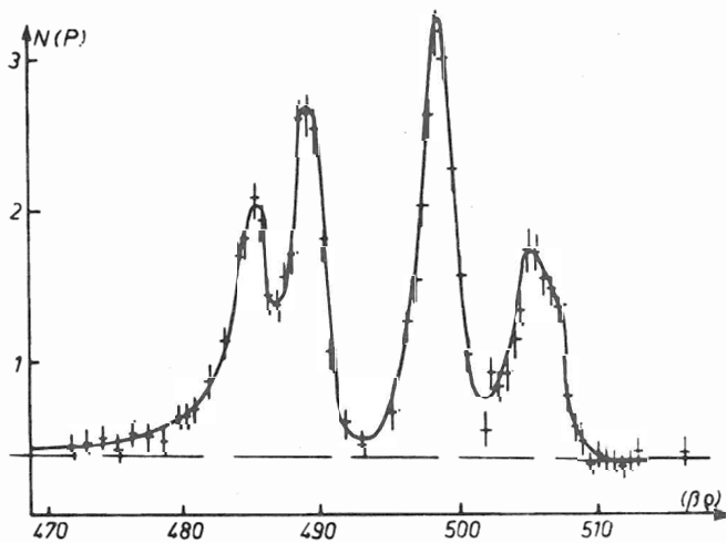
Fig. III.6 - Comparaison des groupes M de deux transitions E1 retardées \frac{5}{2} \frac{3}{2} + [651] - \frac{7}{2} \frac{1}{2} - [530] dans ^{231}\text{Pa} et ^{233}\text{Pa} .
