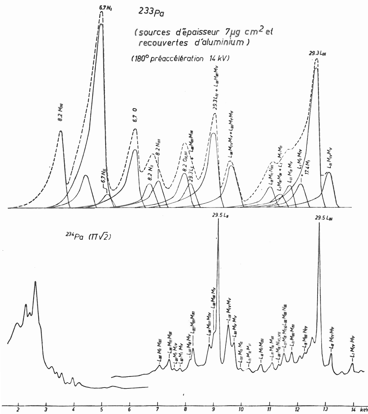
Fig. III.4 - Comparaison des spectres Auger L du ^{233}\text{Pa} et du ^{234}\text{Pa} .
