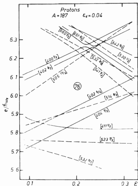
Fig. I.1 - Etats de protons A = 187 .
