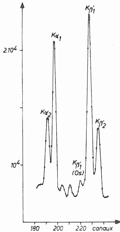
Fig. IV .9 - 187 Pt - 187 Ir Groupe XK
