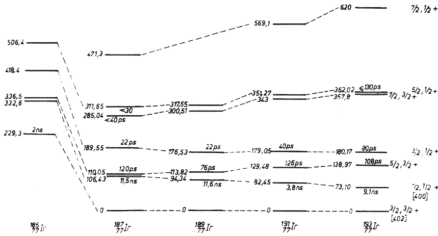
Fig. IV.11 - Les bandes de rotation \frac{3}{2}^+(402) et \frac{1}{2}^+(400) dans les iridium de masse impaire.
