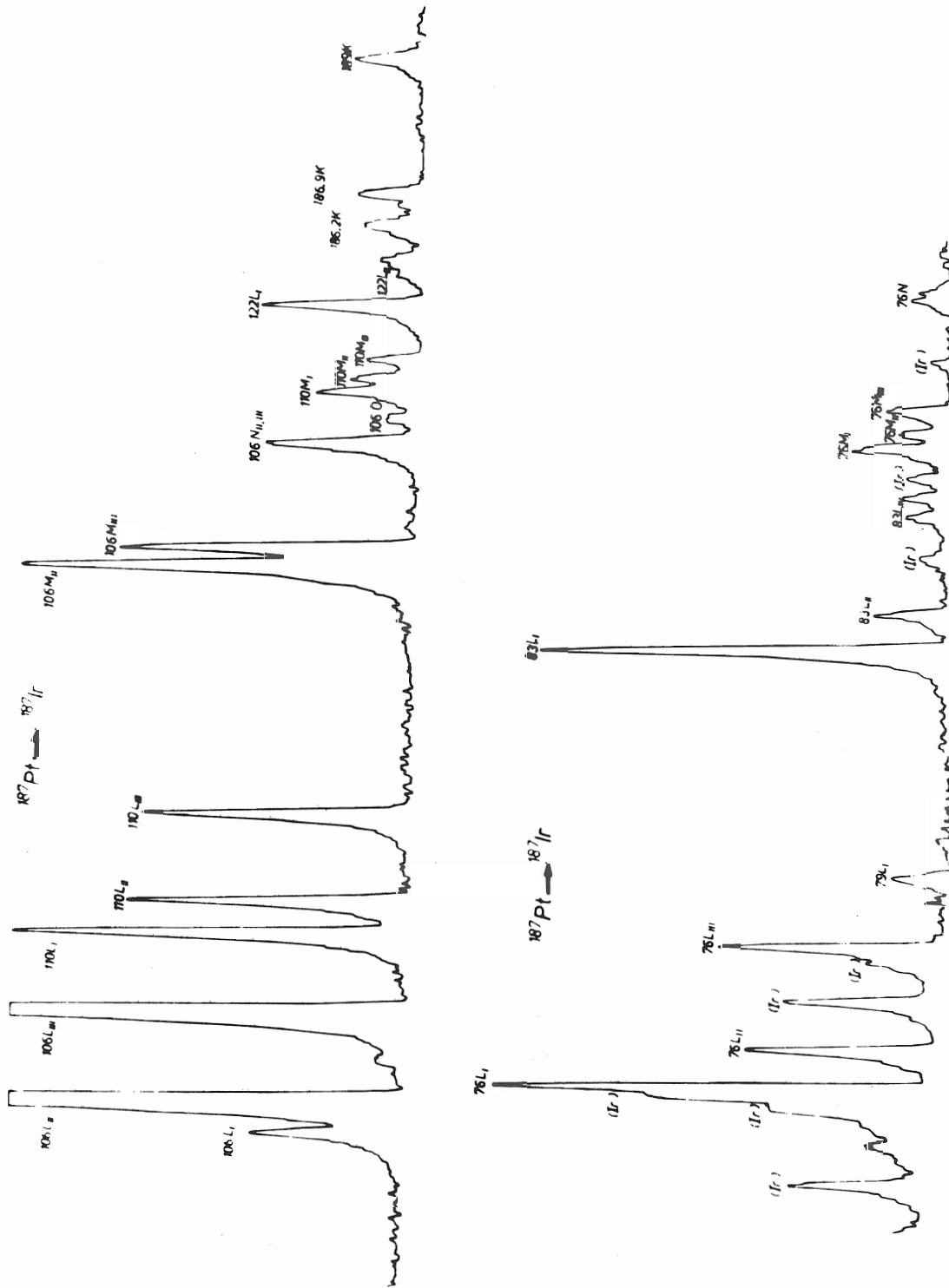
Fig. IV .4 - ^{187}\text{Pt} \rightarrow ^{187}\text{Ir} - Microdensitogrammes.
