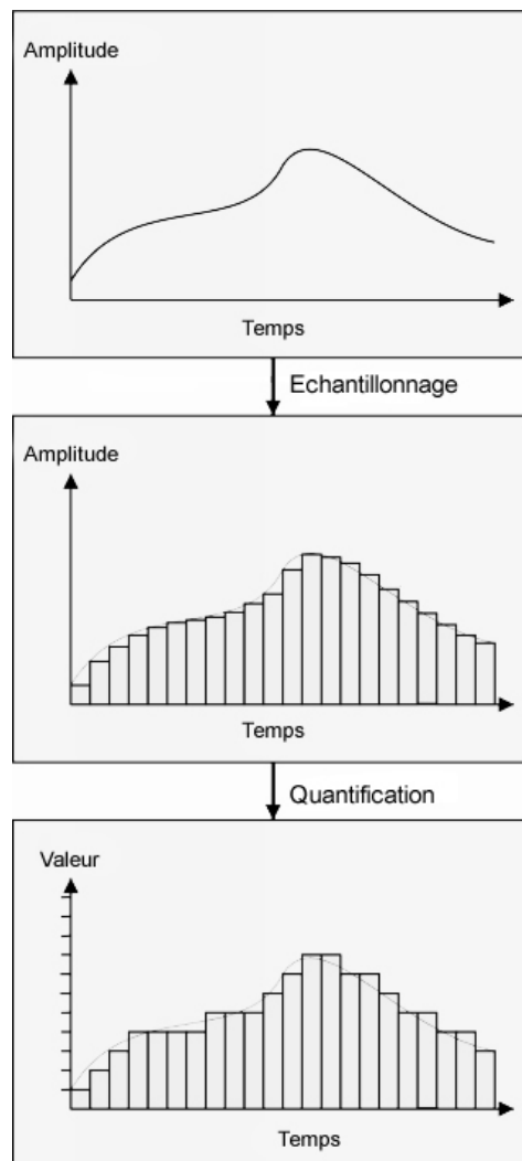
Figure 3.1. Échantillonnage et Quantification d'un signal analogique
