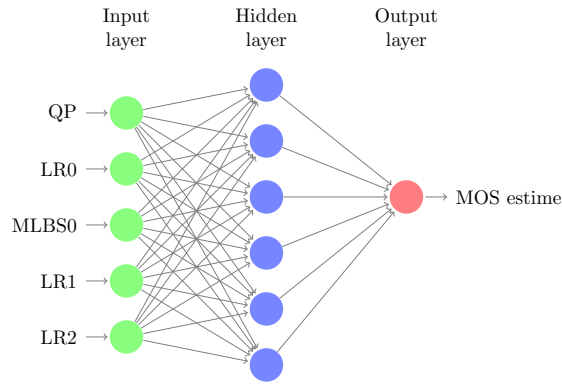
Figure 6.10. Architecture du réseau de neurones pour 3 couches
