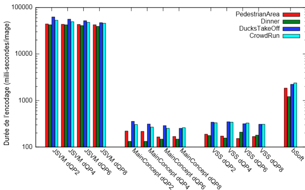
Figure 5.10. Durée de l'encodage avec différents dQP entre les couches MGS pour différents encodeurs
