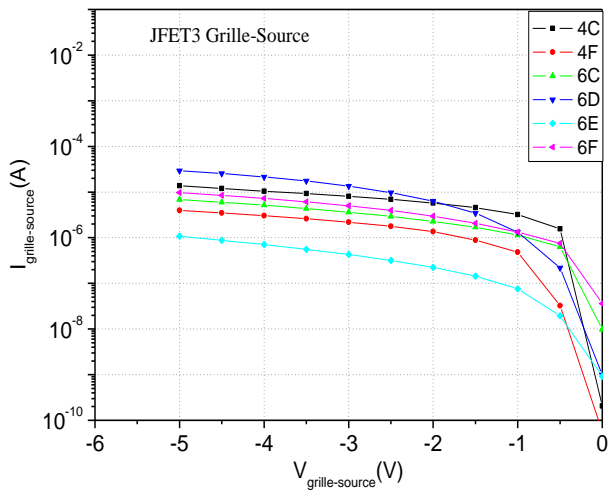
Figure 61 : Caractéristiques I_{gs}(V_{gs}) et I_{ds}(V_{ds}) des JFET 3 avec un canal de type N
