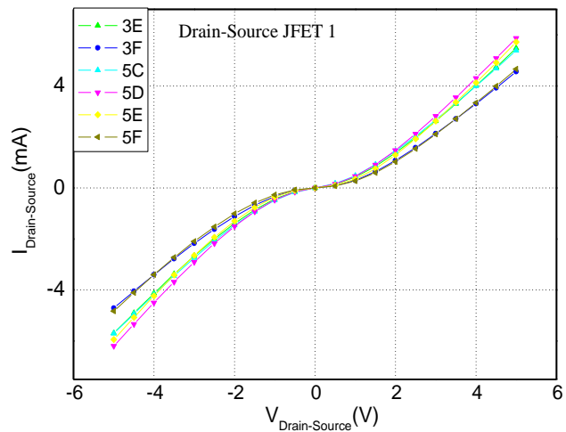
Figure 62 : Caractéristiques I_{gs}(V_{gs}) et I_{ds}(V_{ds}) des JFET 1 avec un canal de type P
