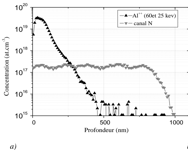
Figure 113 : a) Profil d'implantation aluminium de la grille, la source et le drain pour les caissons de type P. Ce profil a été superposé avec celui du canal N, b) tableau des énergies et les doses d'implantation.
