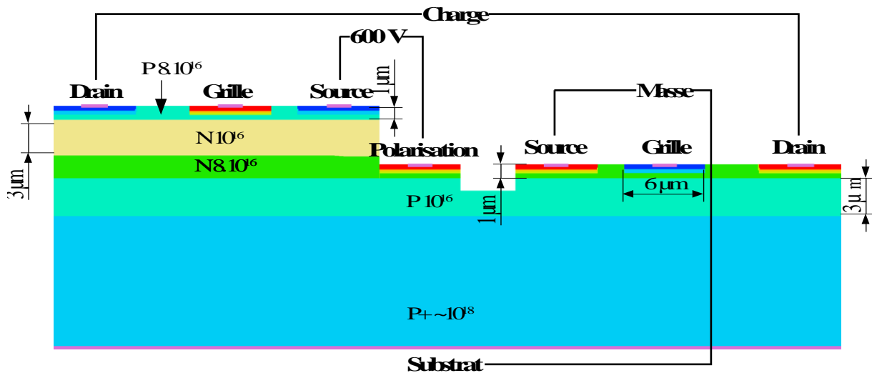
Figure 98 : Structure simulée des JFET type N et P intégrés sur le même substrat SiC pour réaliser l'étage de puissance du bras d'onduleur.
