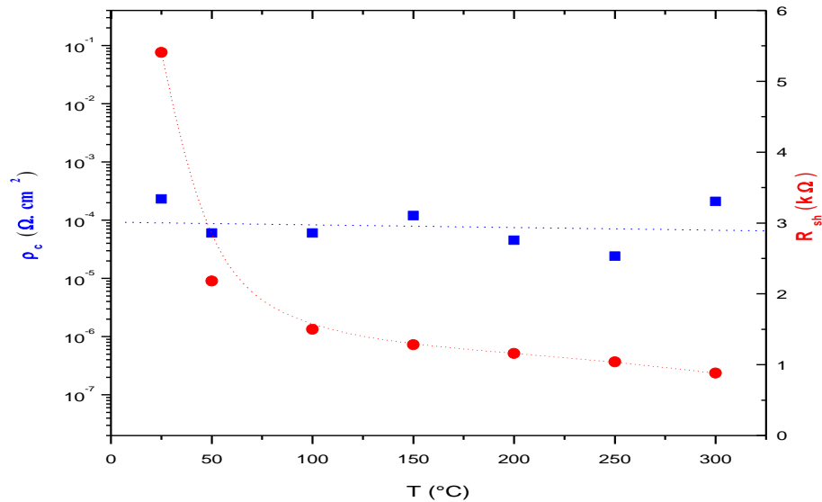
Figure 94 : Variation de la résistance spécifique de contact et la résistance carrée R_{sh} en fonction de la température de 25 à 300 °C, pour l'empilement Ni(10)/Ti(40)/Al(240)/Ni(10 nm) recuits à 800 °C sous argon.
