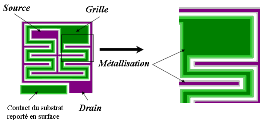
Figure 20-a: Structure en serpentín avec une grille P + métallisée sur toute sa largeur (gris pour les drain et source N + , vert clair pour la grille P + , violet et vert foncé pour la métallisation des couches).
