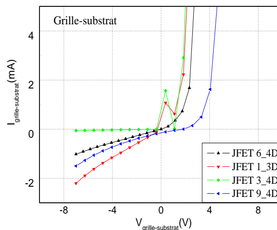
Figure 53 : Mesures I_{\text{grille-substrat}}(V)
