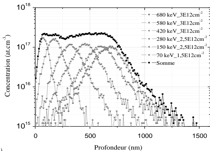
Figure 112 : a) Profil d'implantation du canal P, b) tableau des énergies et les doses d'implantation pour le canal P des JFET de la plaque II-VI EB-EC376-2 SYA.
