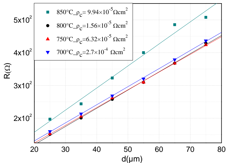
Figure 82 : La variation de la résistance entre les plots TLM et l'extraction de la résistance spécifique de contact pour les empilements Ni(10)/Ti(40)/Al(240)/Ni(10 nm) recuits à différentes températures comprises entre 700 °C et 850 °C.
