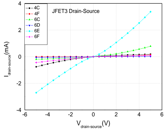
Figure 61 : Caractéristiques I_{gs}(V_{gs}) et I_{ds}(V_{ds}) des JFET 3 avec un canal de type N
