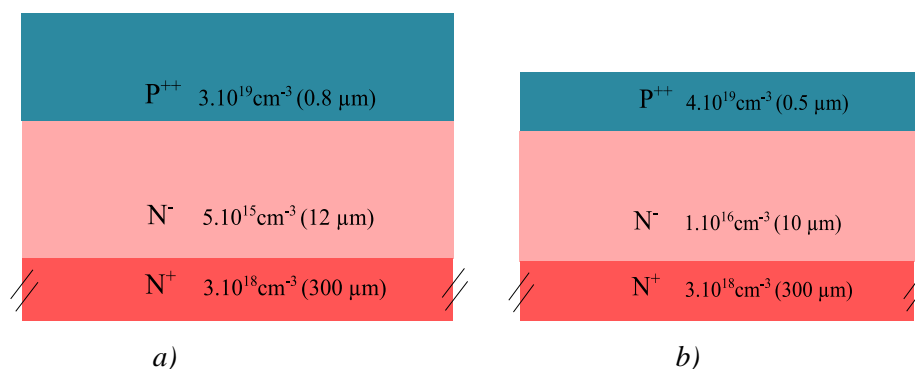
Figure 71 : Structure des échantillons avec les couches \text{P}^+ en surface : a) épitaxiées b) implantées.
