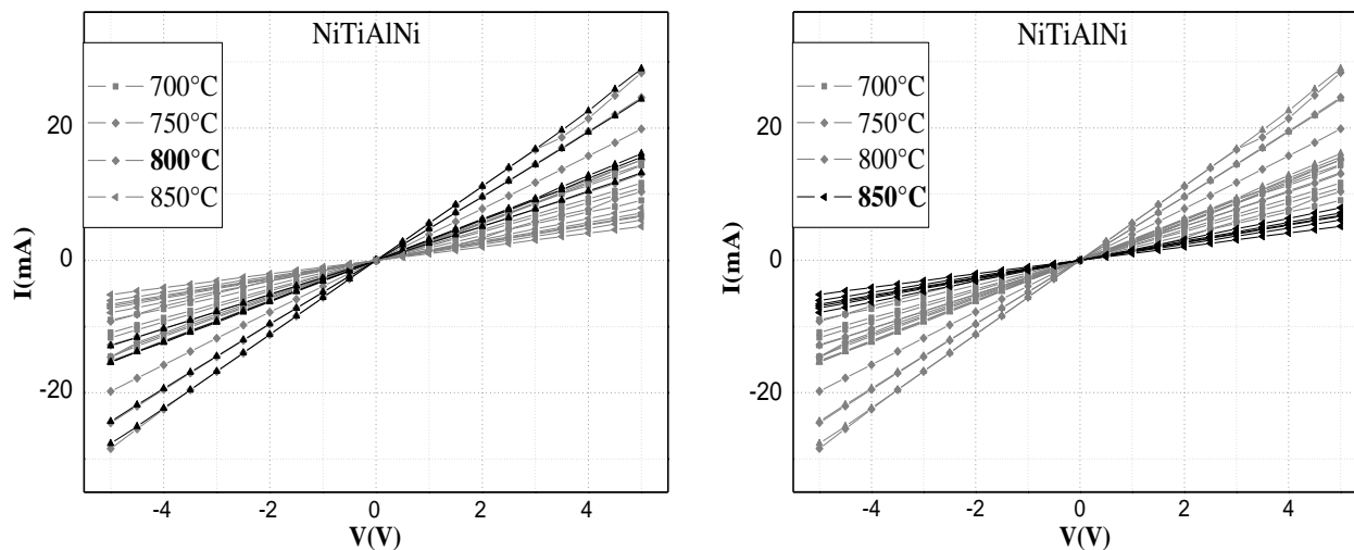
Figure 80 : Mesure I(V) des empilements Ni(10)/Ti(40)/Al(240)/Ni(10 nm), recuits de 700 °C à 850 °C sous Argon.
