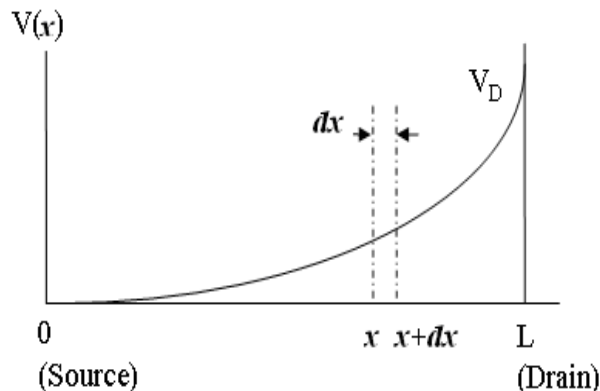
Fig 2: Variation de la tension du drain V_a tout au long du canal.
