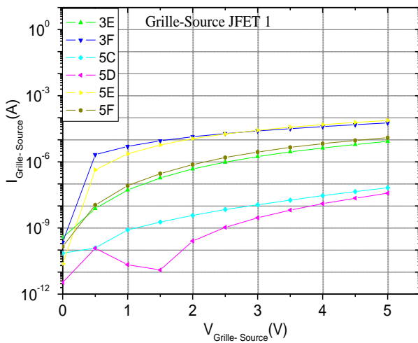
Figure 62 : Caractéristiques I_{gs}(V_{gs}) et I_{ds}(V_{ds}) des JFET 1 avec un canal de type P
