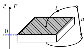
Figure 1.5 – Schéma d'une plaque piézoélectrique.
