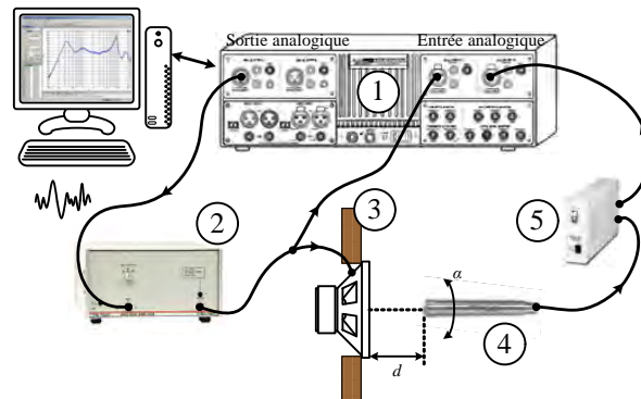
(b) Banc de caractérisation de la pression acoustique.
