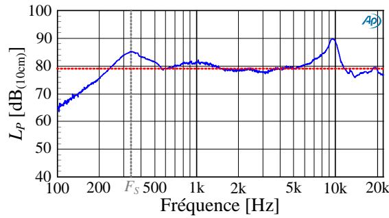
Figure 5.16 – Courbe de réponse en pression acoustique.
