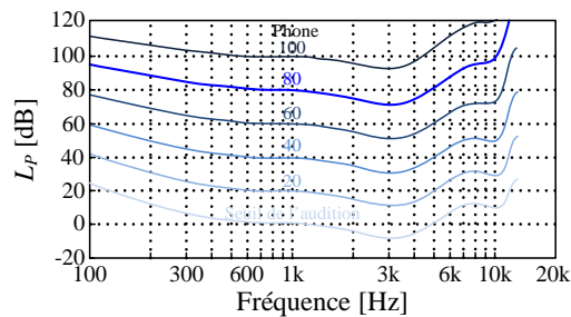
Figure 4.18 – Contours isosoniques (audition humaine).
