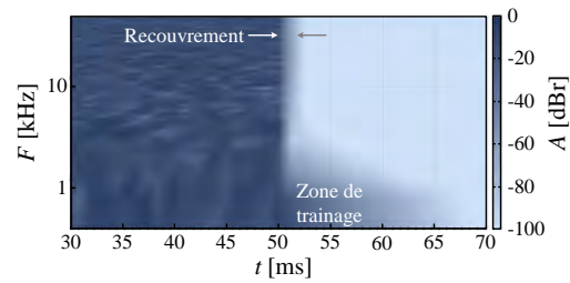
(c) Spectrogramme de l'accélération (commande en courant).
