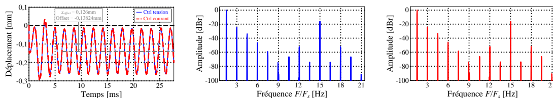
(a) x(t) pour la commande en tension et courant. (b) IMD, commande en tension (tout non-linéaire). (c) IMD, commande en courant (tout non-linéaire).
