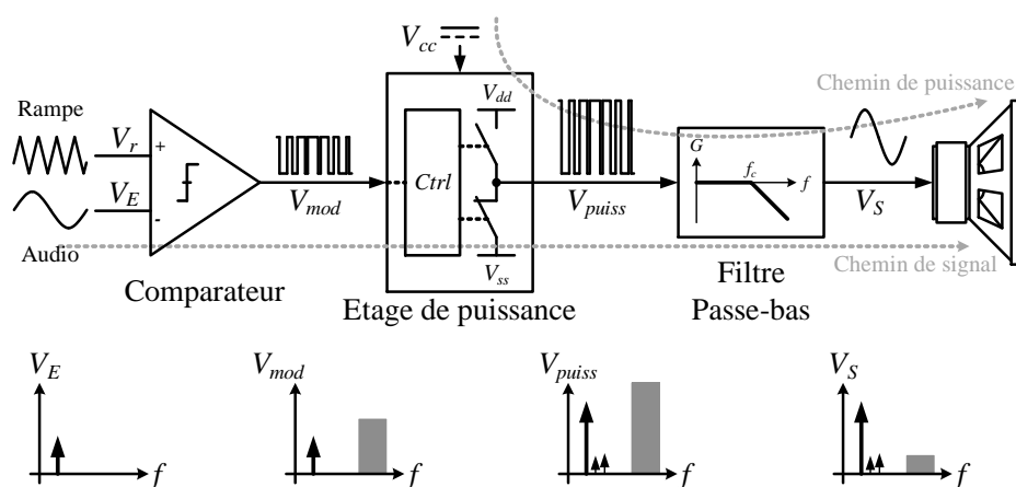
Figure 1.20 – Schéma de principe du Classe-D analogique.
