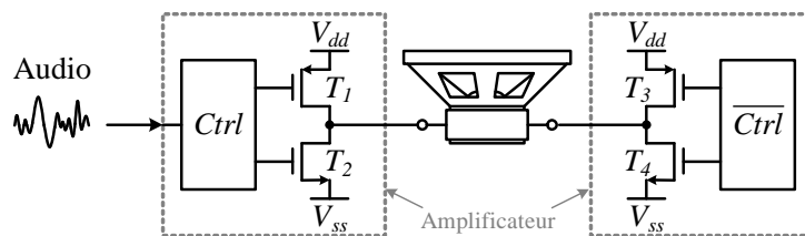
Figure 1.15 – Schéma d'une configuration pont en H.
