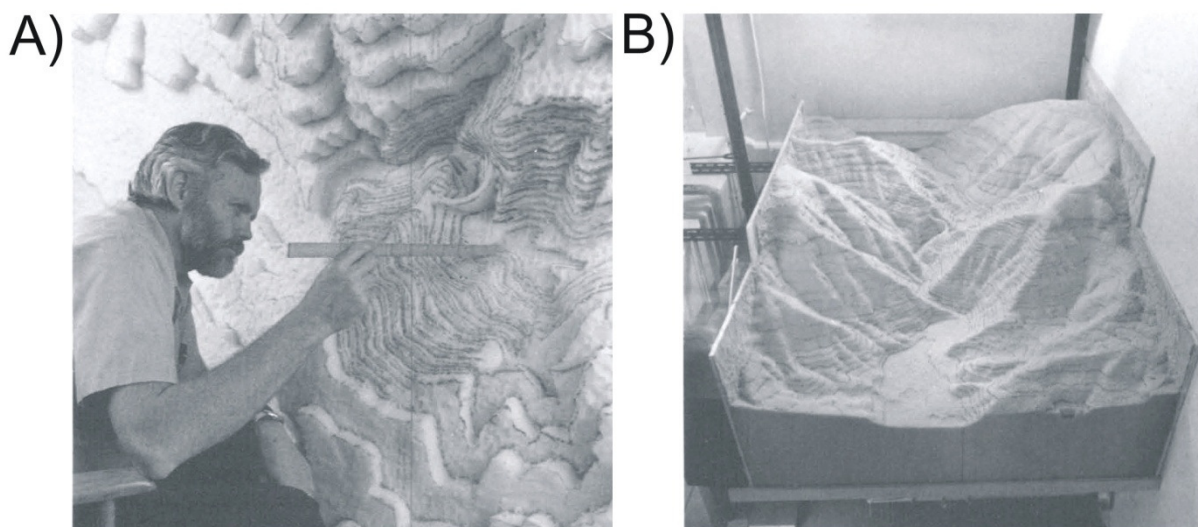
Figure 1-28 : Construction d'un modèle 3D analogique de topographie réaliste (A), représentant le relief autour du barrage de Pacoima en Californie (B) [d'après Anooshehpoor & Brune, 1989]. Le barrage est figuré au centre du modèle.
