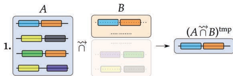
(a) Le calcul de A \tilde{\cap} B sans découpage de l'index conduit à deux faux positifs de séquence.
