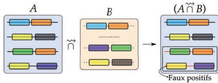
(a) Le calcul de A \tilde{\cap} B sans découpage de l'index conduit à deux faux positifs de séquence.
