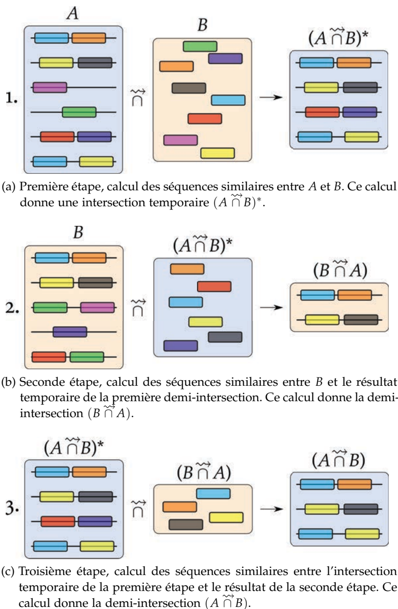
FIGURE 18: Le pipeline complet de la méthode permet le calcul de (A \overset{\rightsquigarrow}{\cap} B) et (B \overset{\rightsquigarrow}{\cap} A) en suivant les trois étapes décrites dans cette figure. On voit que la dernière étape permet d'enlever un faux positif de séquence présent dans (A \overset{\rightsquigarrow}{\cap} B)^* . La résolution de ce cas de faux positif est expliqué en détail figure 20.
