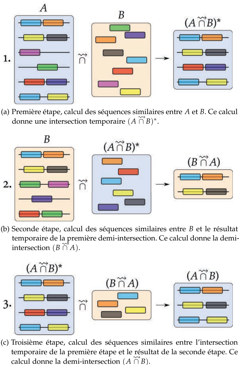
FIGURE 18: Le pipeline complet de la méthode permet le calcul de (A \overset{\rightsquigarrow}{\cap} B) et (B \overset{\rightsquigarrow}{\cap} A) en suivant les trois étapes décrites dans cette figure. On voit que la dernière étape permet d'enlever un faux positif de séquence présent dans (A \overset{\rightsquigarrow}{\cap} B)^* . La résolution de ce cas de faux positif est expliqué en détail figure 20.
