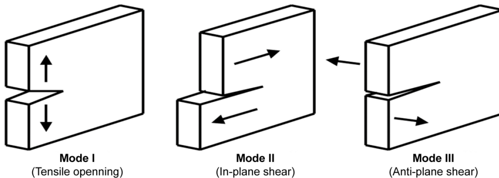
Figure 15: Les trois modes de rupture d'une fracture. Mode I - ouverture normale aux épontes; Mode II - glissement dans la direction du plan de cisaillement; Mode III - glissement dans la direction perpendiculaire à la linéation de cisaillement. [Mach et al., 2007].
