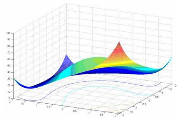
(c) Fonction Perm à 2 variables
