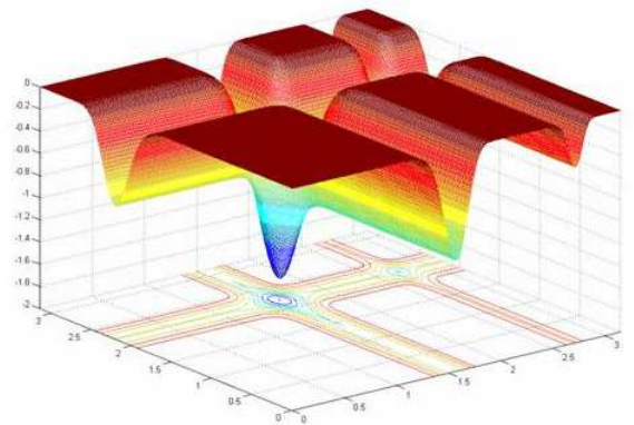
(b) Fonction Michalewicz à 2 variables
