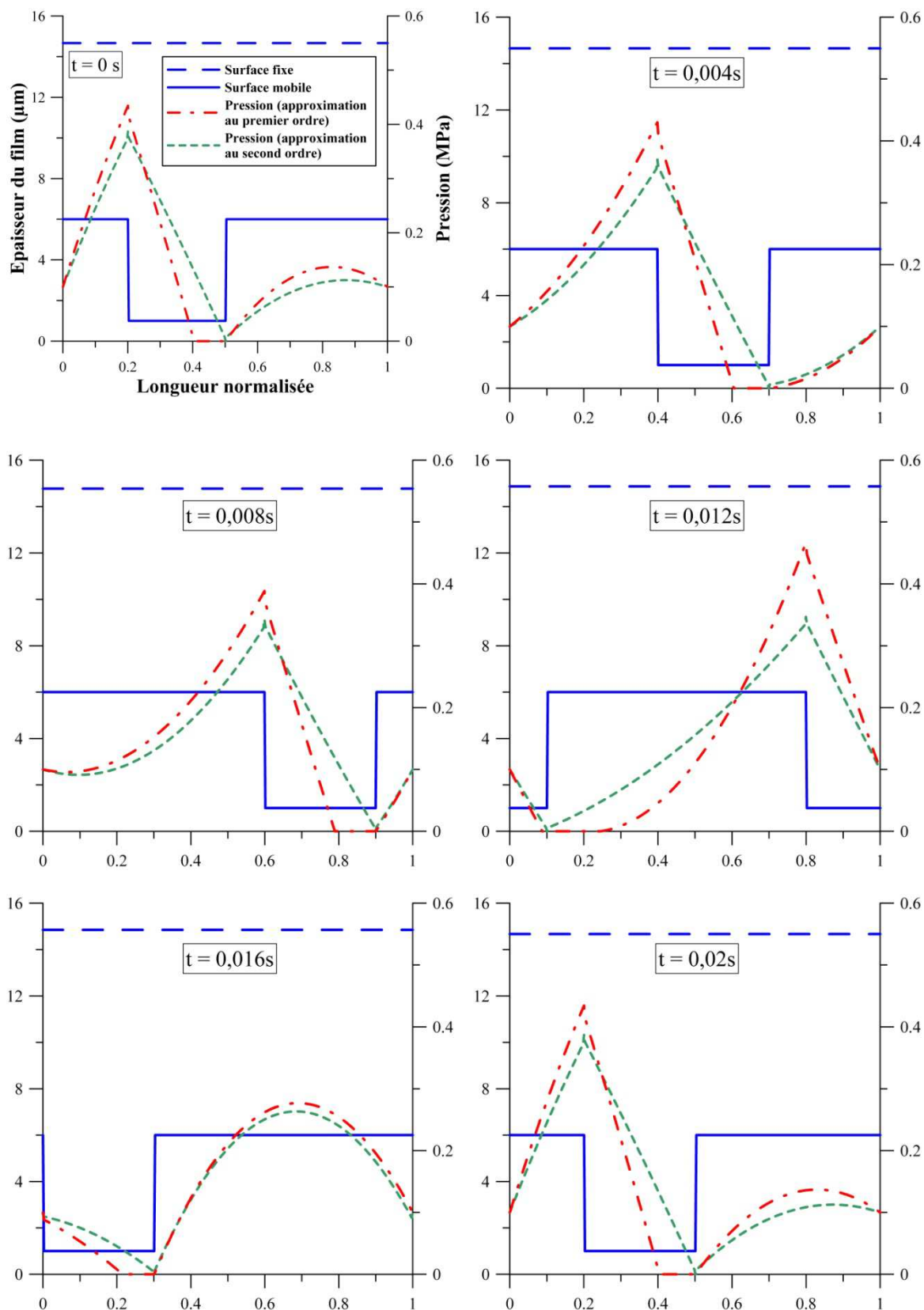
Figure 2.43. Evolution de la géométrie du patin et de la distribution de pression à travers une période T_t = 0,02 \text{ s} ( U = 1 \text{ m/s} et W_a = 1 \text{ N/mm} ).
