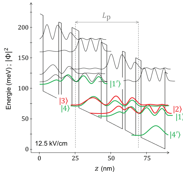
FIGURE 5.1 – Diagramme de bande de la période élémentaire d'une région active à trois puits quantiques de type phonon-résonant au champ d'alignement (12.5 kV/cm). La séquence est issue de la référence [93].
