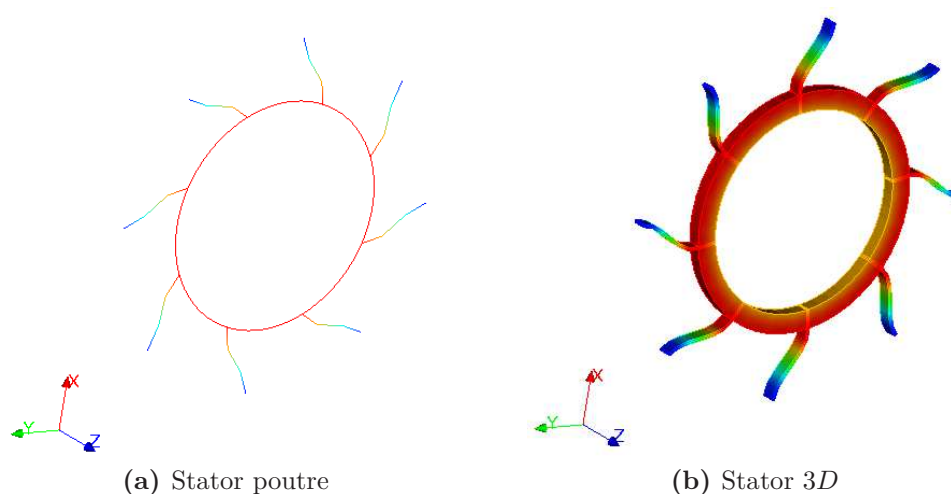
Figure 3.32.: Premier mode propre du stator
