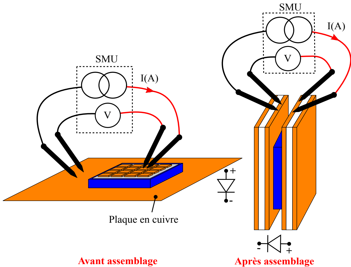
Figure 3.18 Circuit de mesure pour la caractérisation électrique des diodes avant et après l'assemblage
