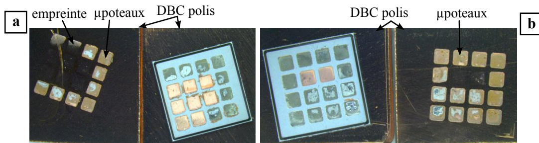
Figure 3.21 Photos des échantillons assemblés par le four RTA après le test de cisaillement avec les DBC polis
