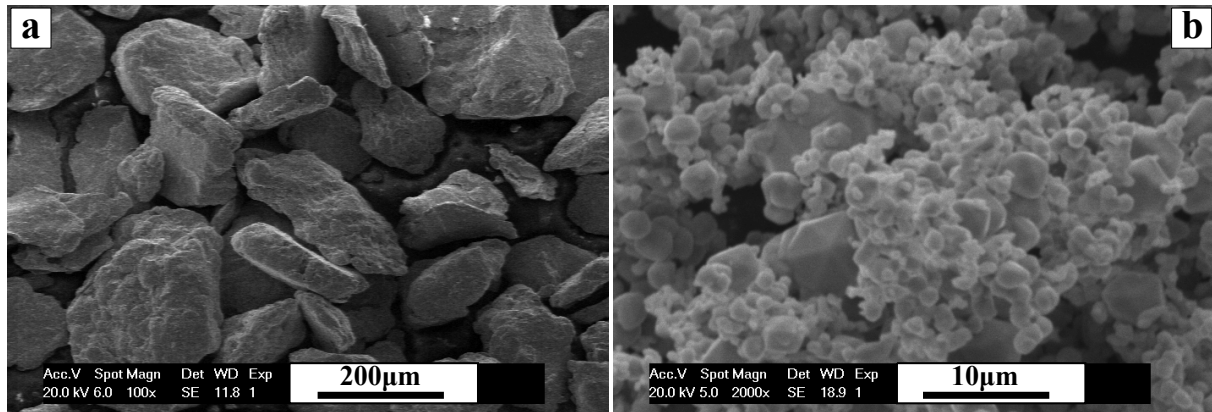
Figure 4.2 Photo MEB de la poudre de molybdène avec la taille de particule (a) 55 à 355 \mu\text{m} et (b) 2 \mu\text{m}
