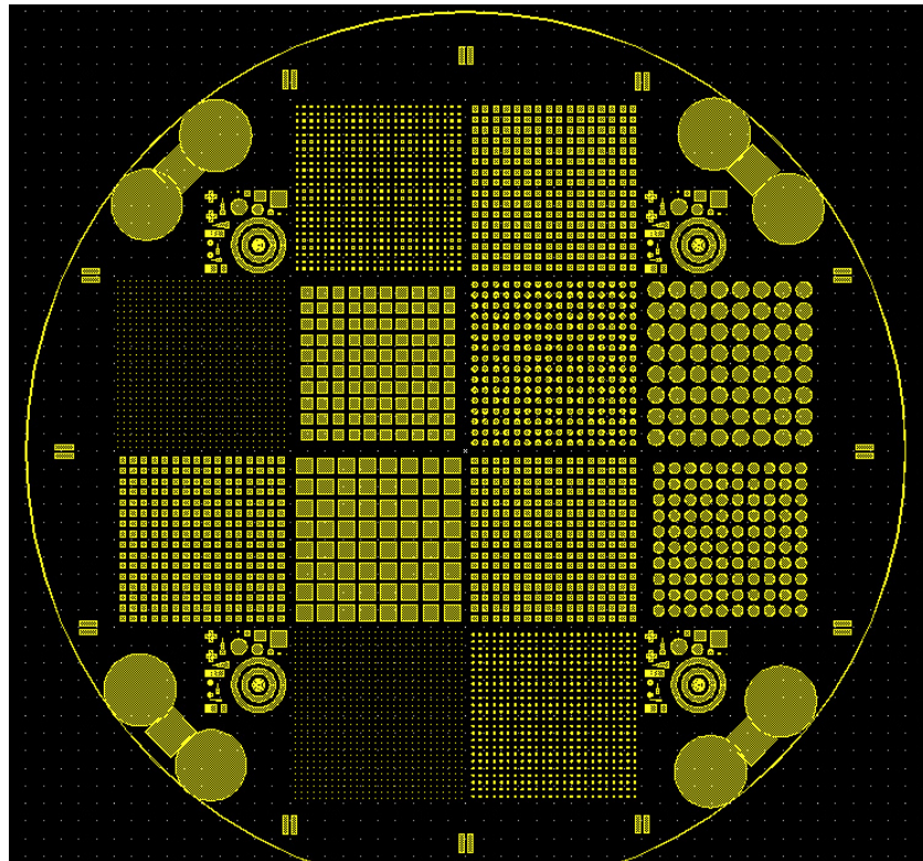
Figure 3.2 Photo du masque de test contenant des motifs carré et cercle de différents dimensions : 50, 100, 300, 600 et 900 \mu\text{m} . Ce masque a servi aux essais préliminaires effectués sur des wafers de silicium bruts de deux pouces de diamètre.
