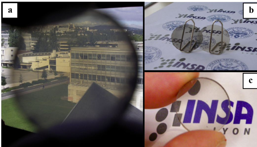
Figure 1.22 Photos montrant l'aspect transparent des céramiques frittées au SPS (a) \alpha\text{-Al}_2\text{O}_3 polycristallin [Lallemant et al. 2012], (b) YAG [Spina et al. 2012] et (c) \text{MgAl}_2\text{O}_4 spinelle [Bonfont et al. 2012]
