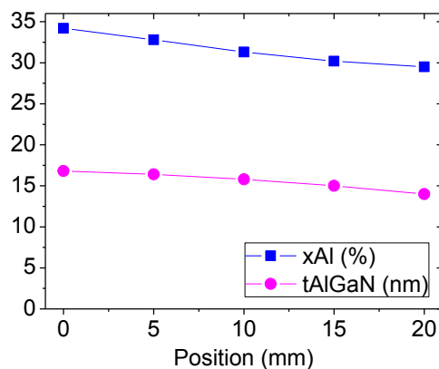
Figure III.3-5 : Gradient en épaisseur et en teneur en aluminium dans la barrière AlGaN, estimé par DRX sur l'échantillon D382.
