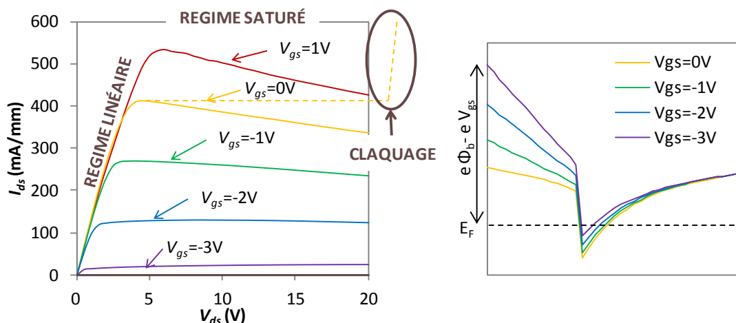
Figure I.5-2 : Réseau de caractéristiques de sortie I_{ds}(V_{ds}, V_{gs}) d'un transistor HEMT AlGaIn/GaN à droite, et modèle de bande du transistor polarisé à gauche.
