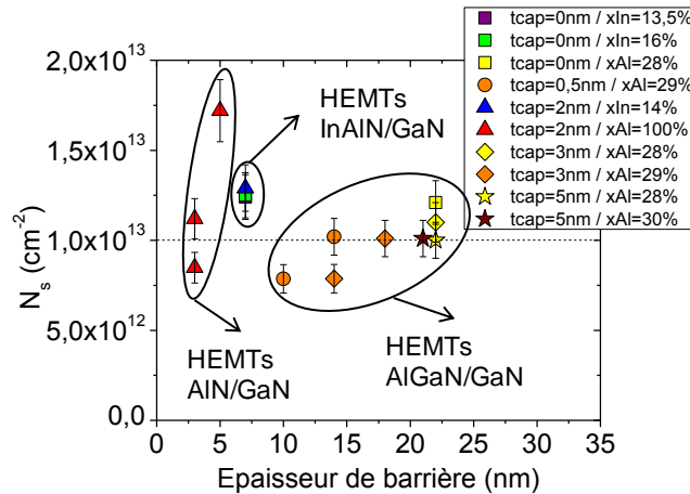
Figure II.3-3 : Densité d'électrons du gaz 2D mesuré par C-V des hétérostructures HEMTs AlGaIn/GaN, AlN/GaN et InAlN/GaN. La forme des symboles est associée à une épaisseur de cap, et la couleur de remplissage des symboles correspond à la teneur en aluminium ou en indium de la barrière. Le trait pointillé correspond à la valeur de N_s minimale recherchée.
