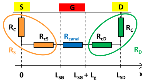
Figure I.5-3 : Représentation schématique des résistances en série présentes dans la structure HEMT. R_c est la résistance des contacts Ohmiques, R_{cS} et R_{cD} correspondent aux résistances du canal côté source et drain respectivement.
