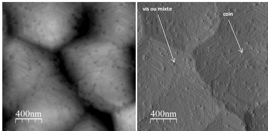
Figure I.4-7 : Scan AFM de 2\,\mu\text{m} \times 2\,\mu\text{m} d'une structure HEMT AlGaIn/GaN épitaxiée par EJM-NH 3 . A gauche l'image est en mode topographique et à droite, l'image est en mode dérivé.
