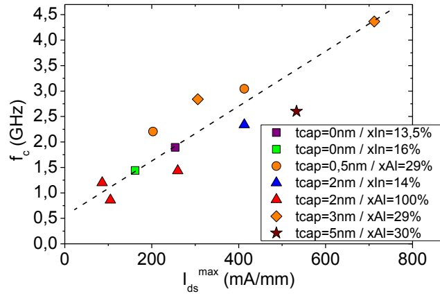
Figure II.5-4 : Fréquence de coupure intrinsèque des transistors avec L_g = 2-3 \mu\text{m} en fonction du maximum de densité de courant I_{ds} .
