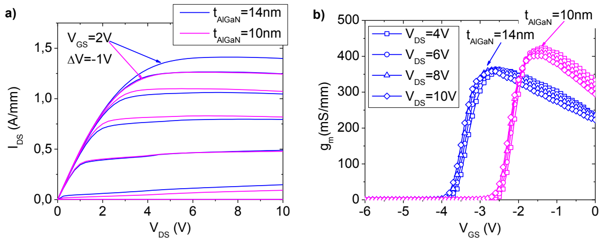
Figure IV.3-1 : Caractéristique de sortie (a) et transconductance (b) des structures fines AlGaN/GaN mesuré sur un transistor ayant pour dimension 2 \times 50 \mu\text{m} \times 0,25 \mu\text{m} . L'espaceur source drain est de 1,5 \mu\text{m} , et L_{sg} = 400 \text{ nm} .
