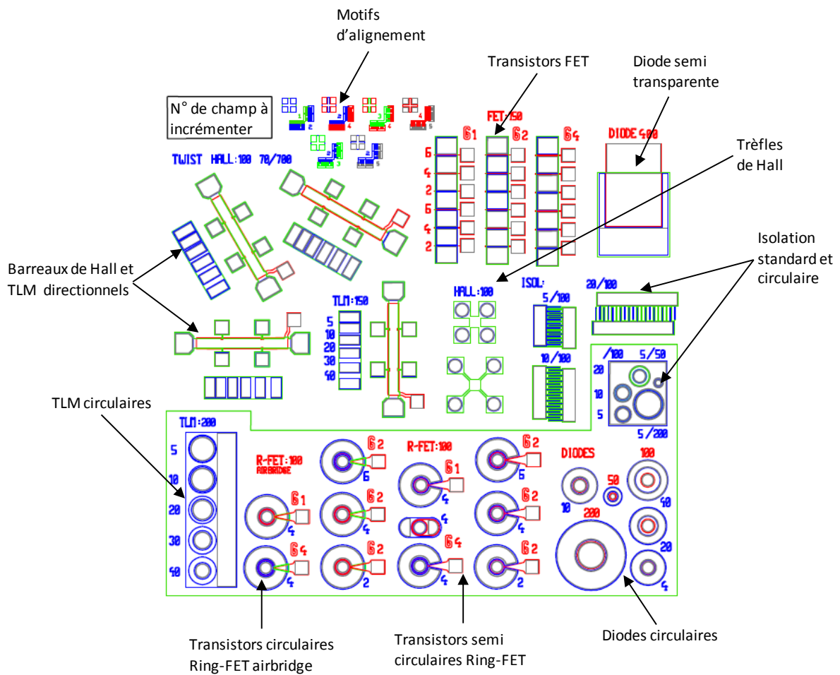
Figure I.4-12 : Champ ( 3700 \mu\text{m} \times 3600 \mu\text{m} ) du masque utilisé pour réaliser des composants test sur les échantillons épitaxiés. Chaque couleur correspond à un niveau de masque : mésas (vert foncé), ohmique (bleu), résine air bridge (vert clair), grille (rouge), épaisseur (gris).
