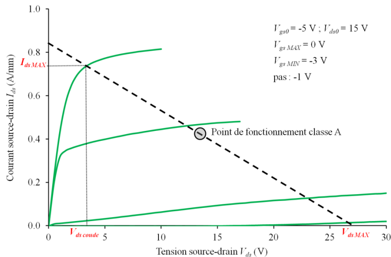
Figure I.5-6 : Caractéristique pulsée avec le point de polarisation ( V_{gs0} = -5\text{V} ; V_{ds0} = 15\text{V} ) et droite de charge optimale dans le but d'obtenir le maximum de puissance en sortie d'un transistor fonctionnant en classe A.
