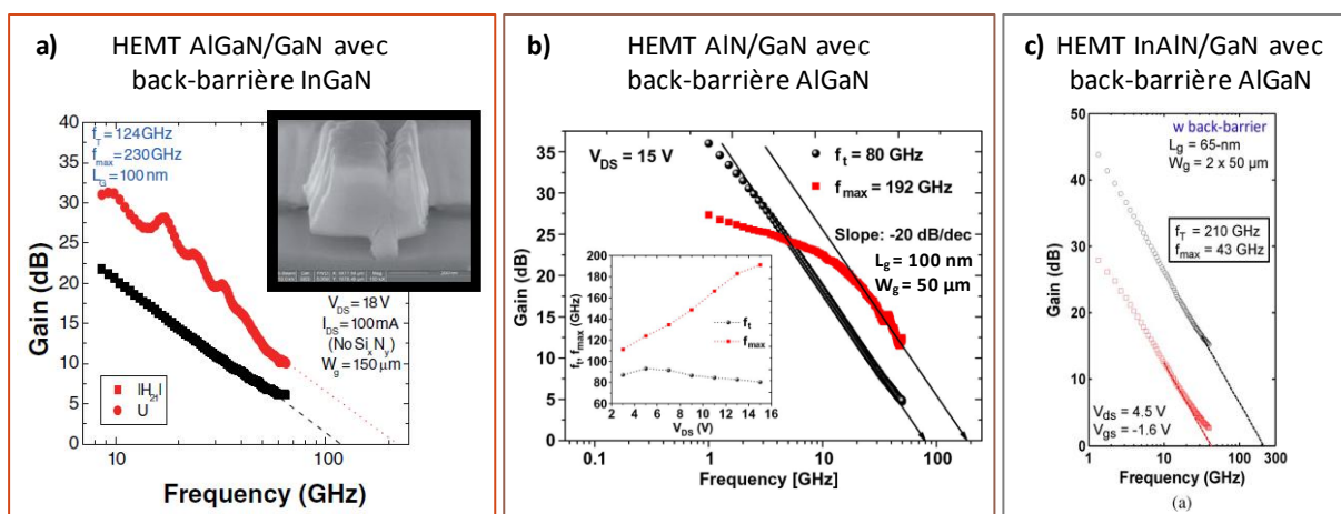
Figure III.1-3 : Performances en fréquence de transistors de différentes barrières ayant une barrière de confinement a) InGaIn [5] ou b) et c) AlGaIn ([7] et [6] respectivement).
