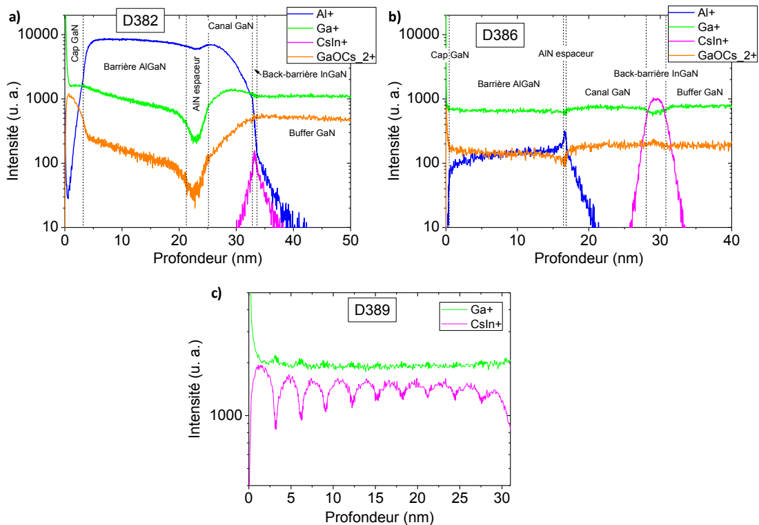
Figure III.3-11 : Profil en profondeur des structures HEMTs à barrière de confinement \text{InGaN} (a et b) et d'un super réseau \text{InGaN/GaN} (c).
