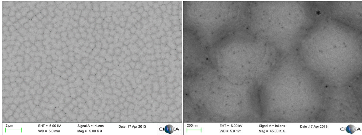
Figure I.4-6 : Image MEB d'une structure HEMT AlGaIn/GaN : morphologie en colline, caractéristique de la croissance de GaN en MBE-NH 3 . A droite, à un grandissement \times 45\,000 : les dislocations sont discernables.
