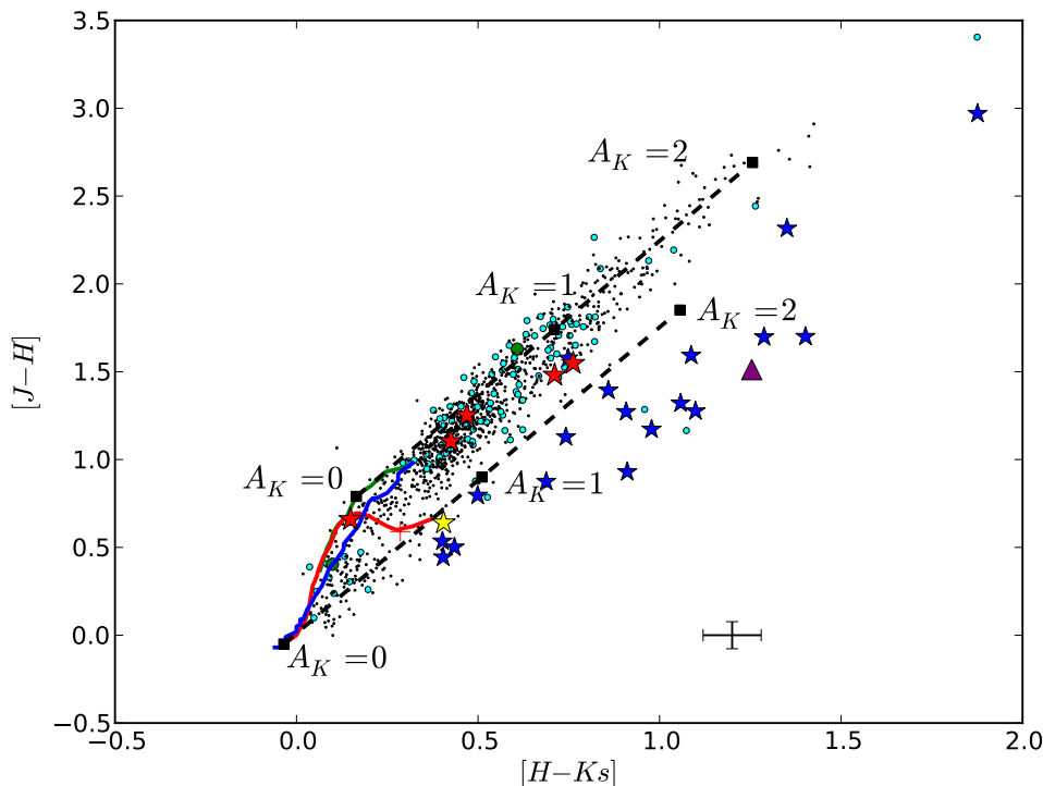
FIGURE 12.18 – Diagramme représentant la couleur [J-H] en fonction de la couleur [H-K_s] pour les sources ponctuelles situées dans la région de 10' \times 10' autour de GX 301-2. Les symboles utilisés sont identiques à ceux utilisés en figure 12.13. Les couleurs corrigées de l'extinction, des étoiles naines, géantes et supergéantes, sont représentées respectivement par les courbes rouges, vertes et bleues et données par Bessell and Brett (1988) et Koornneef (1983). L'étoile jaune correspond à GX 301-2. L'extinction en bande K_s , A_K , est matérialisée par les traits en tirets pour des valeurs comprises entre 0 et 2 magnitudes. Les barres d'erreurs ont été évaluées à partir de la médiane des erreurs sur les couleurs.
