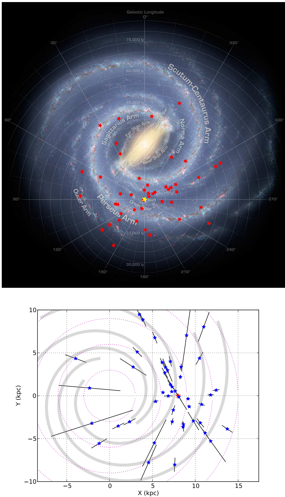
FIGURE 5.6 – Figure du haut : représentation de la distribution des HMXBs (étoiles rouges) dans la Voie Lactée. La position du Soleil aux coordonnées (0 , 8.5 kpc) à partir du centre galactique, est définie par l'étoile jaune. Illustration de la Voie Lactée empruntée à NASA/Adler/U. Chicago/Wesleyan/JPL-Caltech . Figure du bas : position des HMXBs (représentées par les étoiles bleues) avec les barres d'erreur (zoom au voisinage du Soleil, représenté par l'étoile rouge et situé à 8.5 kpc du centre Galactique). Les bras spiraux, représentés par les courbes grises sont issus du modèle de Russeil (2003).
