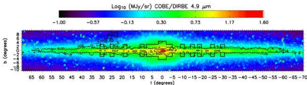
FIGURE 4.3 – Région du ciel couverte par les trois relevés GLIMPSE superposée à une image du plan Galactique obtenue avec l'instrument COBE/DIRBE à 4.9 \mu\text{m} . Les lignes en pointillés représentent les zones couvertes par GLIMPSE I et II. Les extensions en latitude représentent la couverture de GLIMPSE 3D. Figure extraite de Churchwell et al. (2009).
