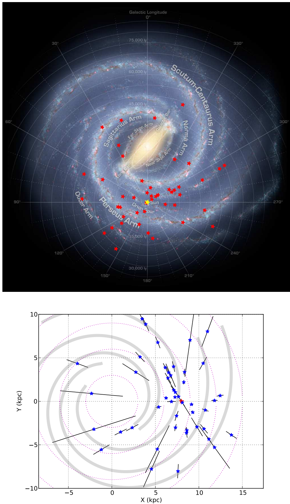
FIGURE 5.6 – Figure du haut : représentation de la distribution des HMXBs (étoiles rouges) dans la Voie Lactée. La position du Soleil aux coordonnées (0, 8.5 \text{ kpc}) à partir du centre galactique, est définie par l'étoile jaune. Illustration de la Voie Lactée empruntée à NASA/Adler/U. Chicago/Wesleyan/JPL-Caltech . Figure du bas : position des HMXBs (représentées par les étoiles bleues) avec les barres d'erreur (zoom au voisinage du Soleil, représenté par l'étoile rouge et situé à 8.5 \text{ kpc} du centre Galactique). Les bras spiraux, représentés par les courbes grises sont issus du modèle de Russeil (2003).
