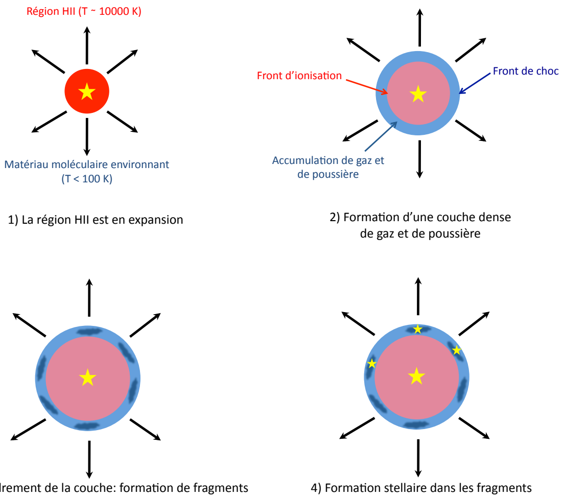
FIGURE 12.15 – Schéma explicatif du mécanisme « d'accumulation et d'effondrement » conduisant à la formation de nouvelles étoiles par expansion d'une région HII entourant une étoile massive.
