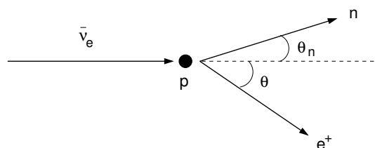
FIGURE 4.4 – Schéma de la réaction \beta inverse.
