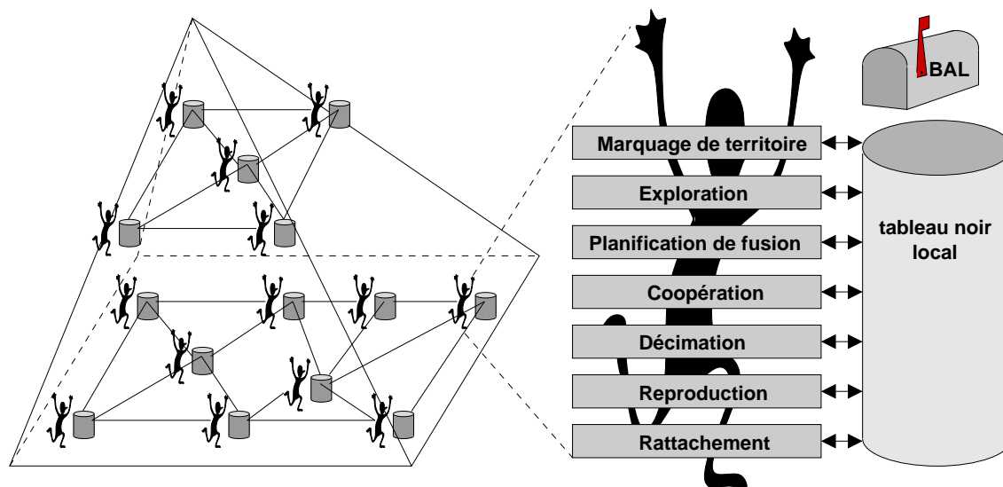
FIG. 9.1 : Un agent de la pyramide ( PrimitivAgt ) et ses sept comportements.
